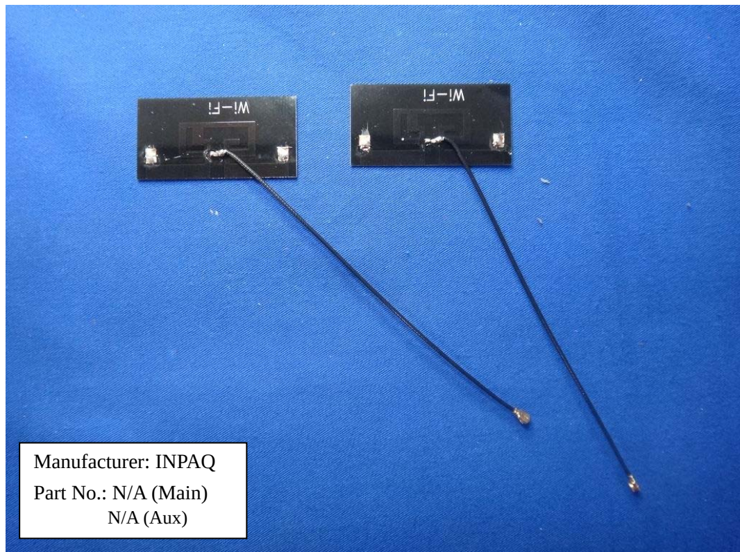
(8) EUT Photo
