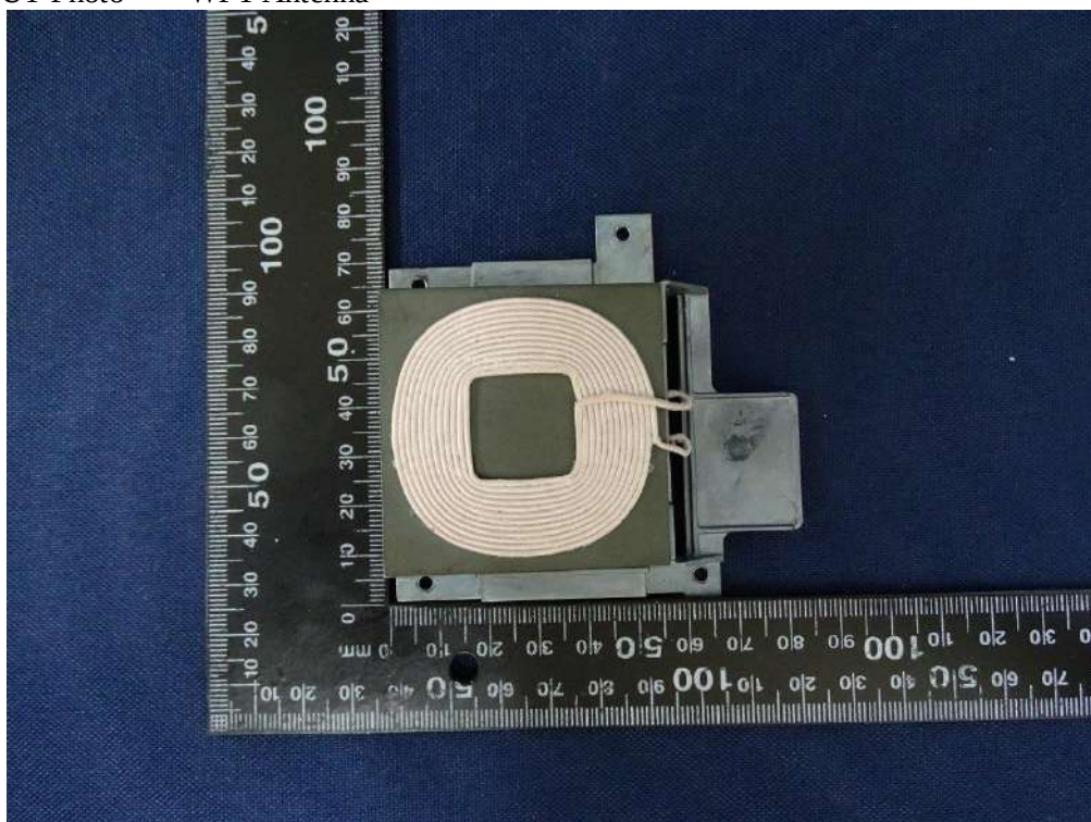
(24) EUT Photo WPT Antenna
