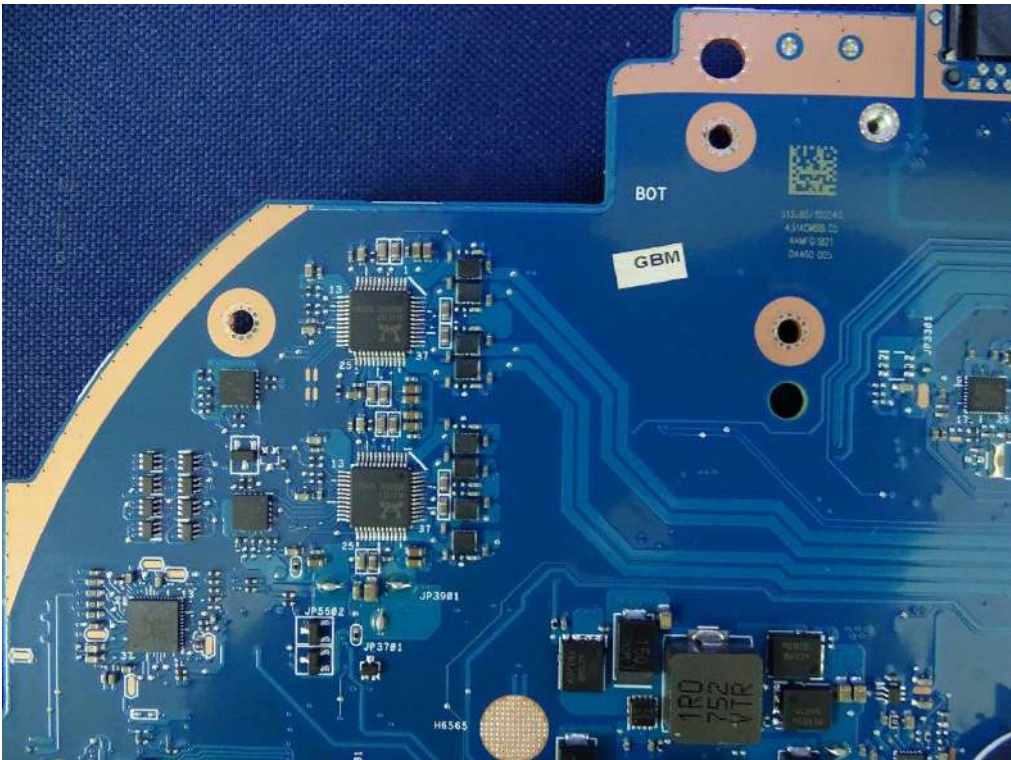
(46) EUT Photo
