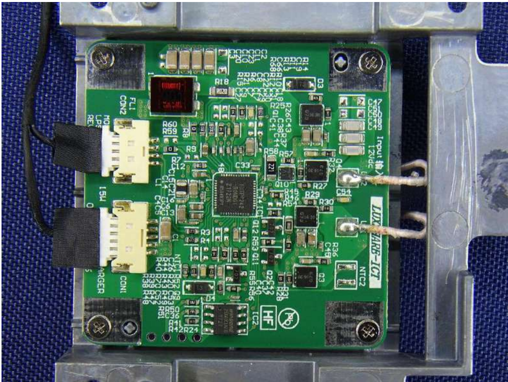
(28) EUT Photo WPT Module
