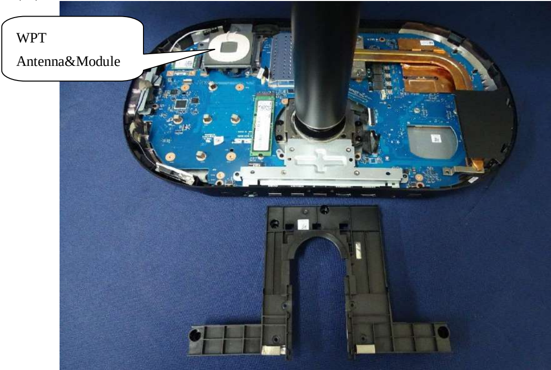
(10) EUT Photo
