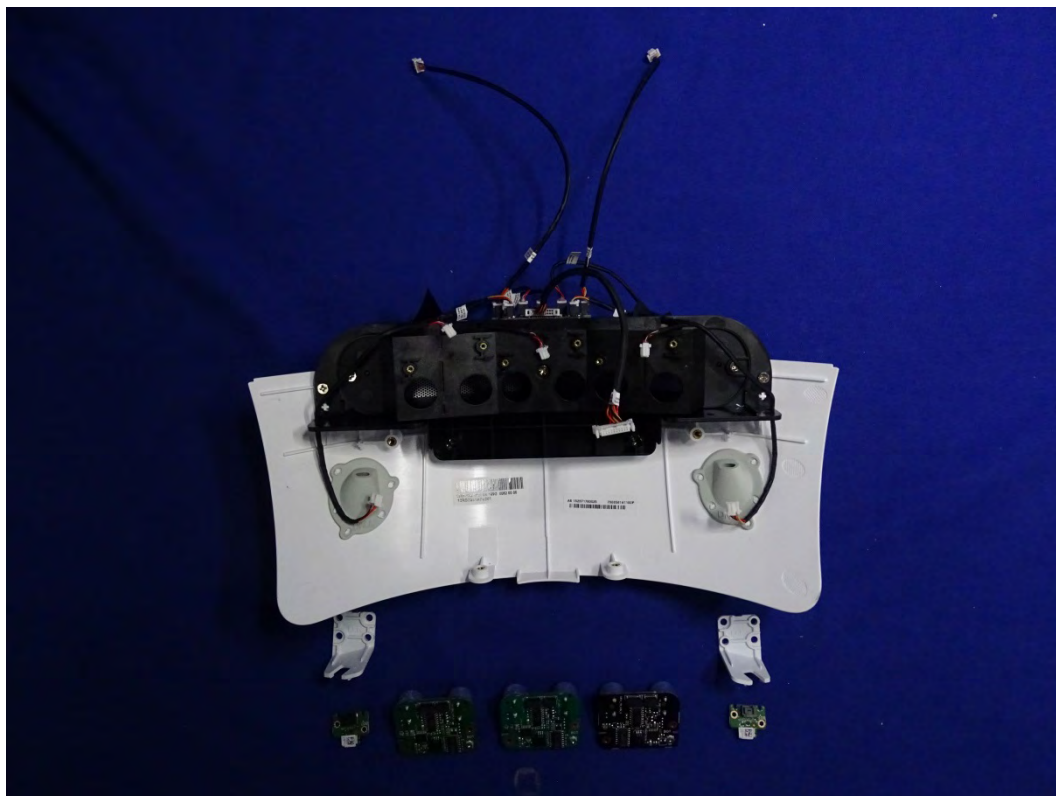
(69) EUT Photo
