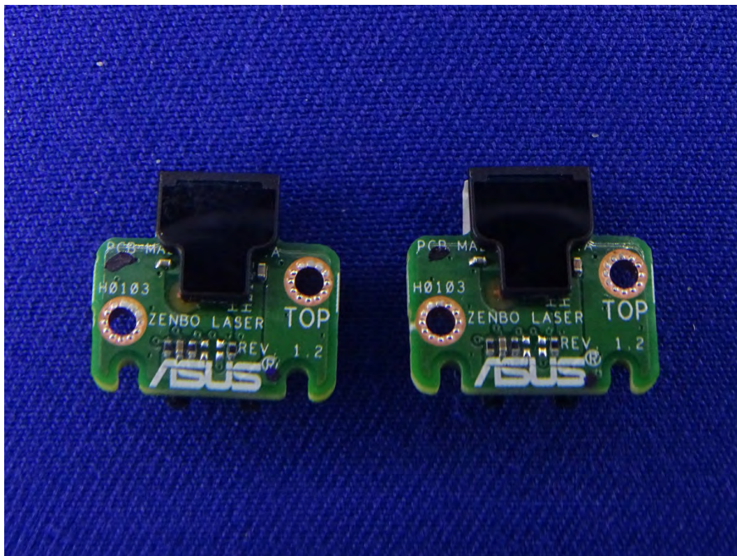
(77) EUT Photo
