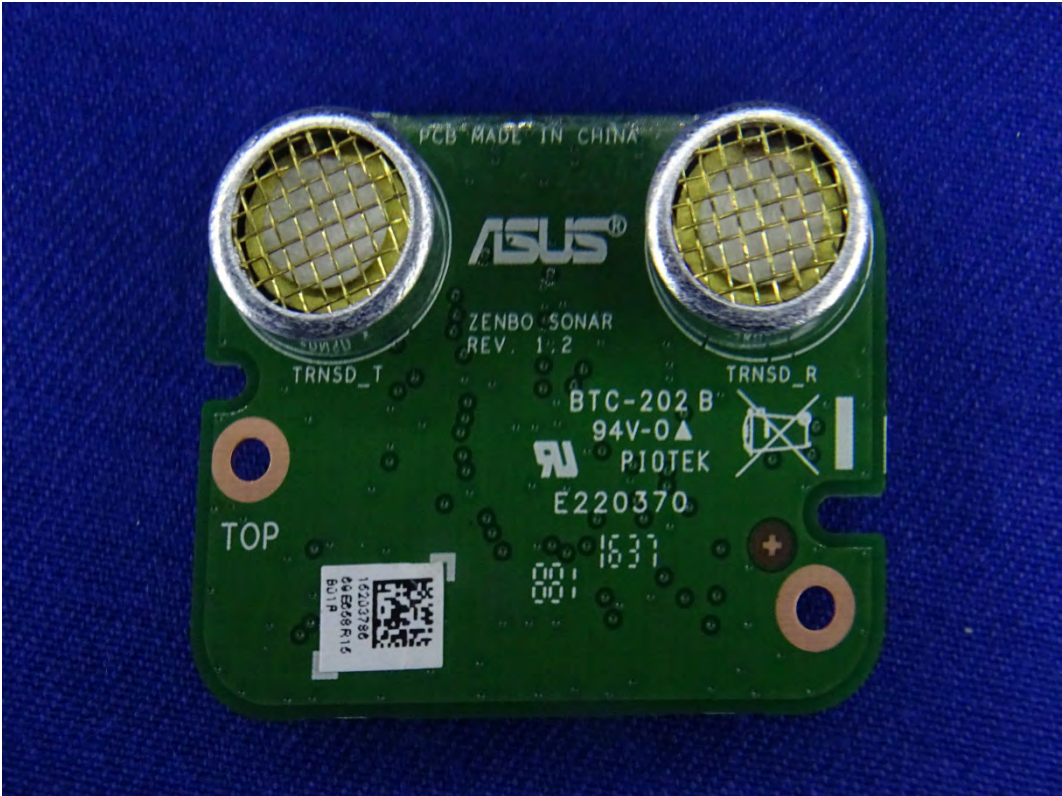
(75) EUT Photo
