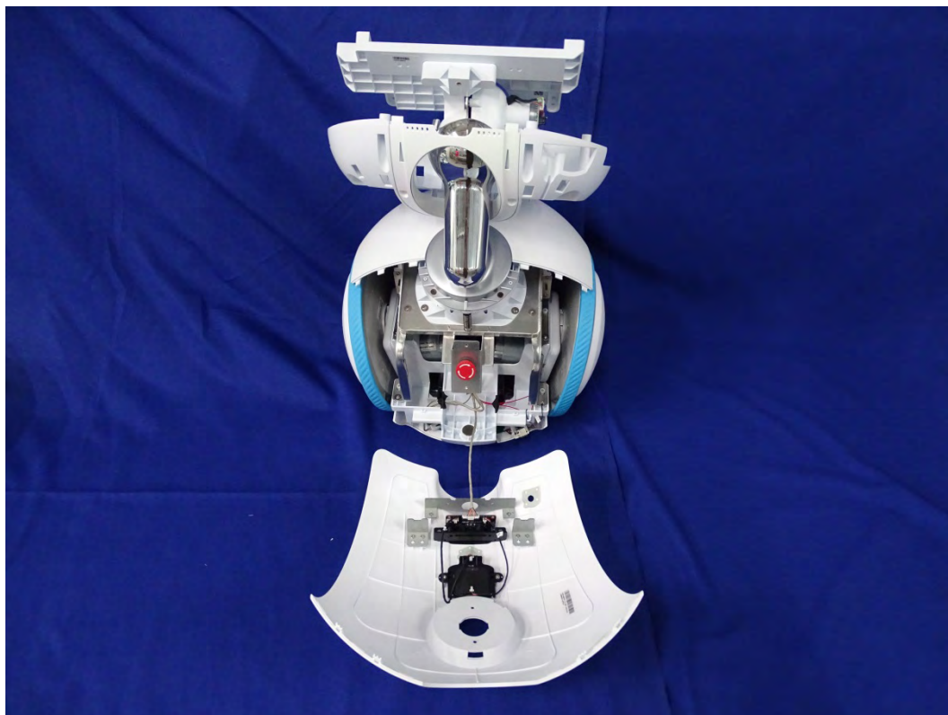
(53) EUT Photo
