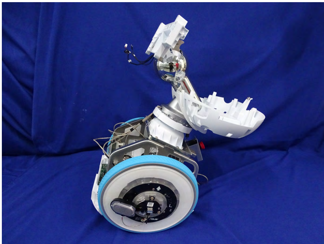
(83) EUT Photo
