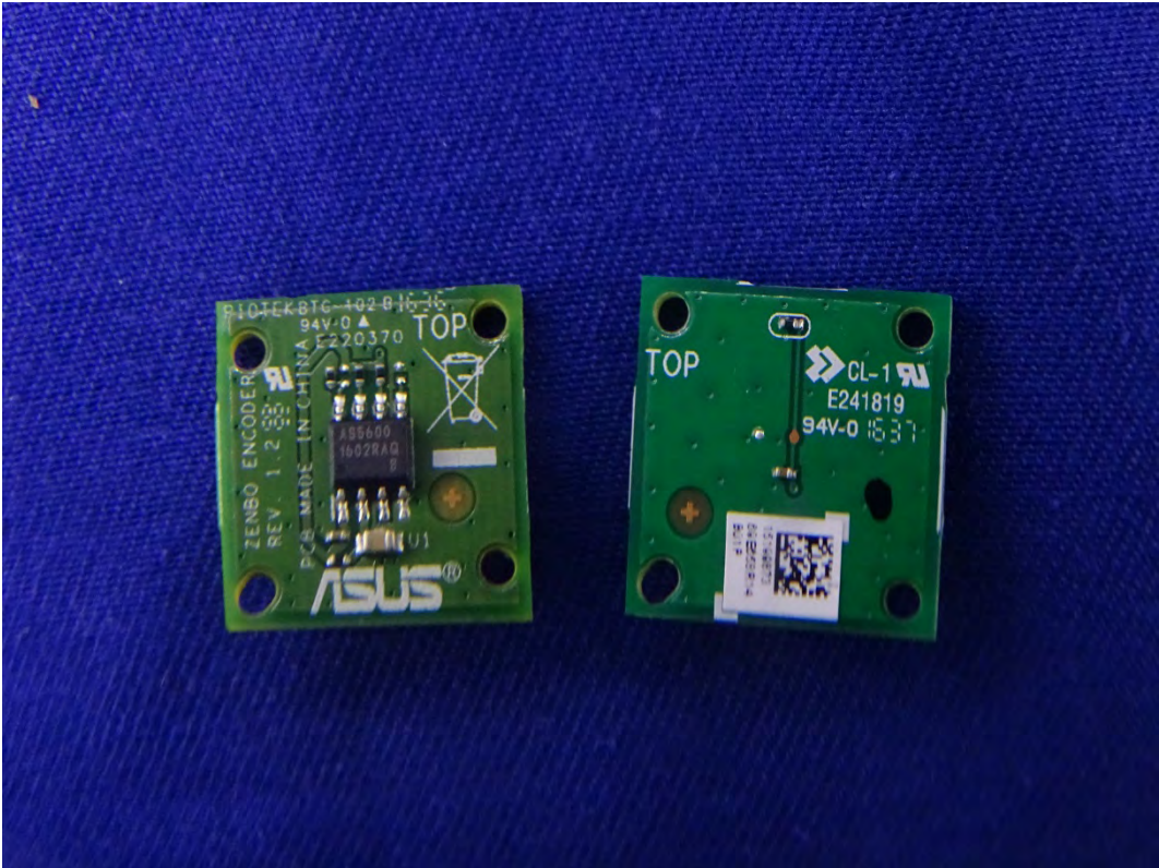
(131) EUT Photo
