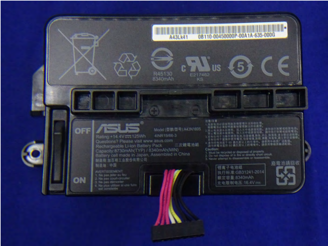
(125) EUT Photo
