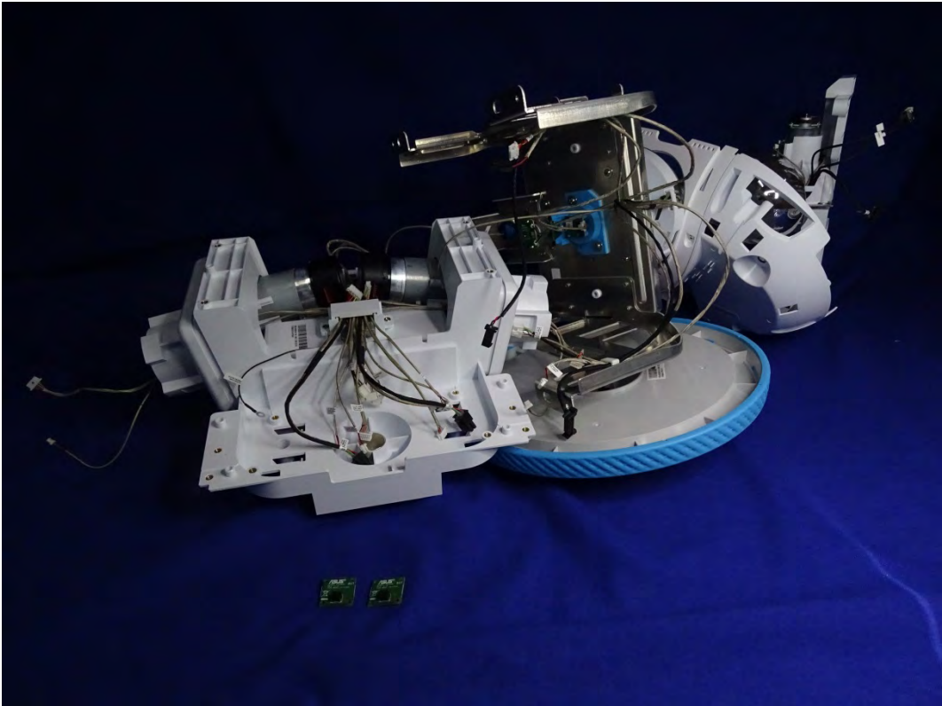
(127) EUT Photo
