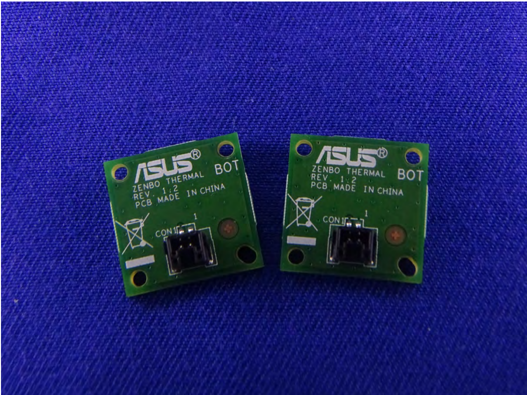
(128) EUT Photo
