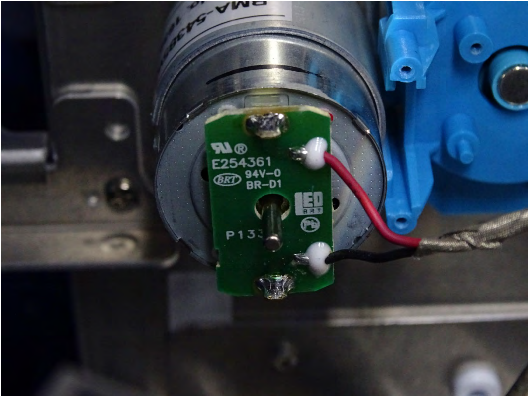
(132) EUT Photo
