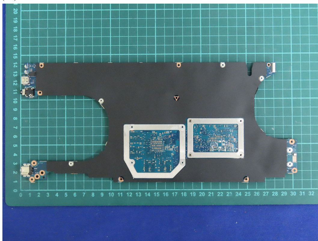
(18) EUT Photo
