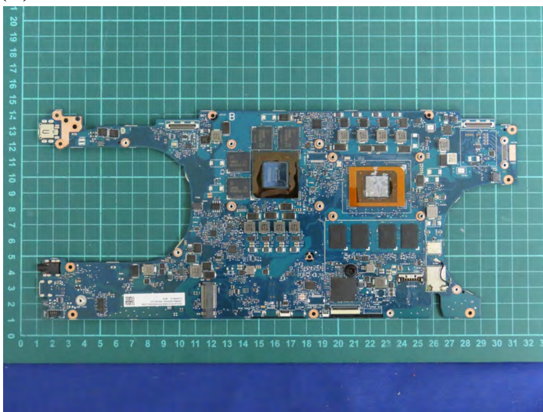
(16) EUT Photo
