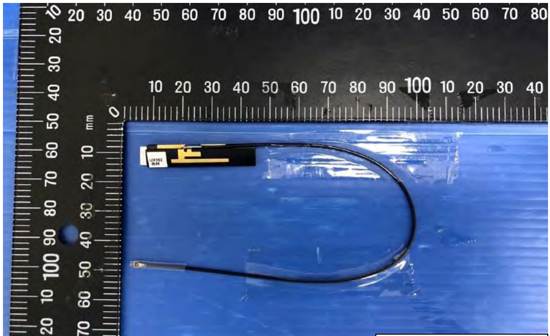
INPAQ Main Antenna Vendor MDA-LB-02-006 ASUS 14008-03200100
