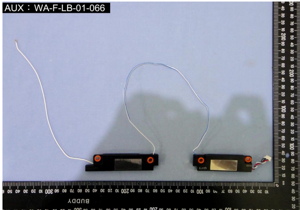
EUT Photo (46)
