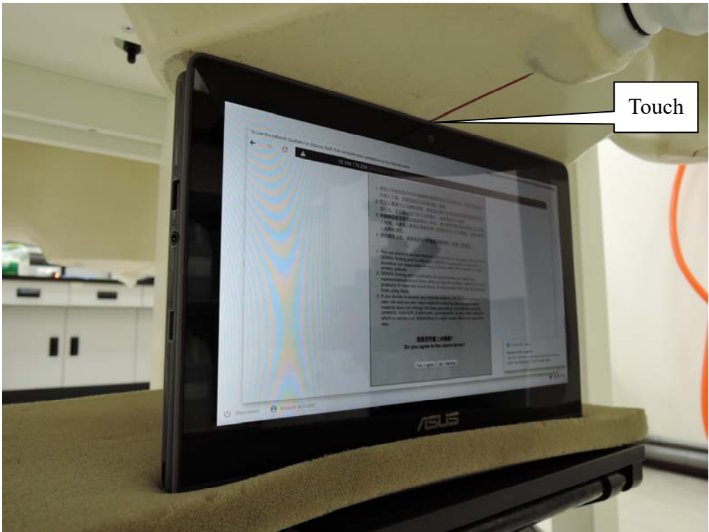
EUT Top(PAD)
