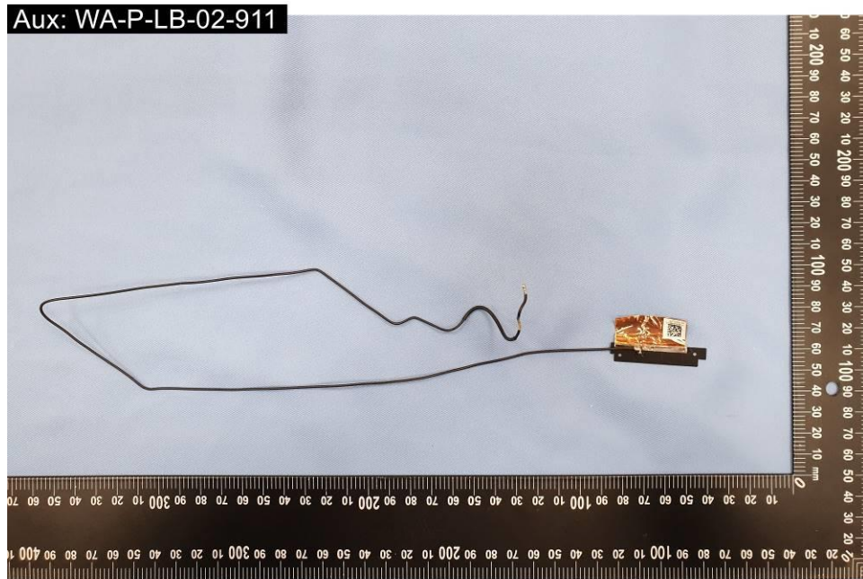
EUT Photo (16)
