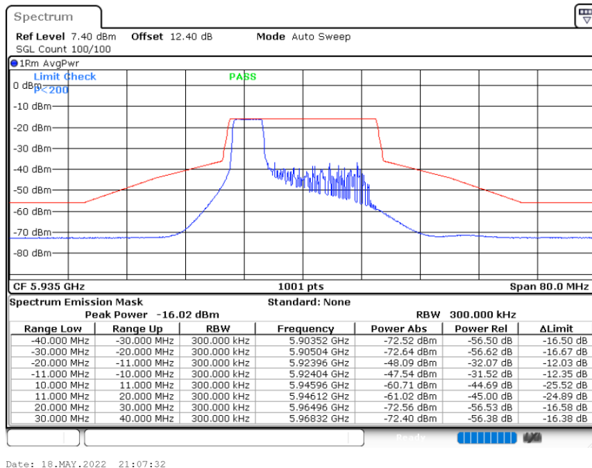
11AX20MIMO_Ant.4+5(4)_5935_52Tone_RU37
