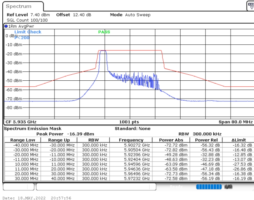
11AX20MIMO_Ant.4+5(4)_5935_52Tone_RU37
