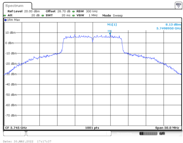
MIMO Ant. 6
