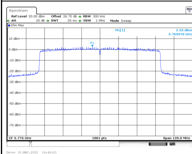
MIMO Ant. 5
