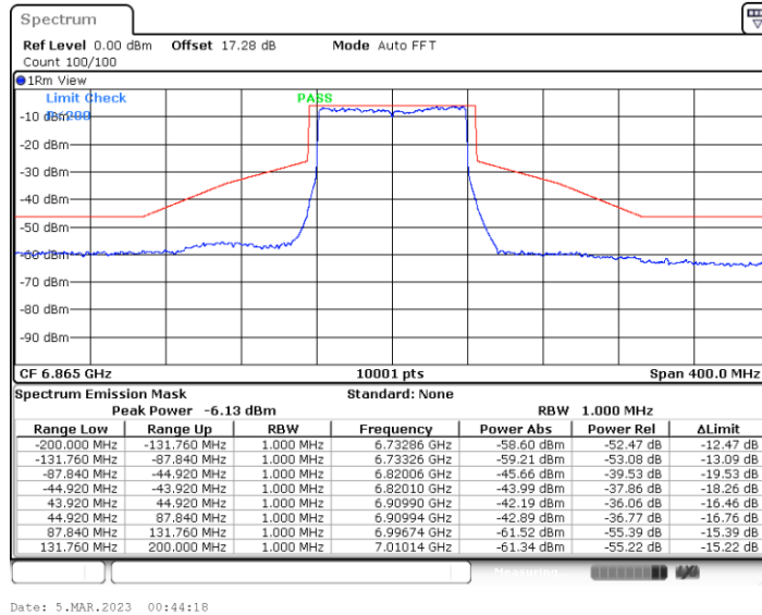
11BE80MIMO_Ant2_6865
