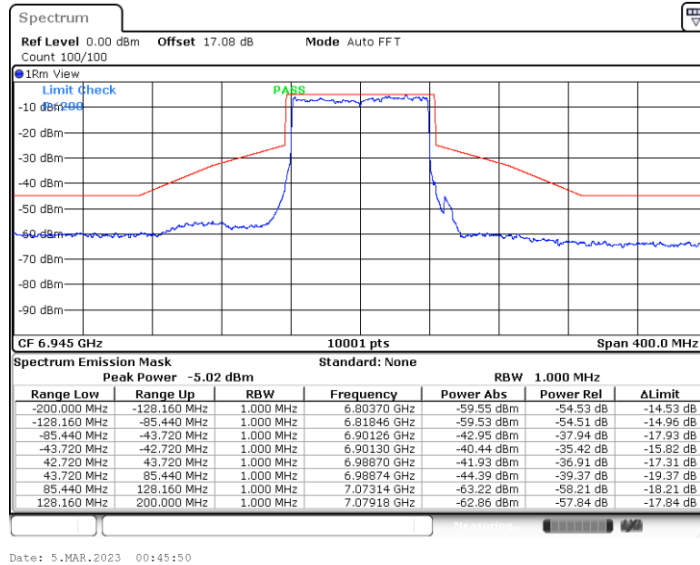
11BE80MIMO_Ant2_6945
