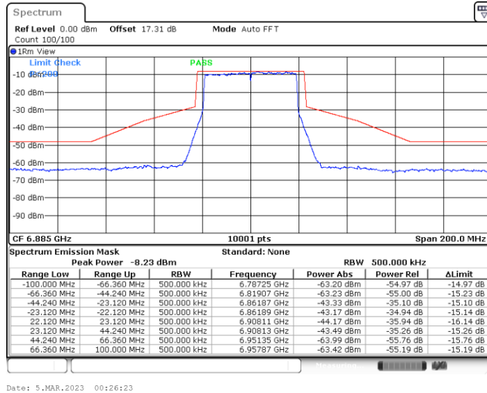
11BE40MIMO_Ant2_6885
