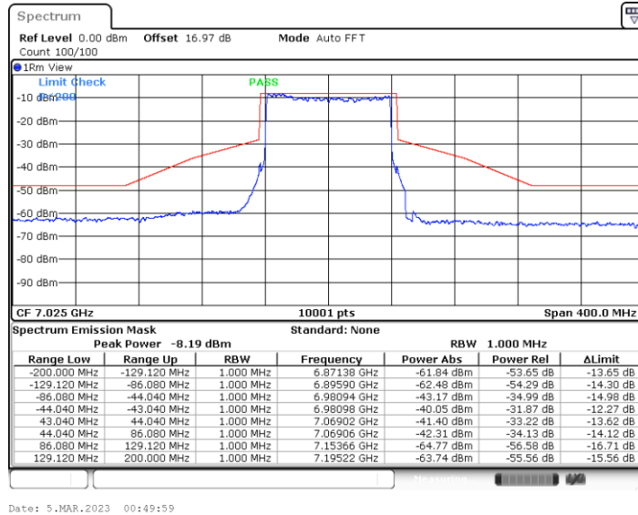
11BE80MIMO_Ant2_7025
