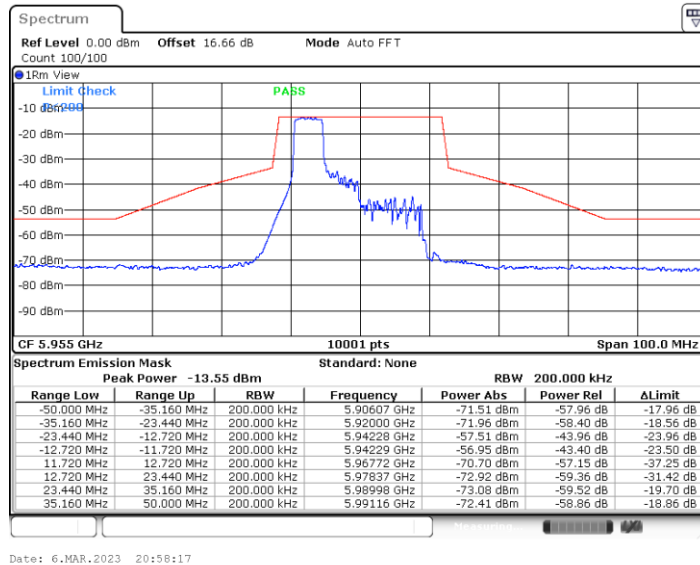
11BE20MIMO_Ant5_5955_106Tone_RU53
