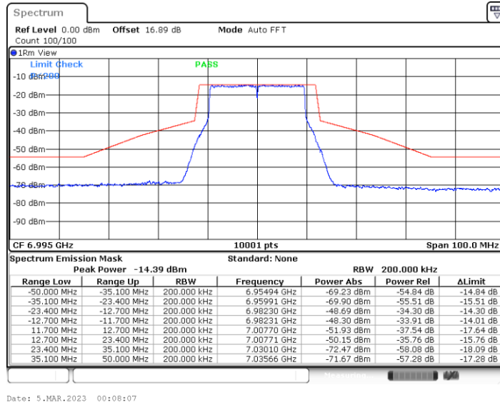
11BE20MIMO_Ant2_6995
