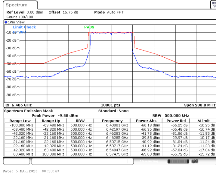
11BE40MIMO_Ant2_6485
