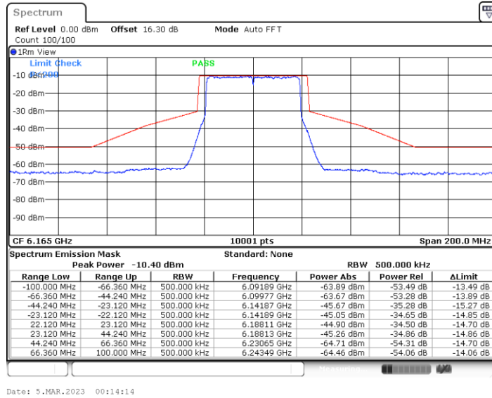
11BE40MIMO_Ant2_6165
