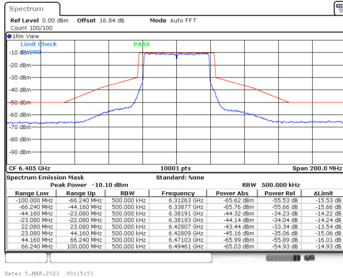
11BE40MIMO_Ant2_6405
