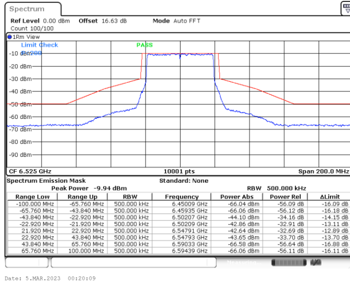
11BE40MIMO_Ant2_6525
