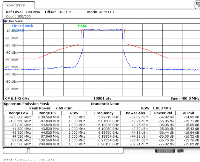
11BE80MIMO_Ant2_6145
