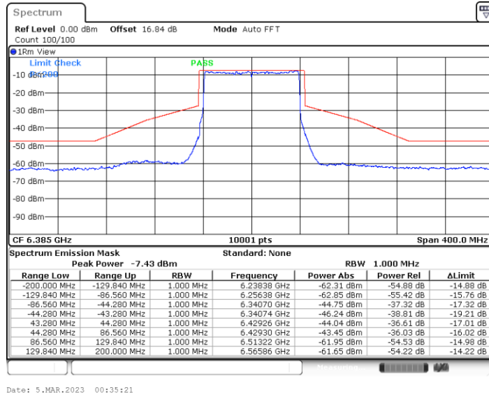
11BE80MIMO_Ant2_6385
