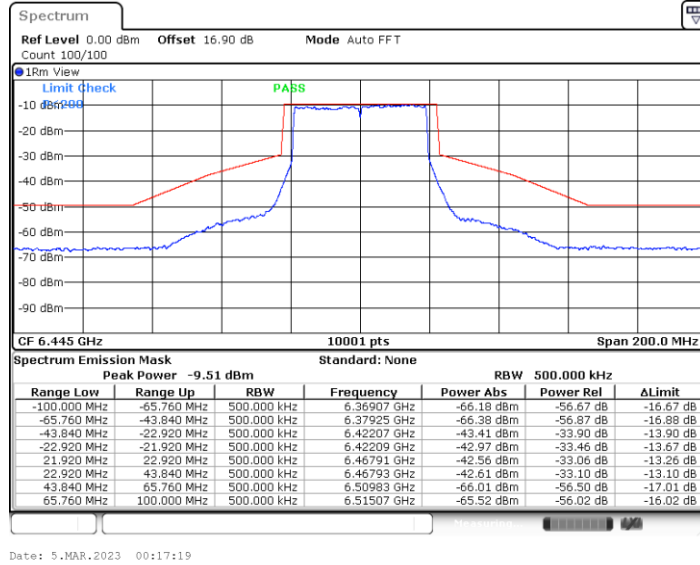
11BE40MIMO_Ant2_6445
