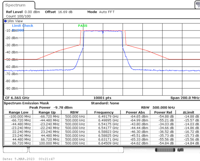
11BE40MIMO_Ant2_6565
