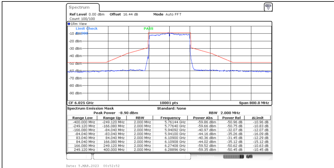
11BE160MIMO_Ant2_6025
