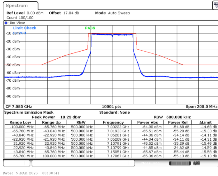
11BE40MIMO_Ant2_7085
