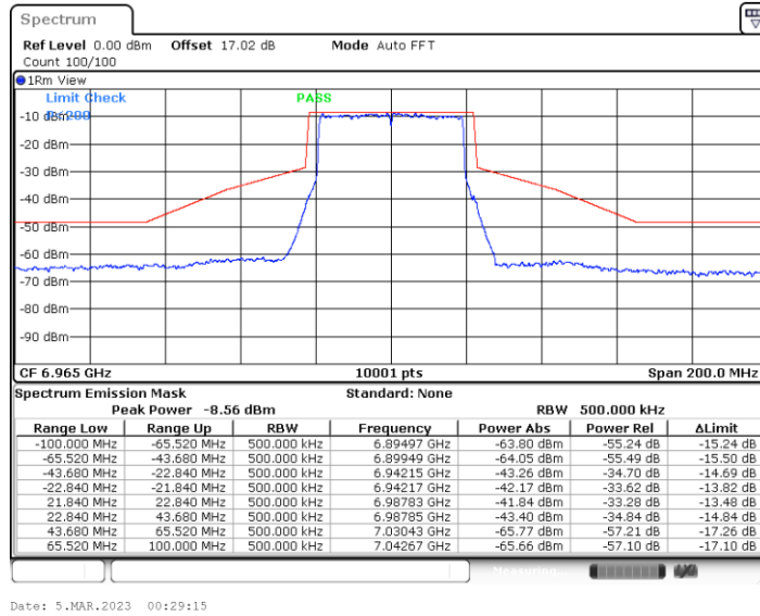
11BE40MIMO_Ant2_6965
