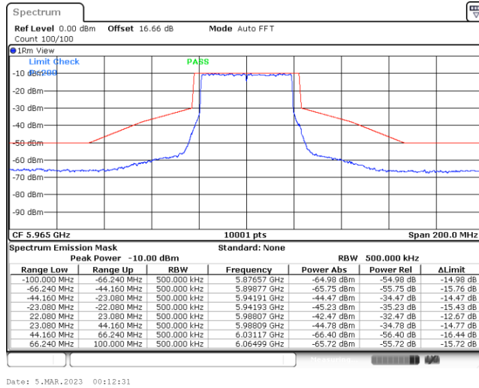
11BE40MIMO_Ant2_5965
