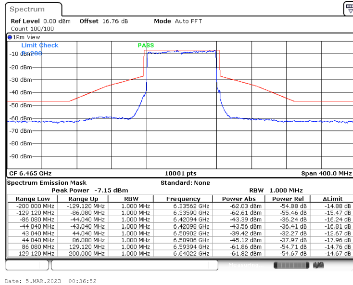
11BE80MIMO_Ant2_6465
