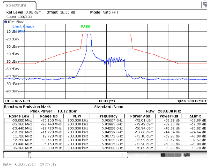
11BE20MIMO_Ant5_5955_52Tone_RU37
