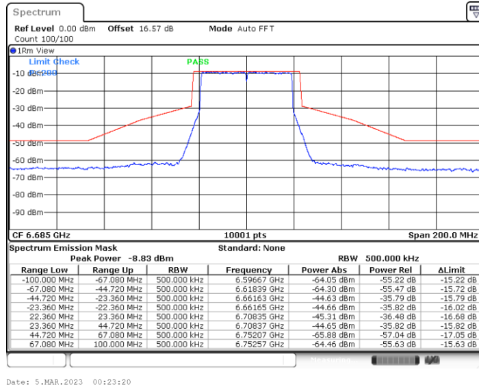
11BE40MIMO_Ant2_6685
