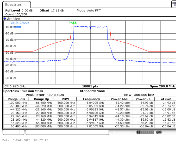
11BE40MIMO_Ant2_6925
