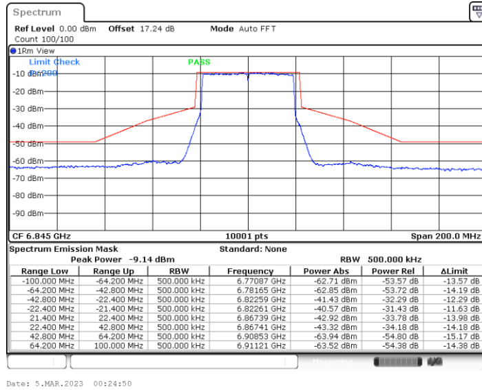
11BE40MIMO_Ant2_6845
