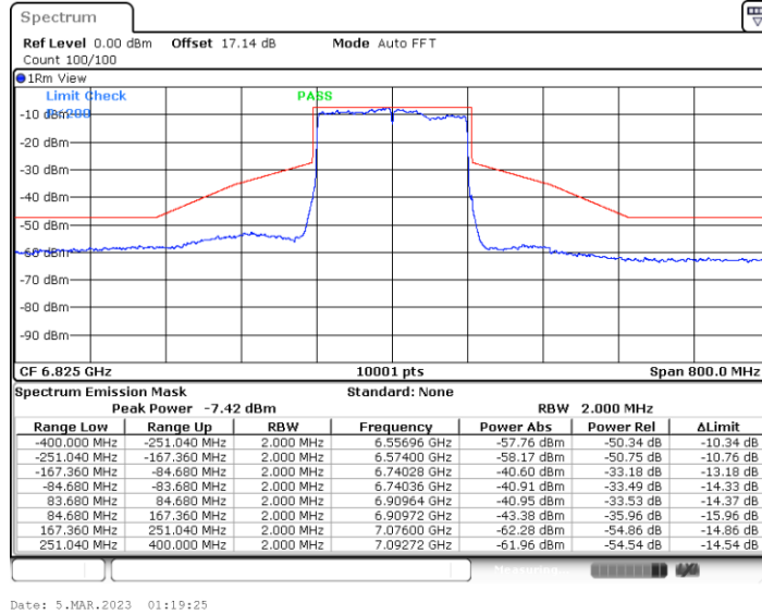
11BE160MIMO_Ant2_6825
