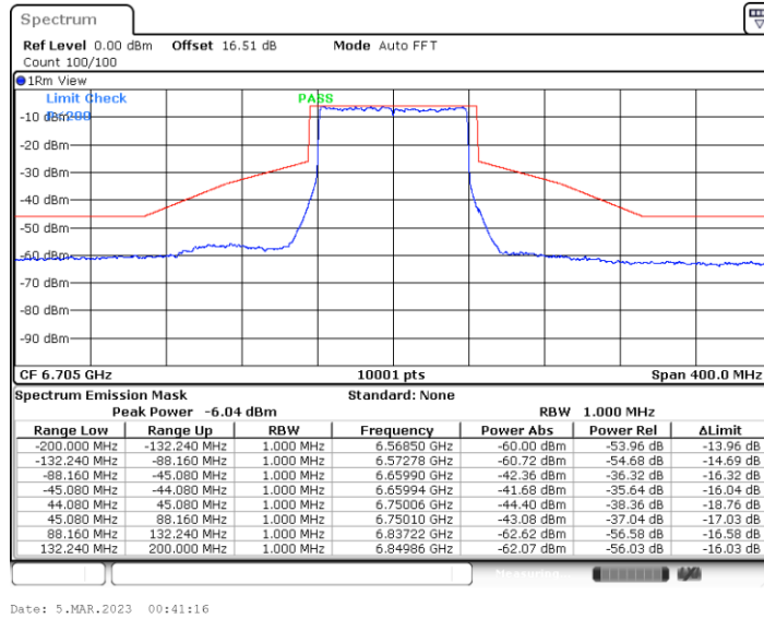
11BE80MIMO_Ant2_6705
