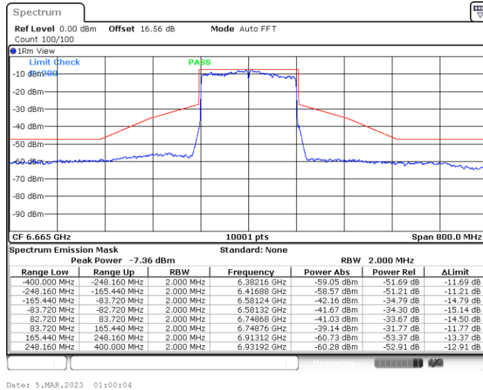
11BE160MIMO_Ant2_6665
