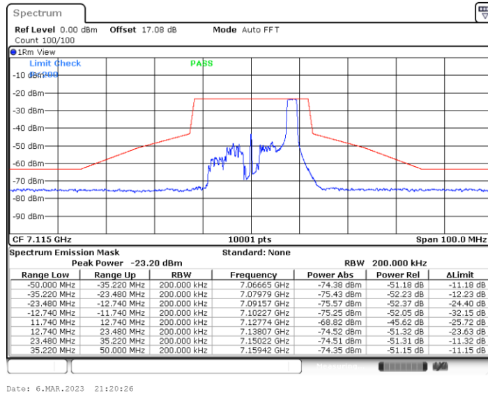
11BE20MIMO_Ant5_7115_106Tone_RU54
