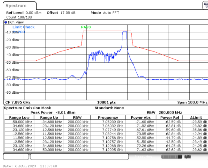
11BE20MIMO_Ant5_7095_106Tone_RU54
