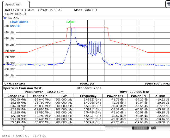
11BE20MIMO_Ant5_6535_52Tone_RU37
