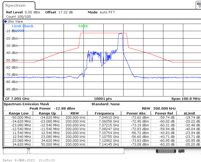
11BE20MIMO_Ant6_7095_52Tone_RU40
