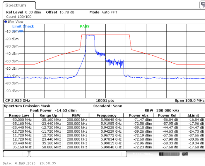
11BE20MIMO_Ant6_5955_106Tone_RU53
