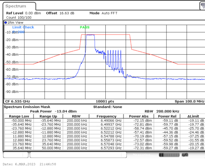
11BE20MIMO_Ant5_6535_106Tone_RU53
