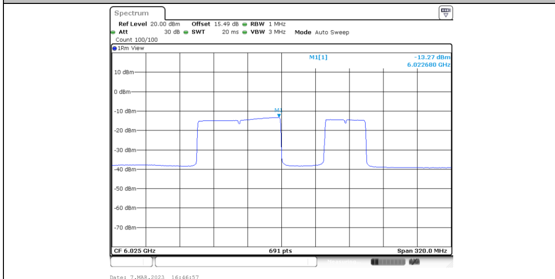
11BE160MIMO_Ant4_6025_Puncturing 40M_4
