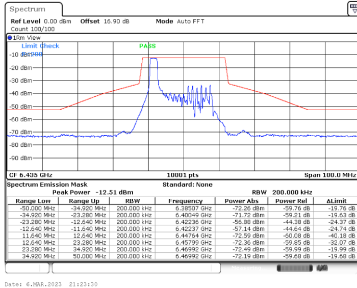
11BE20MIMO_Ant5_6435_52Tone_RU37
