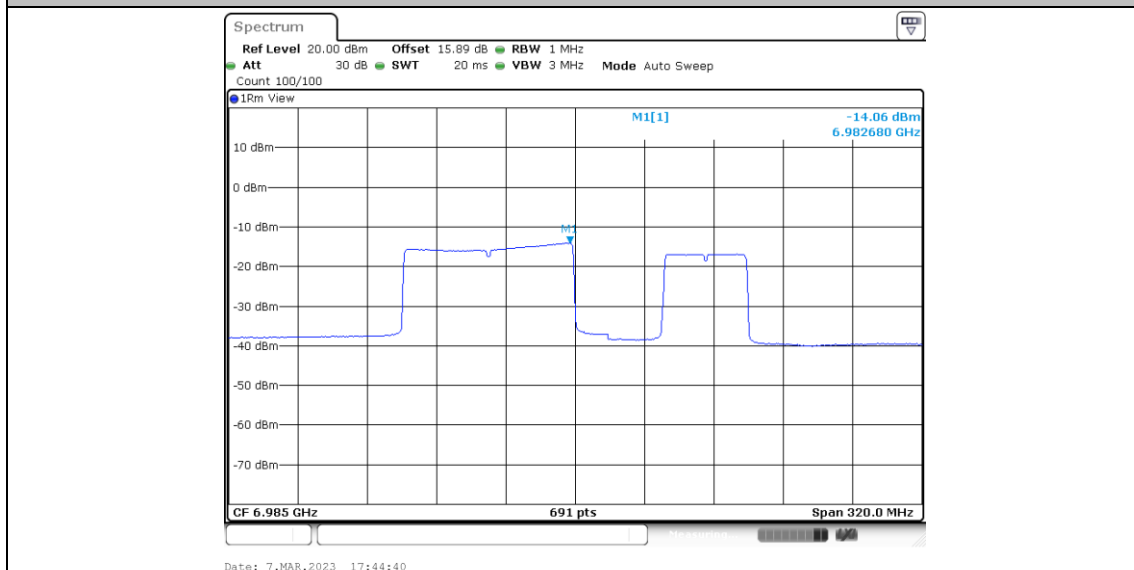
11BE160MIMO_Ant4_6985_Puncturing 40M_4
