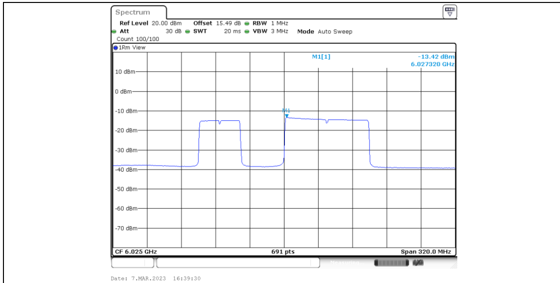
11BE160MIMO_Ant4_6025_Puncturing 40M_3
