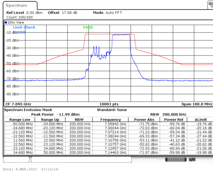
11BE20MIMO_Ant6_7095_26Tone_RU8
