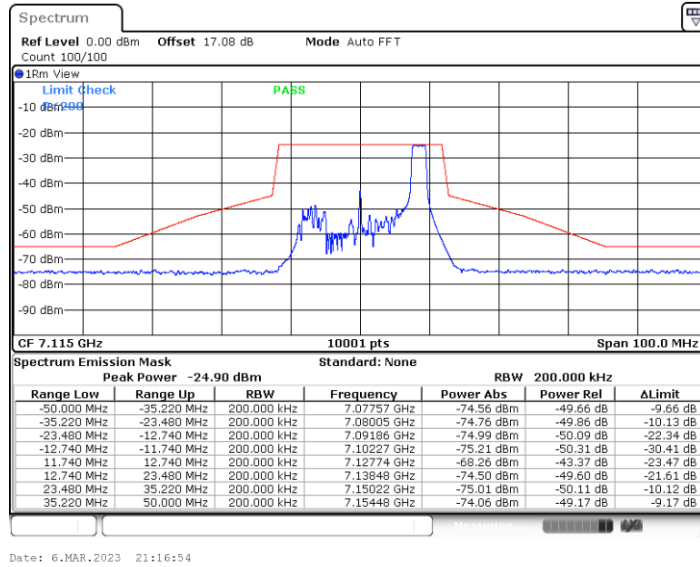
11BE20MIMO_Ant5_7115_52Tone_RU40
