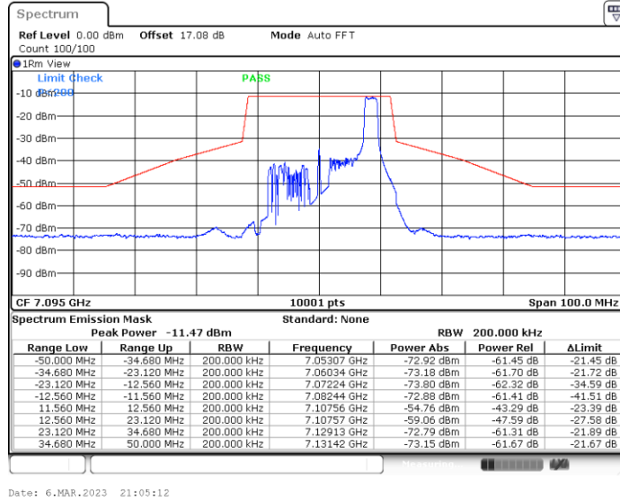
11BE20MIMO_Ant5_7095_52Tone_RU40
