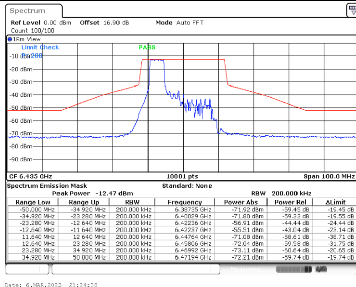
11BE20MIMO_Ant5_6435_106Tone_RU53
