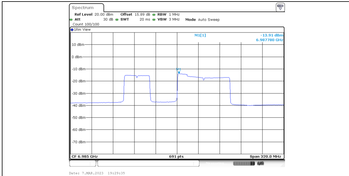
11BE160MIMO_Ant4_6985_Puncturing 40M_3
