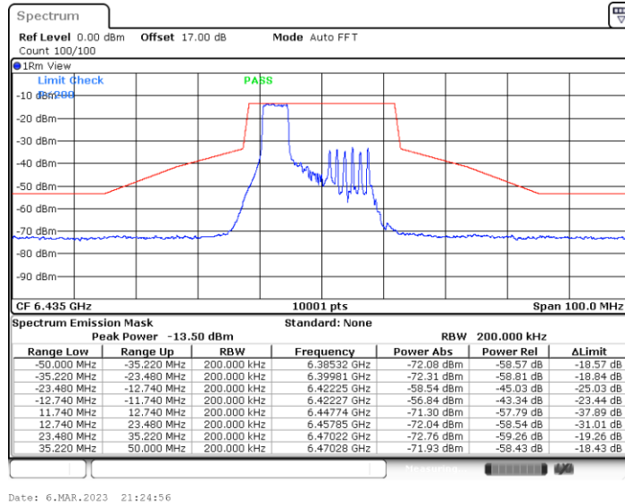
11BE20MIMO_Ant6_6435_106Tone_RU53
