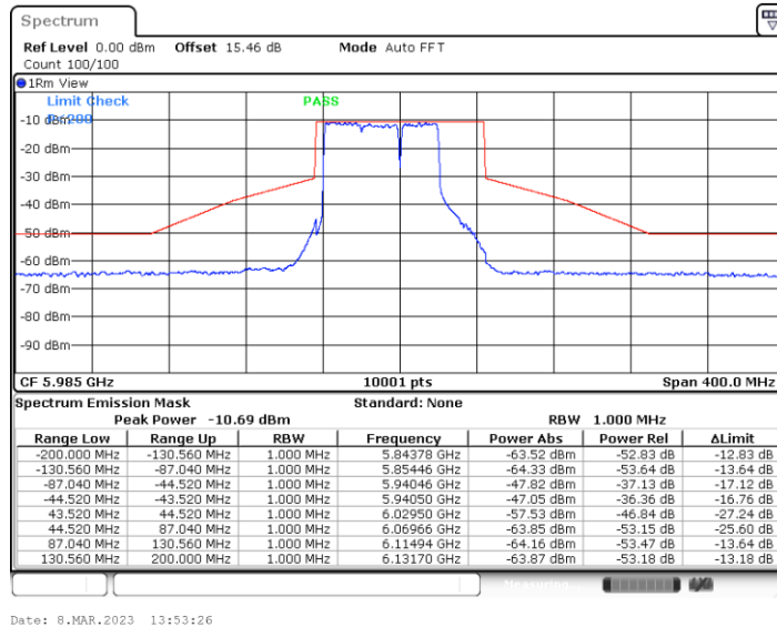
11BE80MIMO_Ant5_5985_Puncturing 20M_1
