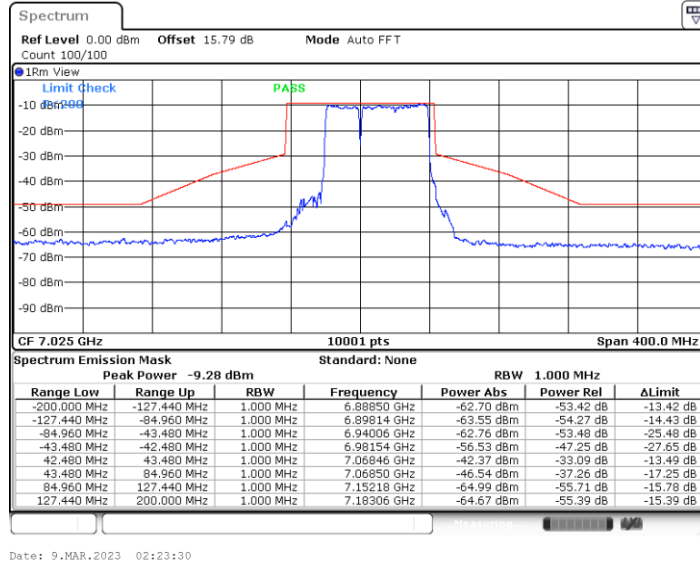
11BE80MIMO_Ant4_7025_Puncturing 20M_2
