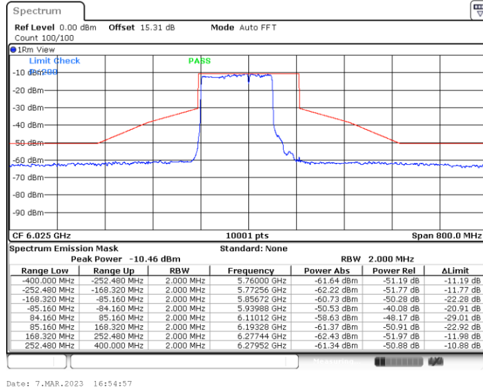
11BE160MIMO_Ant4_6025_Puncturing 20M_1
