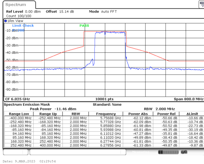
11BE160MIMO_Ant5_6025_Puncturing 40M_2
