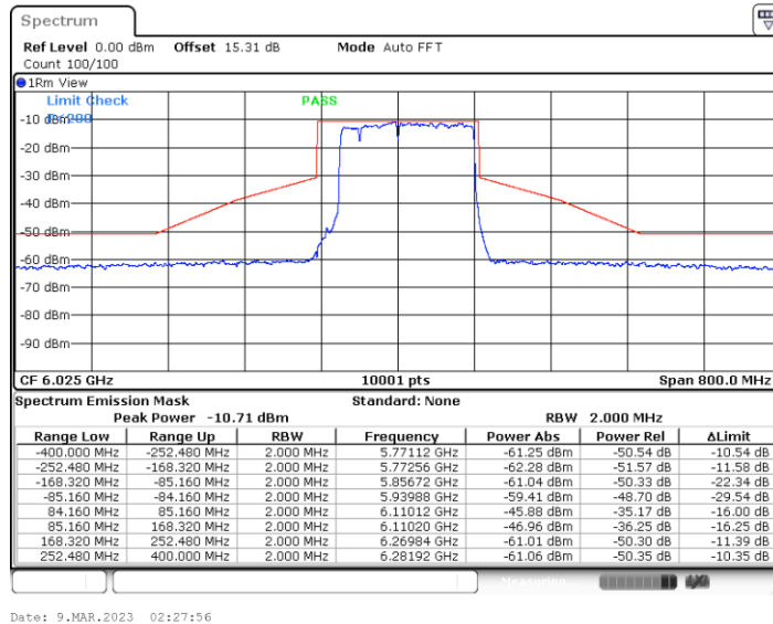
11BE160MIMO_Ant4_6025_Puncturing 20M_2
