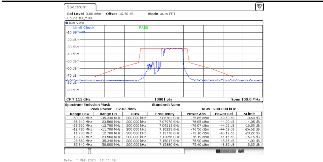
11BE20MIMO_Ant4_7115_52+26_OFDMA_3
