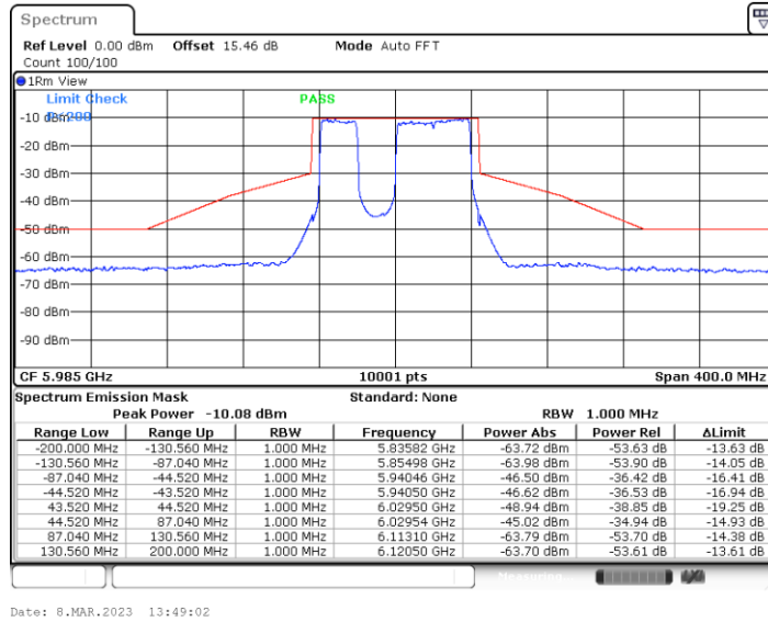
11BE80MIMO_Ant5_5985_Large RU 484+242_4
