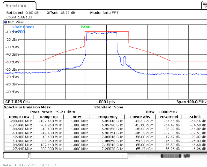
11BE80MIMO_Ant4_7025_Puncturing 20M_1
