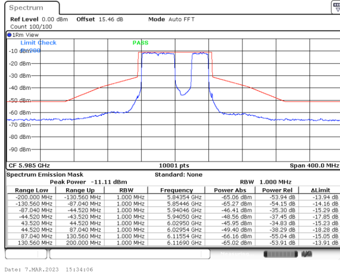
11BE80MIMO_Ant5_5985_Puncturing 20M_4
