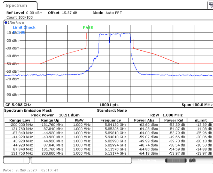
11BE80MIMO_Ant4_5985_Puncturing 20M_2
