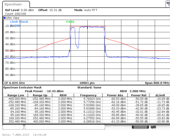
11BE160MIMO_Ant4_6025_Puncturing 20M_4
