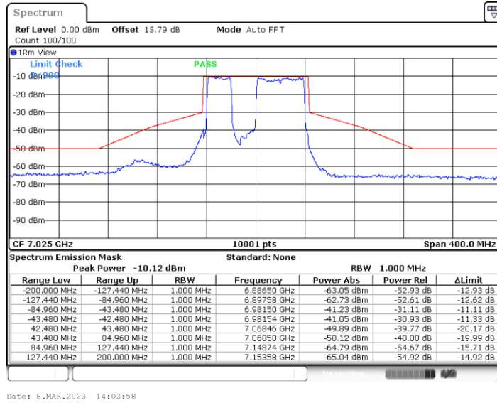
11BE80MIMO_Ant4_7025_Large RU 484+242_4
