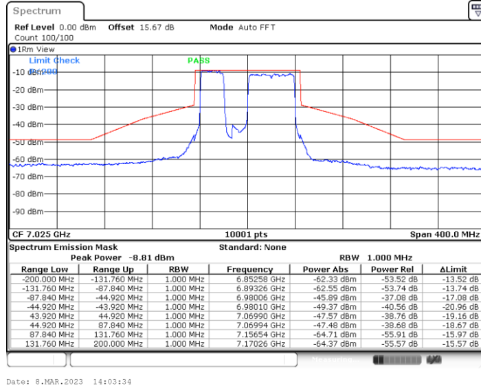
11BE80MIMO_Ant5_7025_Large RU 484+242_4
