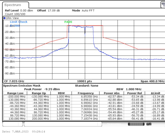
11BE80MIMO_Ant6_7025_Puncturing 20M_1
