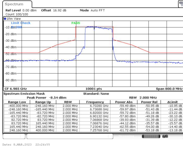
11BE160MIMO_Ant5_6985_Puncturing 40M_2
