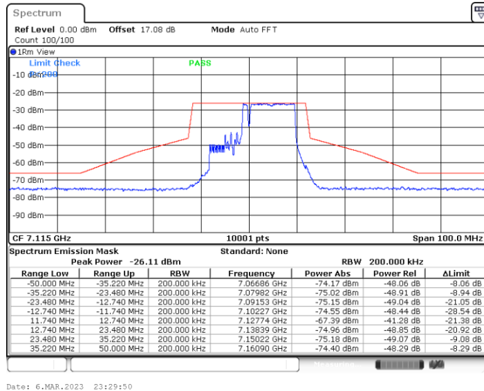
11BE20MIMO_Ant6_7115_52+26_OFDMA_3
