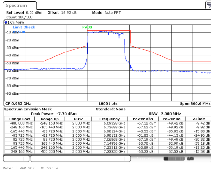
11BE160MIMO_Ant6_6985_Large RU 996+484_3
