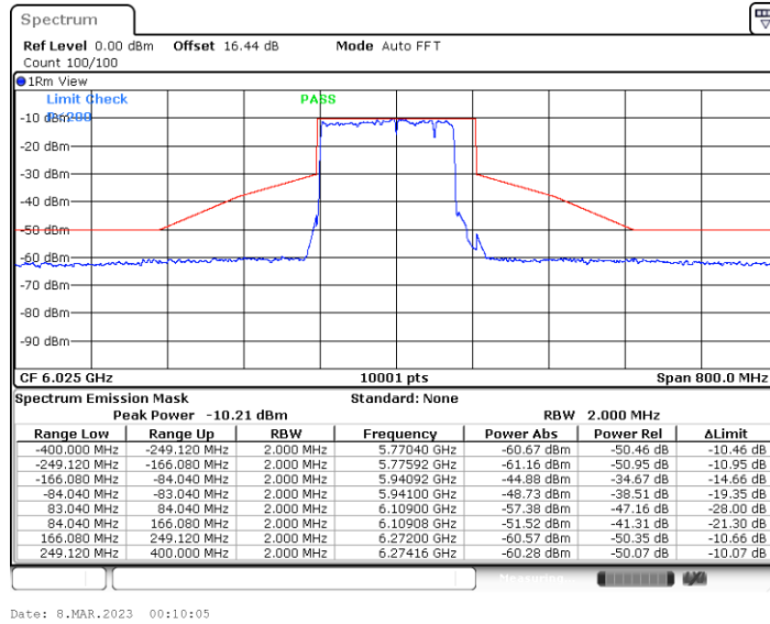
11BE160MIMO_Ant6_6025_Large RU 996+484_3
