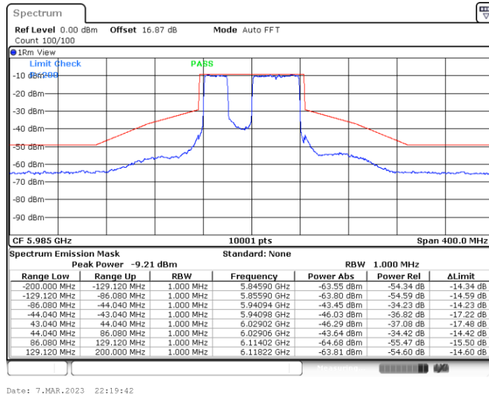
11BE80MIMO_Ant6_5985_Puncturing 20M_3
