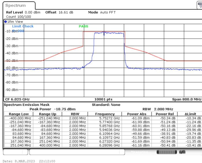
11BE160MIMO_Ant6_6025_Puncturing 40M_2
