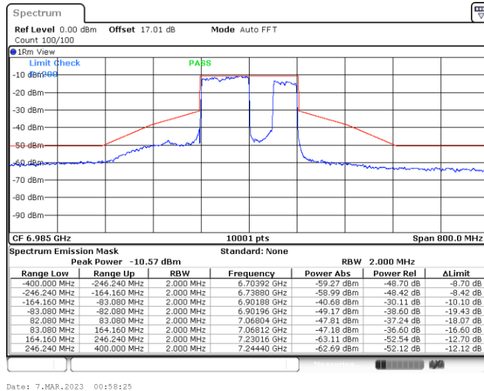
11BE160MIMO_Ant6_6985_Large RU 996+484_4
