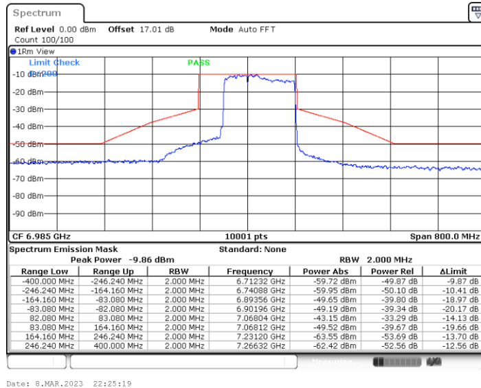
11BE160MIMO_Ant6_6985_Puncturing 40M_2
