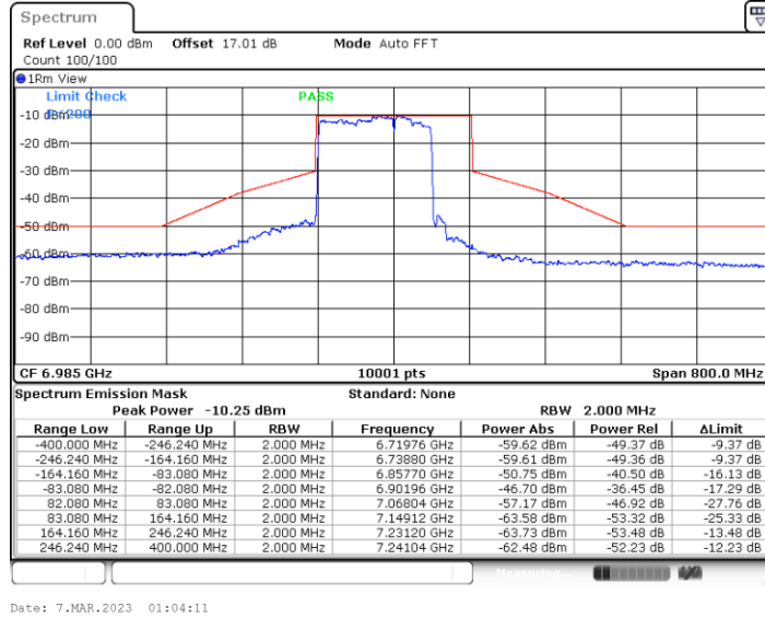
11BE160MIMO_Ant6_6985_Puncturing 40M_1
