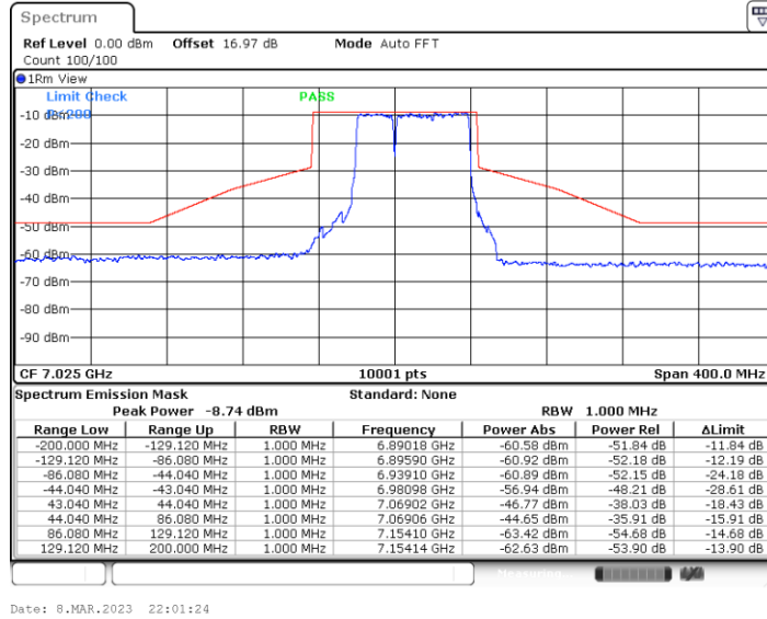
11BE80MIMO_Ant5_7025_Puncturing 20M_2
