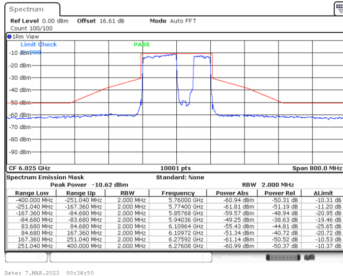
11BE160MIMO_Ant6_6025_Large RU 996+484_4
