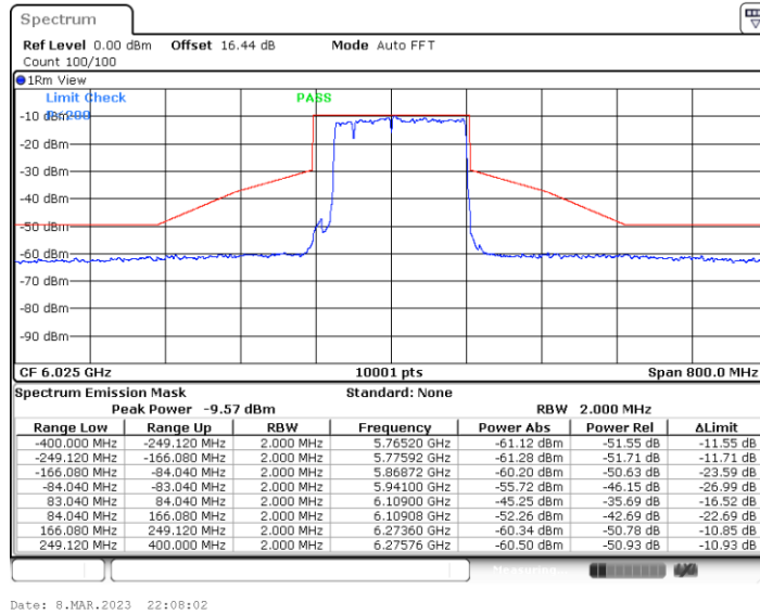
11BE160MIMO_Ant5_6025_Puncturing 20M_2
