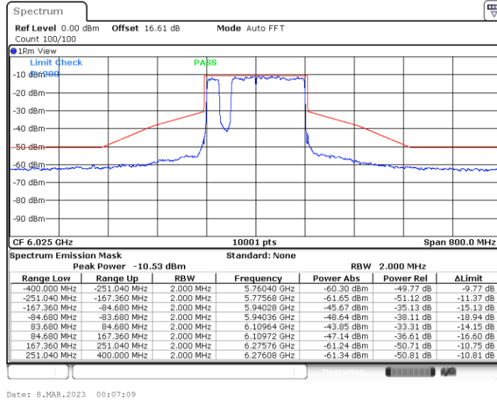
11BE160MIMO_Ant6_6025_Puncturing 20M_4
