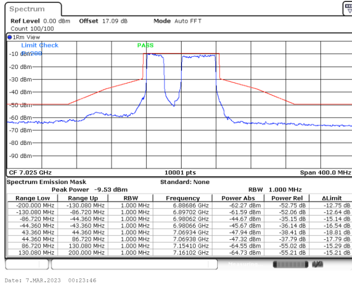
11BE80MIMO_Ant6_7025_Large RU 484+242_4
