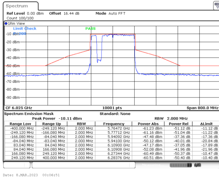
11BE160MIMO_Ant5_6025_Puncturing 20M_4
