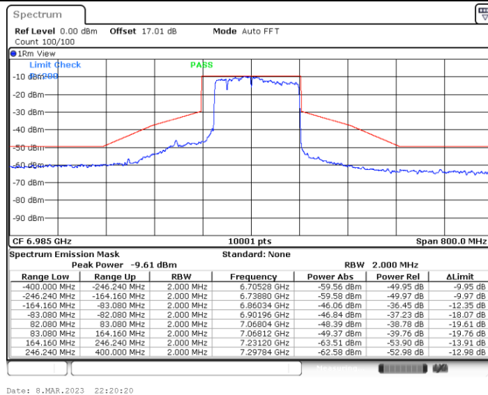
11BE160MIMO_Ant6_6985_Puncturing 20M_2
