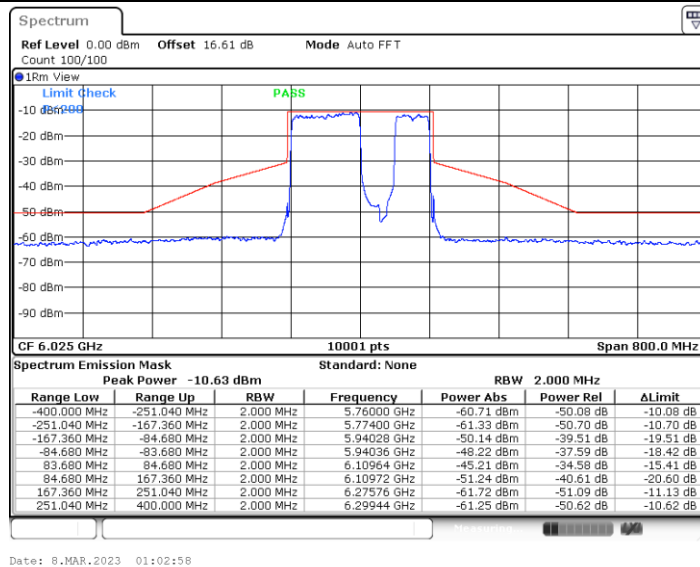
11BE160MIMO_Ant6_6025_Puncturing 40M_4
