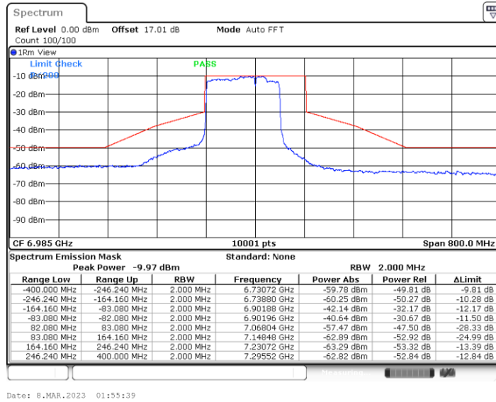
11BE160MIMO_Ant6_6985_Puncturing 20M_1
