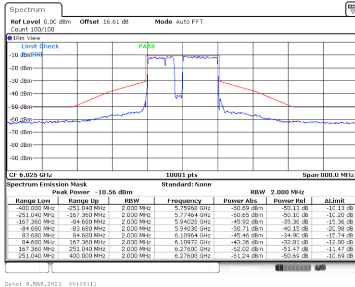
11BE160MIMO_Ant6_6025_Puncturing 20M_6
