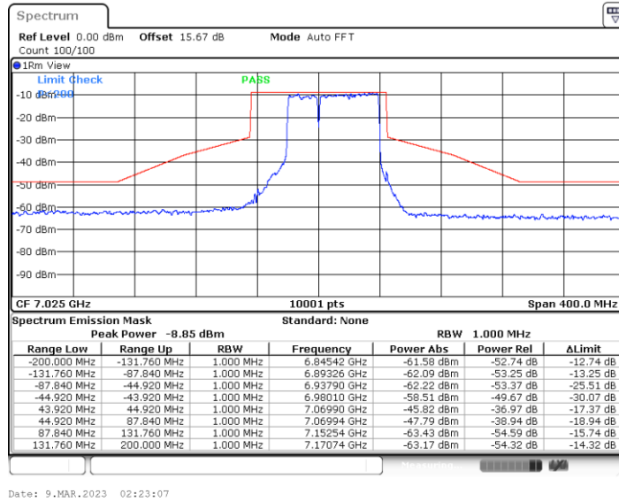
11BE80MIMO_Ant5_7025_Puncturing 20M_2
