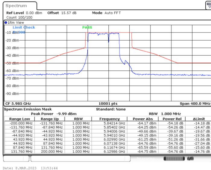
11BE80MIMO_Ant4_5985_Puncturing 20M_1
