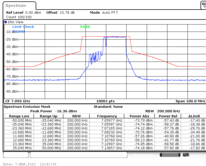
11BE20MIMO_Ant4_7095_52+26_OFDMA_3
