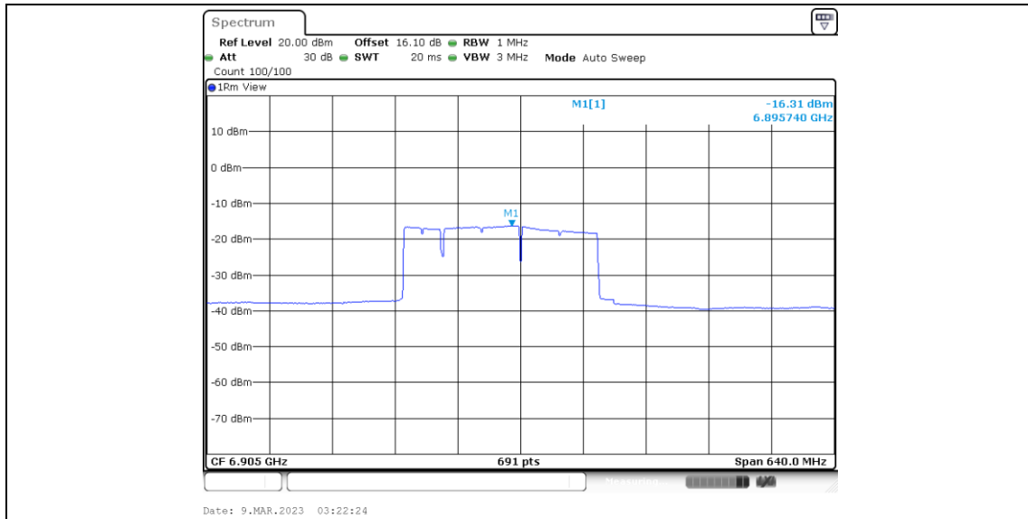
11BE320MIMO_Ant4_6905_Puncturing 80M+40M_3
