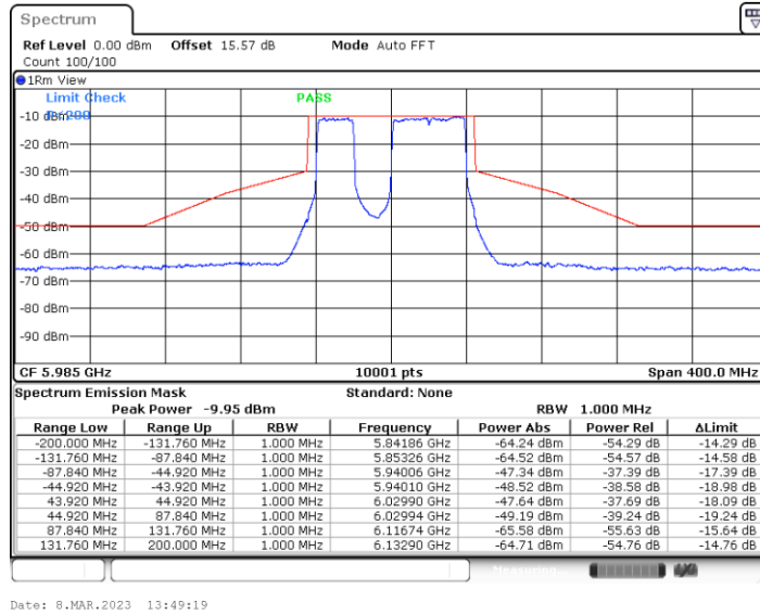
11BE80MIMO_Ant4_5985_Large RU 484+242_4
