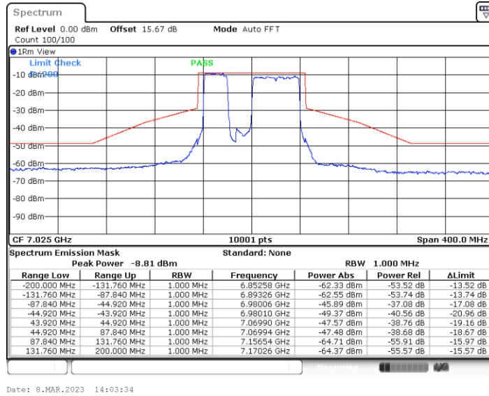
11BE80MIMO_Ant5_7025_Large RU 484+242_4
