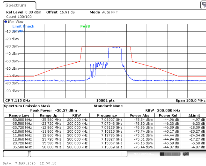
11BE20MIMO_Ant4_7115_106+26_OFDMA_2
