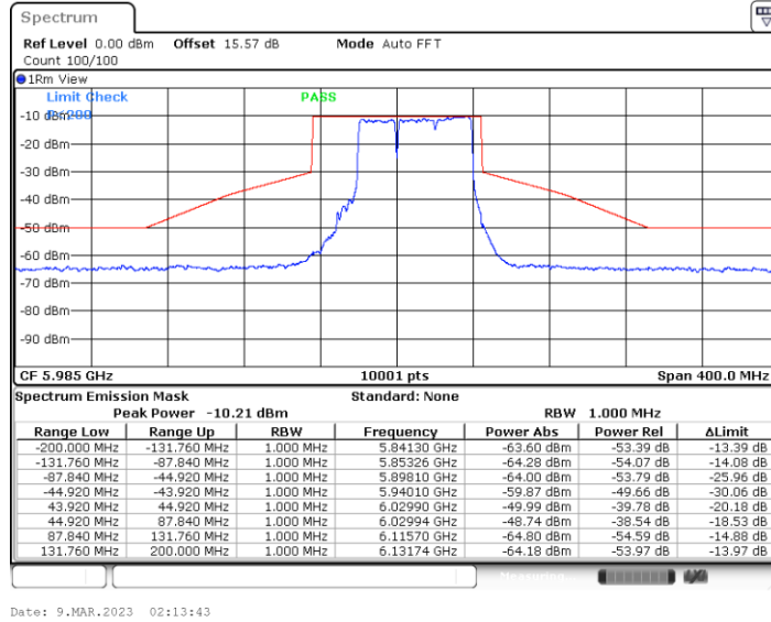
11BE80MIMO_Ant4_5985_Puncturing 20M_2
