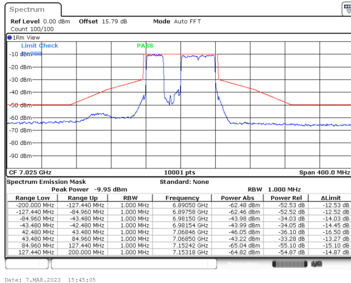
11BE80MIMO_Ant4_7025_Puncturing 20M_3
