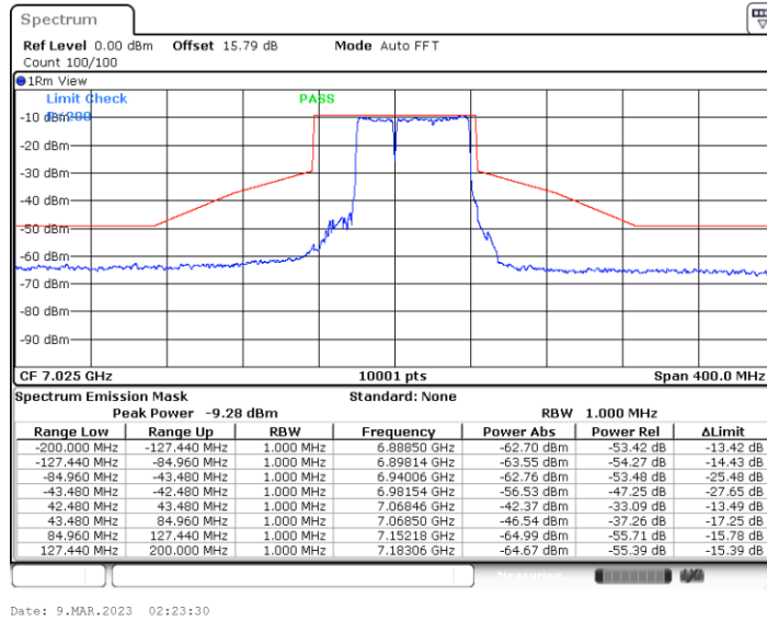
11BE80MIMO_Ant4_7025_Puncturing 20M_2
