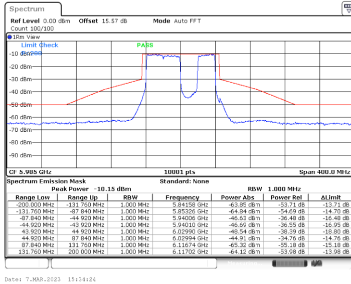
11BE80MIMO_Ant4_5985_Puncturing 20M_4
