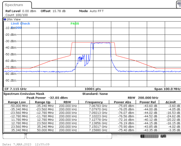
11BE20MIMO_Ant4_7115_52+26_OFDMA_3
