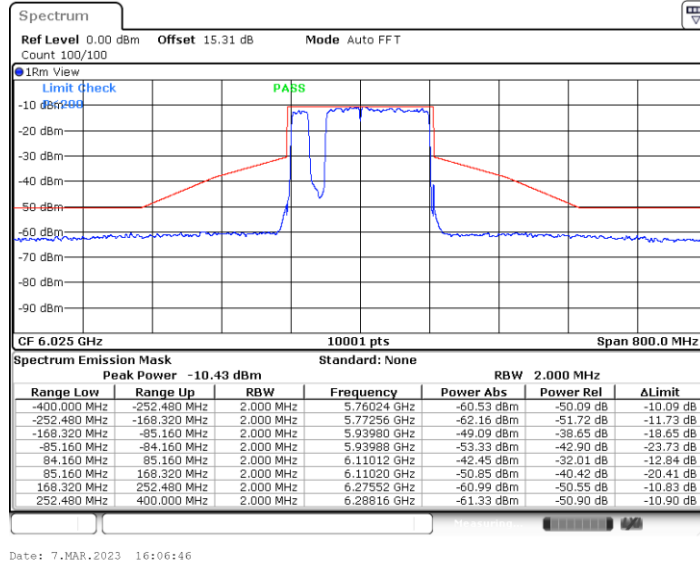
11BE160MIMO_Ant4_6025_Puncturing 20M_4
