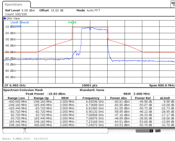
11BE160MIMO_Ant5_6985_Puncturing 40M_2
