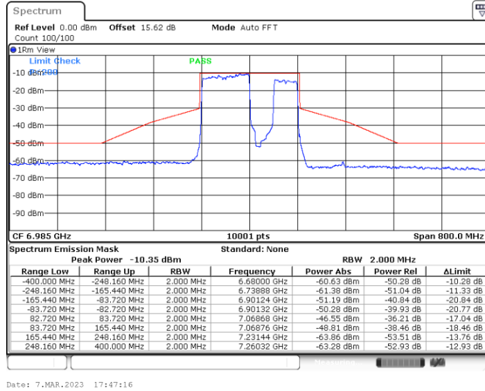
11BE160MIMO_Ant5_6985_Puncturing 40M_4
