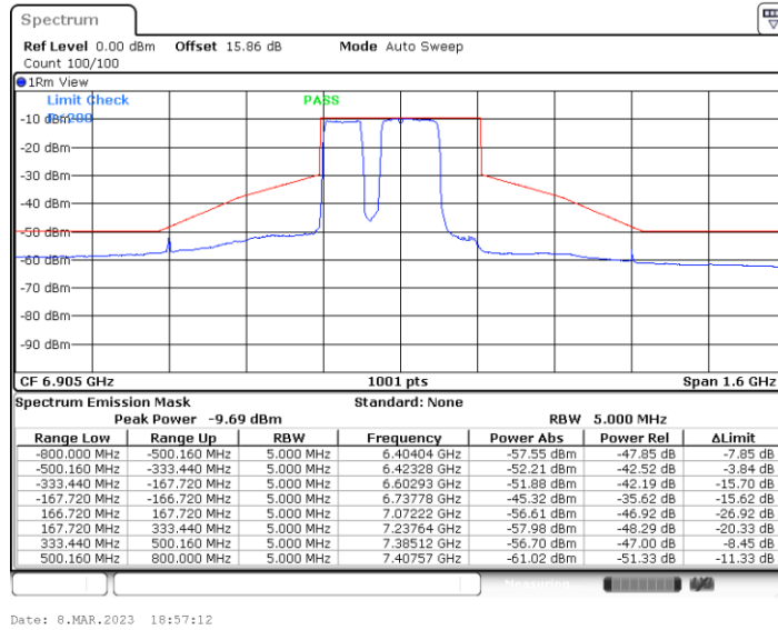
11BE320MIMO_Ant5_6905_Large RU 996*2+484_6
