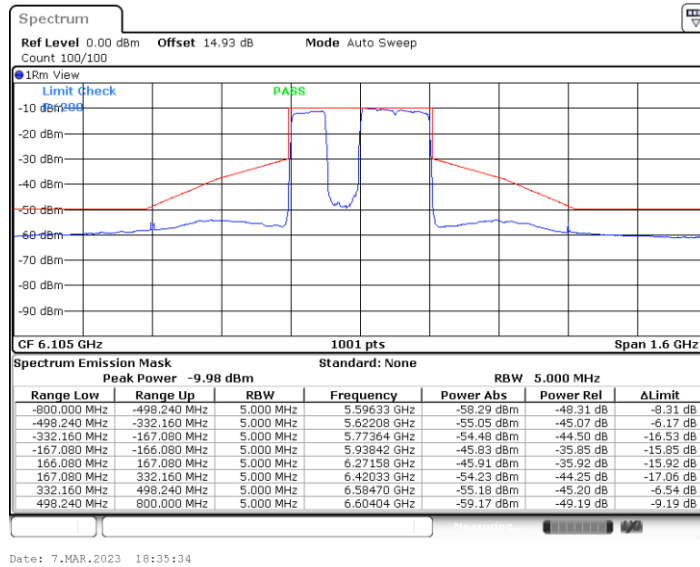
11BE320MIMO_Ant4_6105_Puncturing 80M_3
