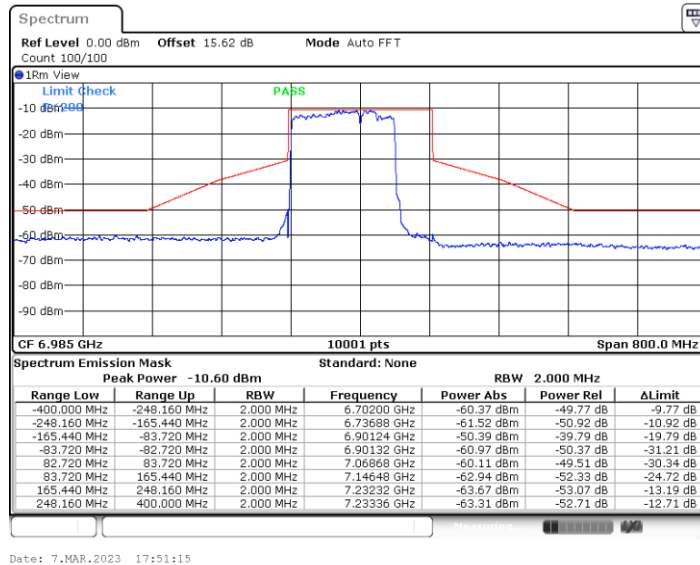
11BE160MIMO_Ant5_6985_Puncturing 20M_1
