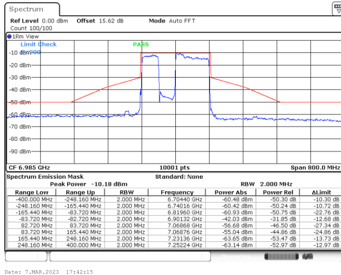
11BE160MIMO_Ant5_6985_Puncturing 40M_3
