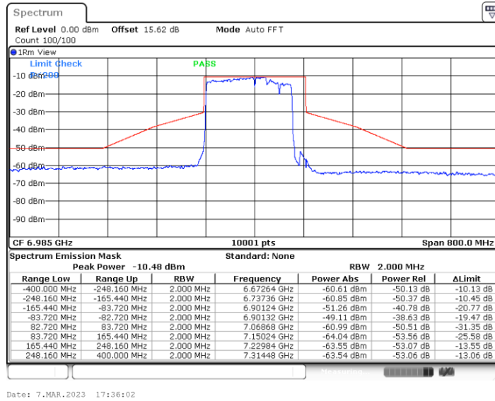
11BE160MIMO_Ant4_6985_Large RU 996+484_3
