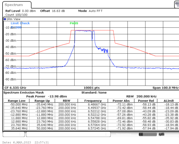
11BE20MIMO_Ant6_6535_52+26_OFDMA_1
