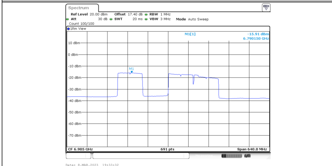
11BE320MIMO_Ant6_6905_Puncturing 80M_3
