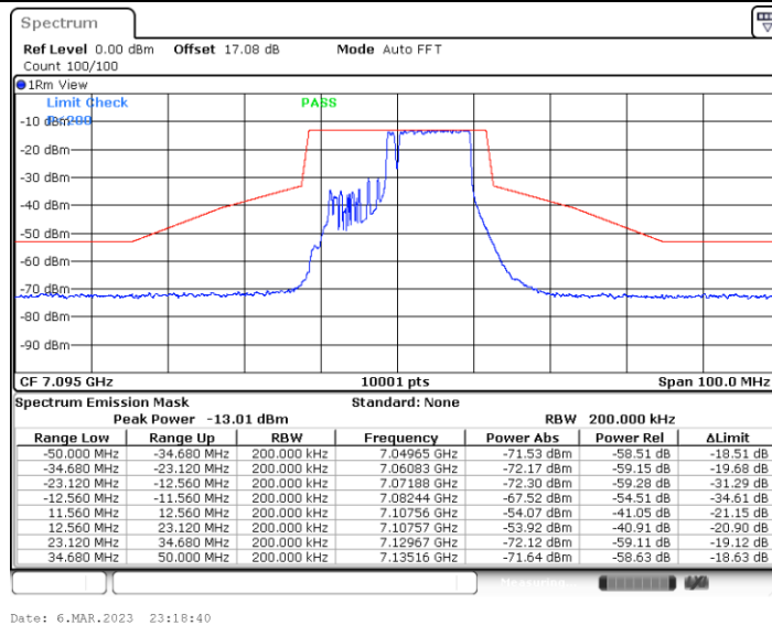
11BE20MIMO_Ant6_7095_52+26_OFDMA_3
