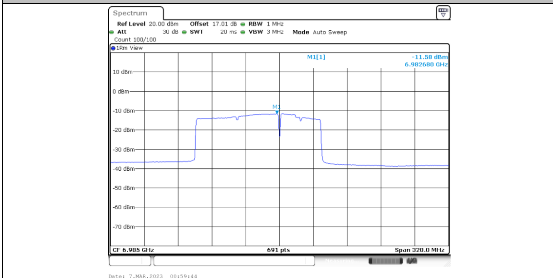
11BE160MIMO_Ant5_6985_Puncturing 40M_1
