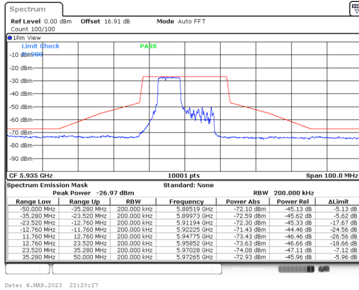
11BE20MIMO_Ant6_5935_106+26_OFDMA_1
