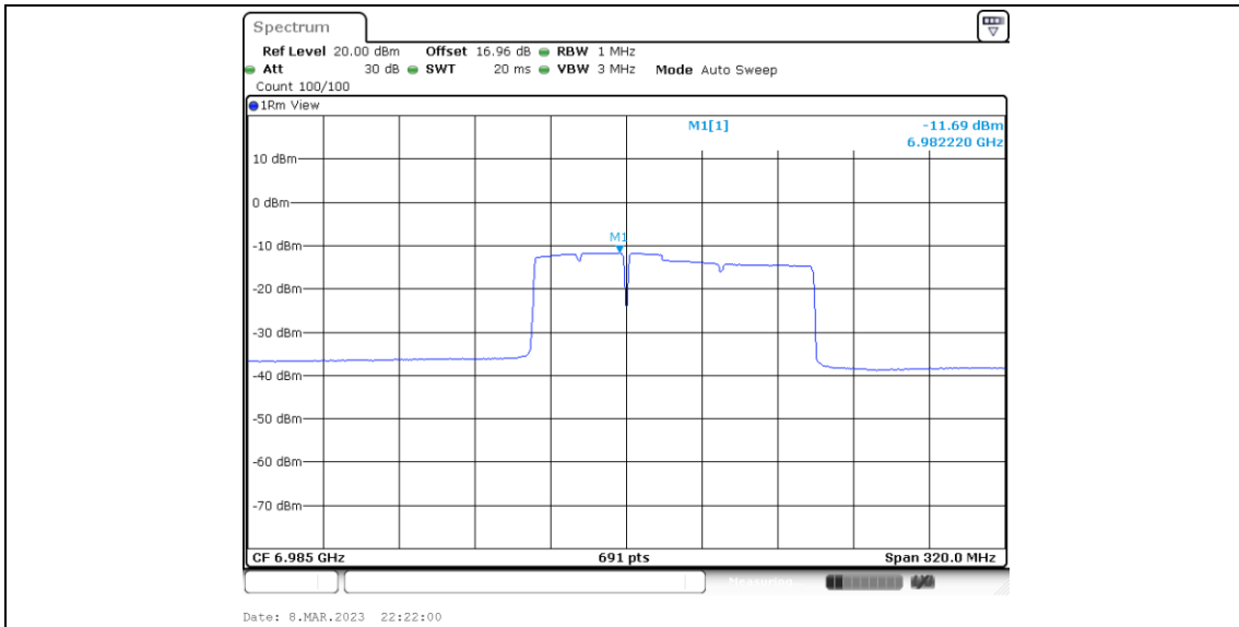
11BE160MIMO_Ant5_6985_Puncturing 40M_2
