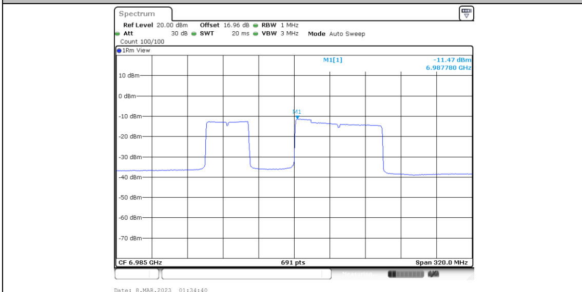
11BE160MIMO_Ant5_6985_Puncturing 40M_3
