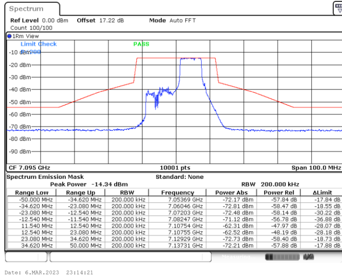
11BE20MIMO_Ant6_7095_106+26_OFDMA_2
