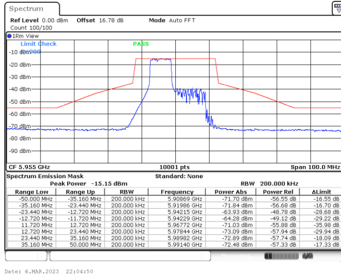
11BE20MIMO_Ant6_5955_106+26_OFDMA_1
