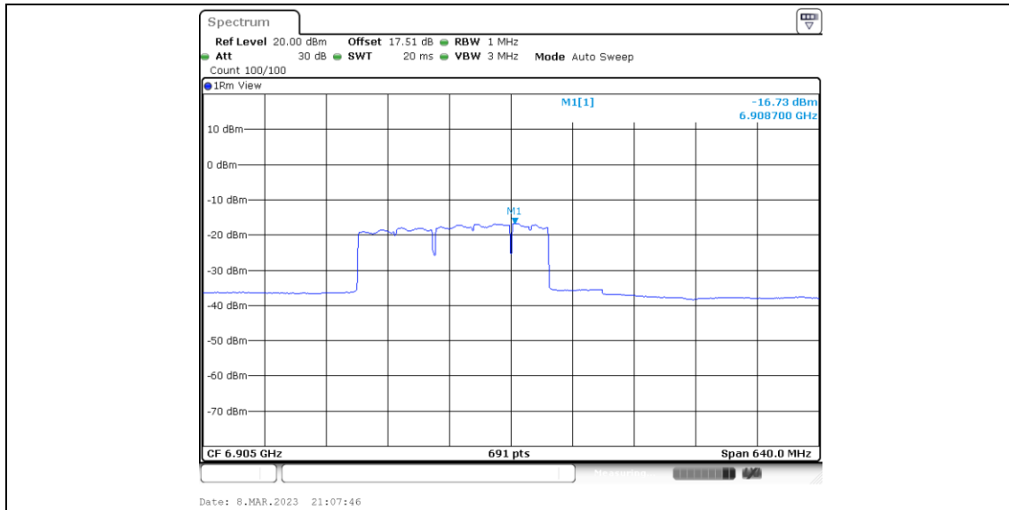
11BE320MIMO_Ant6_6905_Large RU 996*3_4
