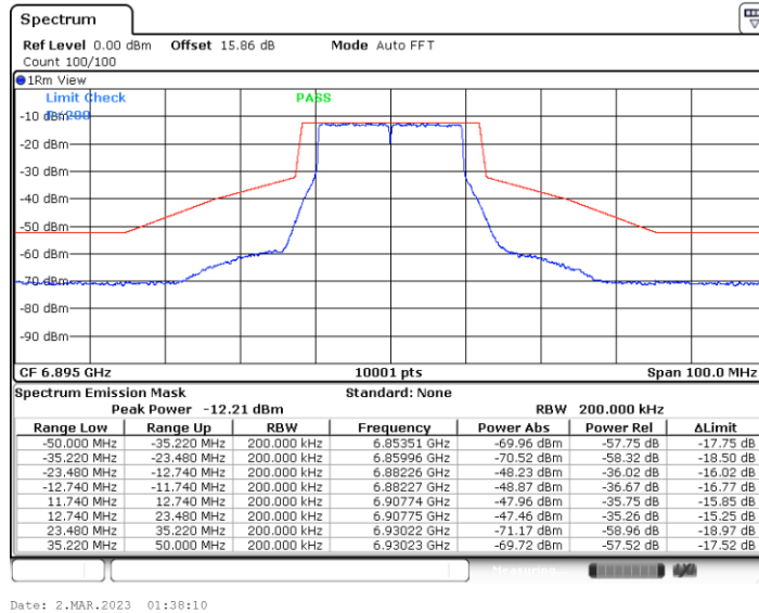
11BE20MIMO_Ant2_6895
