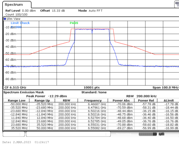
11BE20MIMO_Ant2_6515
