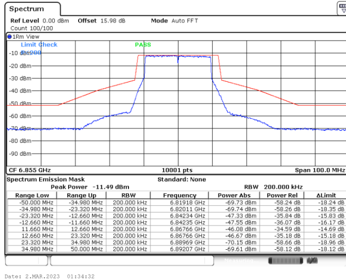
11BE20MIMO_Ant2_6855
