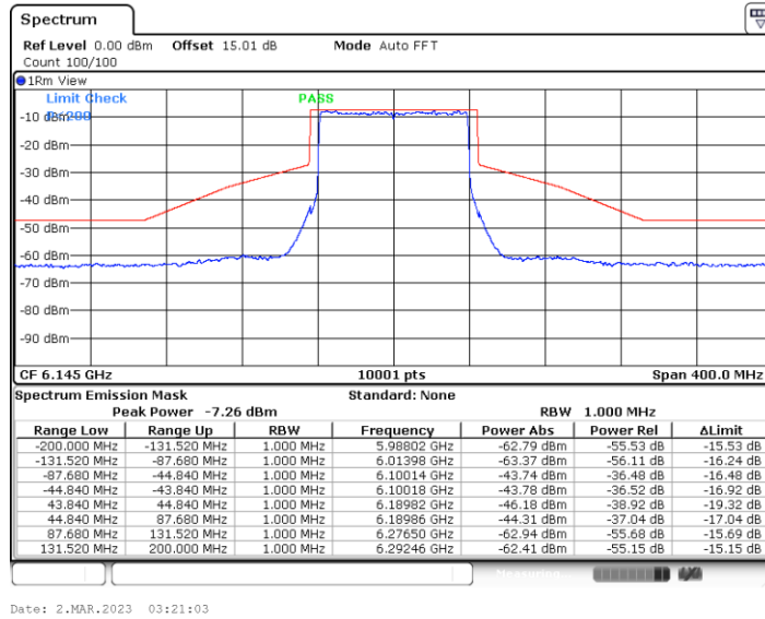
11BE80MIMO_Ant2_6145
