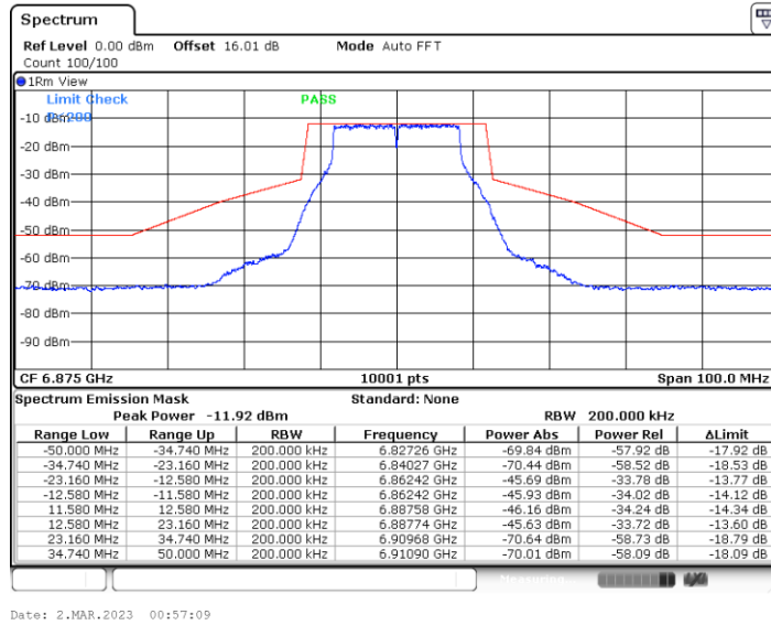
11A-CDD_Ant2_6875
