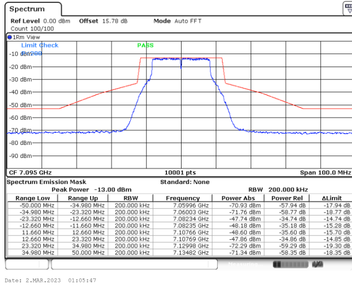
11A-CDD_Ant2_7095
