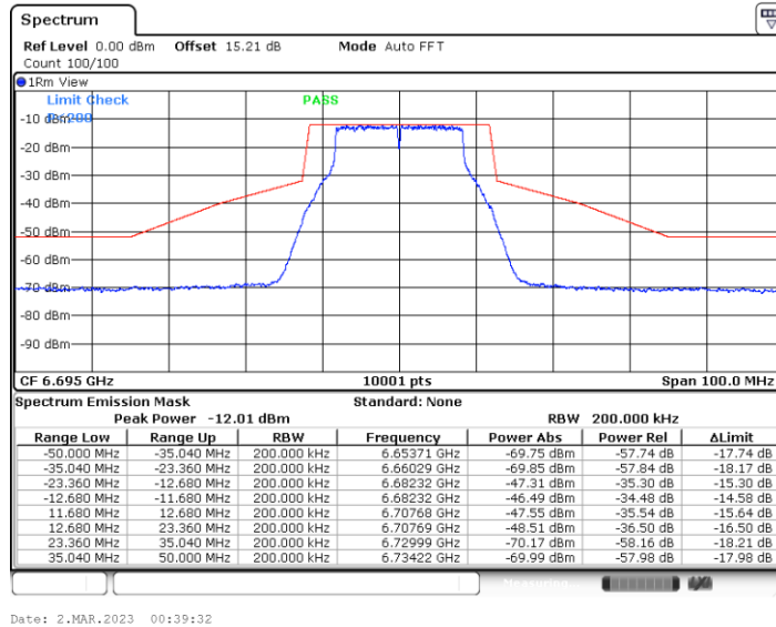
11A-CDD_Ant2_6695
