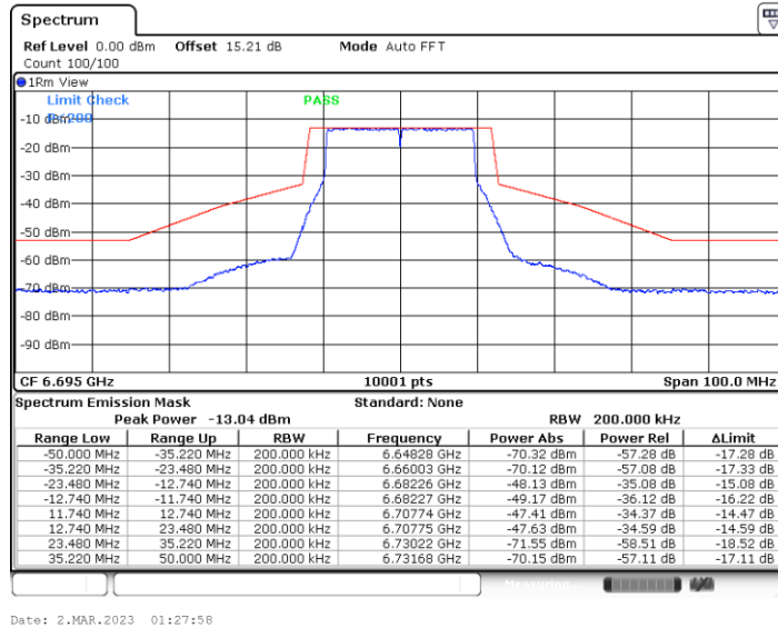
11BE20MIMO_Ant2_6695
