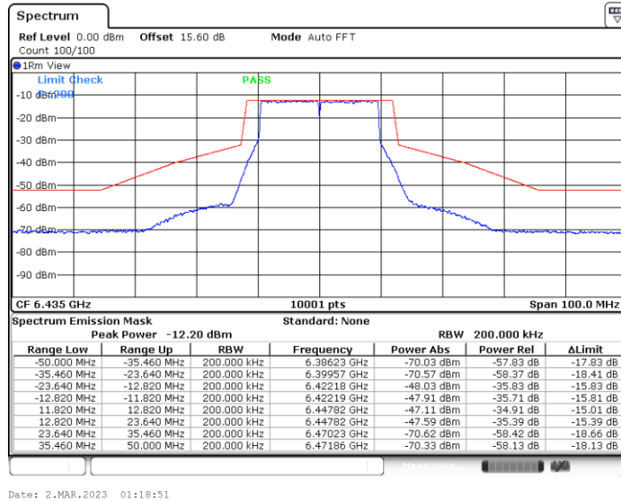
11BE20MIMO_Ant2_6435
