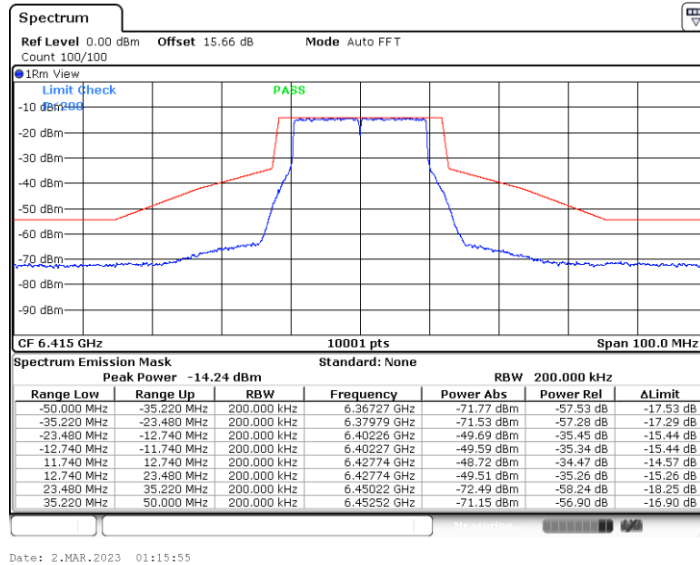
11BE20MIMO_Ant2_6415
