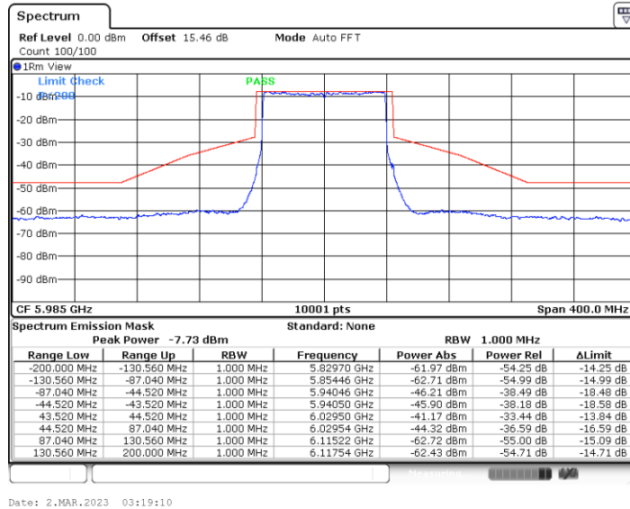
11BE80MIMO_Ant2_5985
