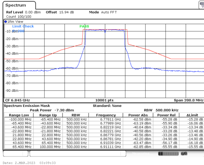
11BE40MIMO_Ant2_6845
