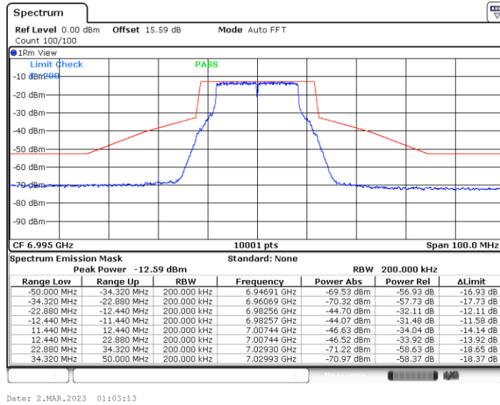
11A-CDD_Ant2_6995
