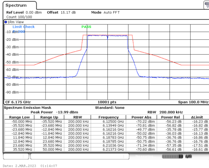
11BE20MIMO_Ant2_6175
