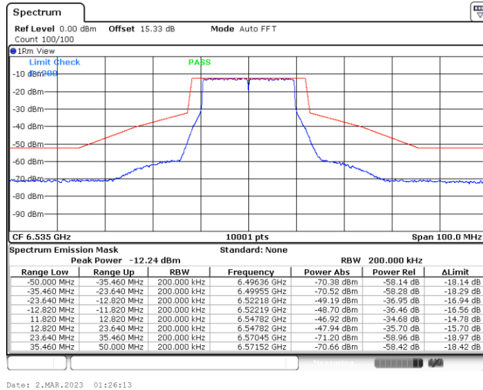
11BE20MIMO_Ant2_6535
