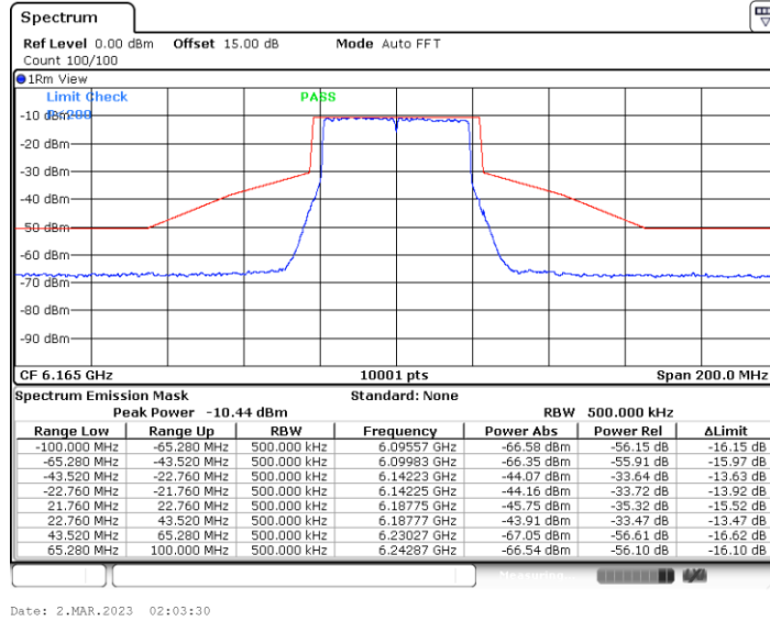
11BE40MIMO_Ant2_6165
