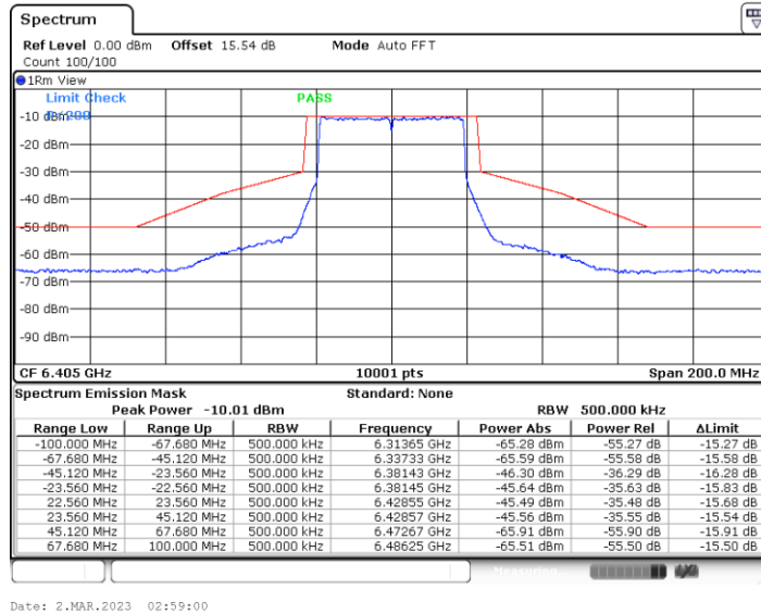
11BE40MIMO_Ant2_6405
