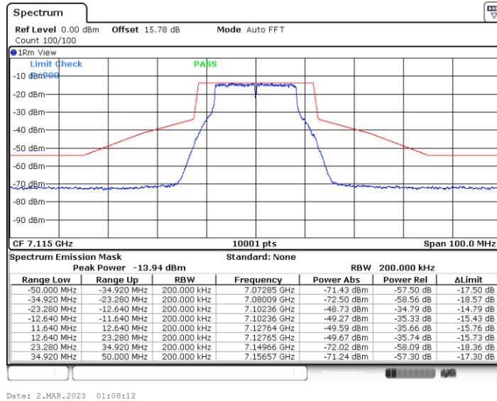
11A-CDD_Ant2_7115
