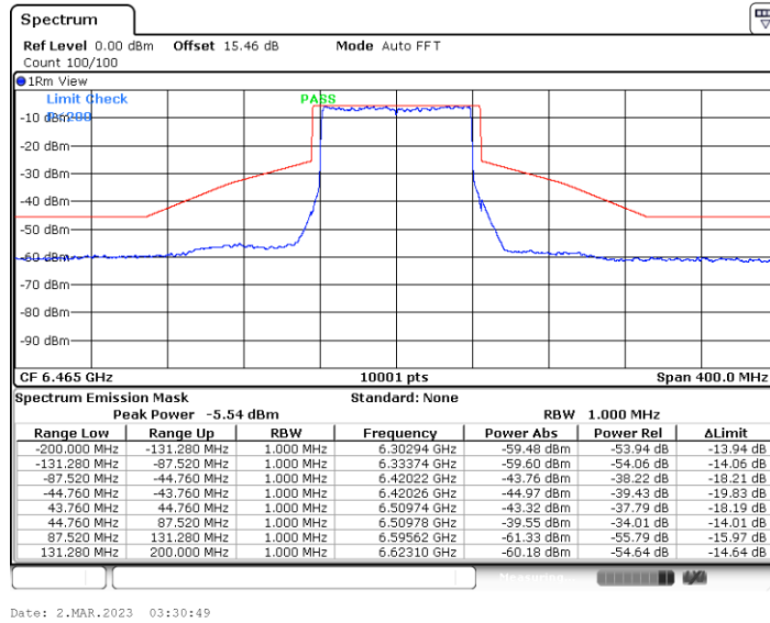
11BE80MIMO_Ant2_6465
