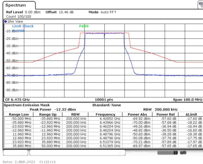
11BE20MIMO_Ant2_6475
