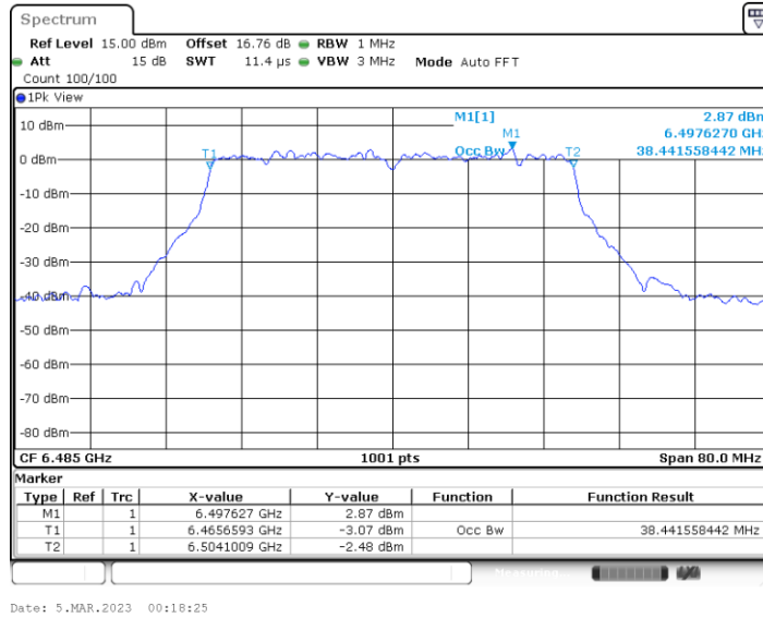
11BE40MIMO_Ant2_6485
