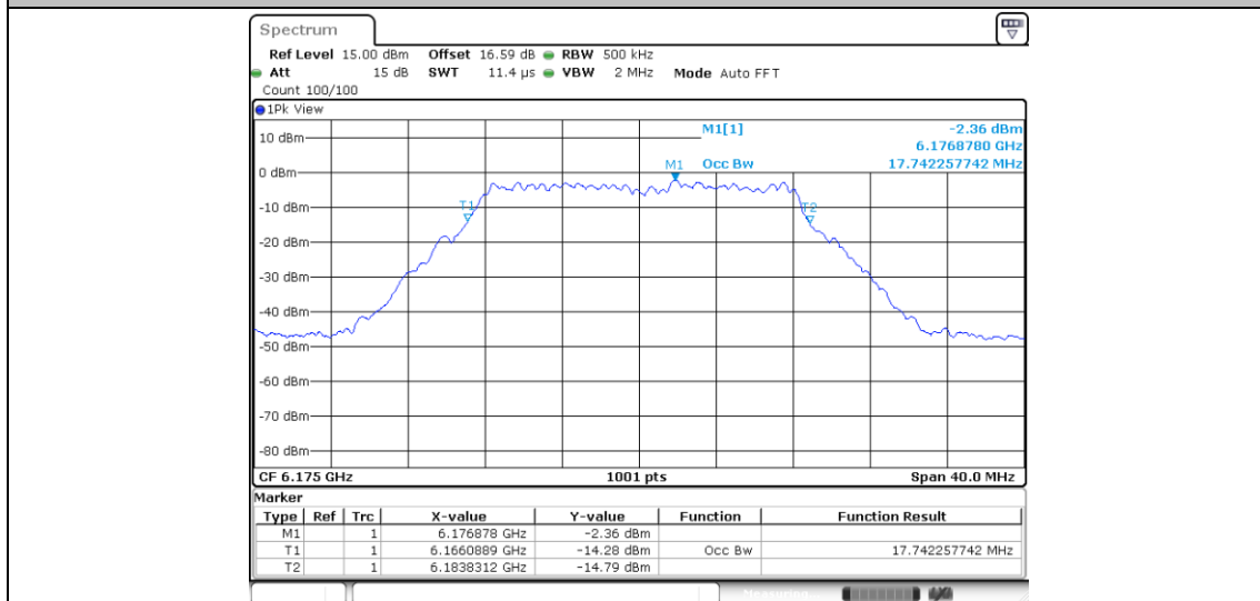
11A-CDD_Ant6_6175
