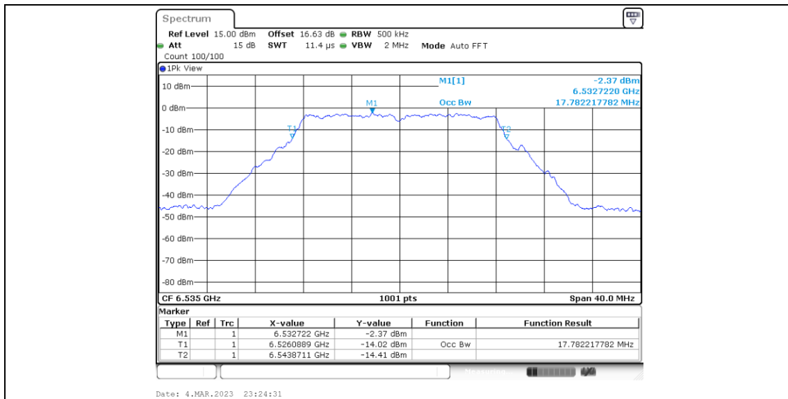
11A-CDD_Ant6_6535
