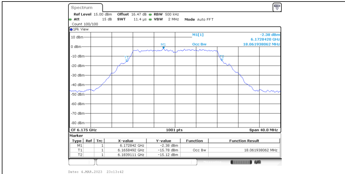
11A-CDD_Ant6_6175
