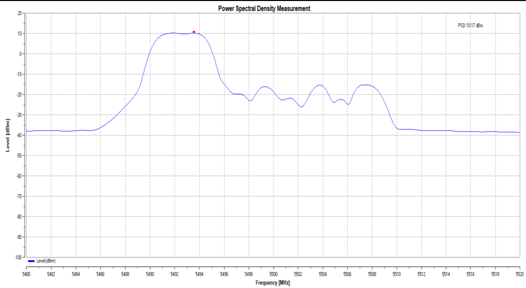
11BE20MIMO_total_5500_52Tone_RU37
