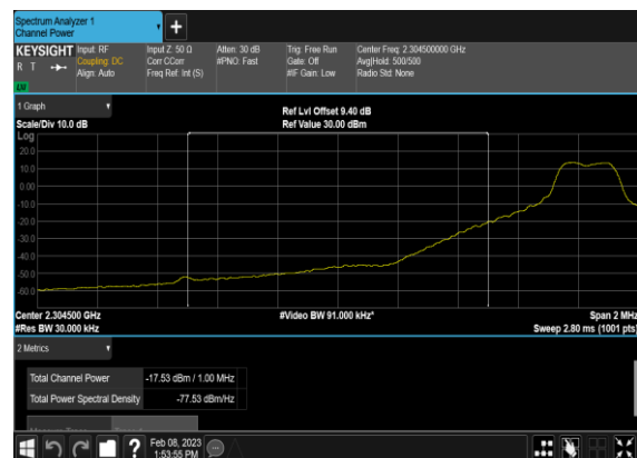
N30(5M)_DFT-s-OFDM_QPSK_Edge_1RB_Left_Low_ CH_CHP_PASS
