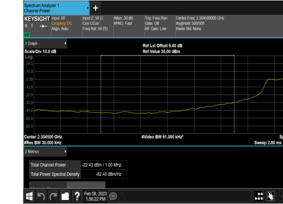
N30(5M)_DFT-s-OFDM_BPSK_Outer_Full_Low_CH_ CHP_PASS
