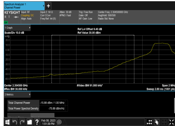
N30(5M)_DFT-s-OFDM_BPSK_Edge_1RB_Left_Low_ CH_CHP_PASS
