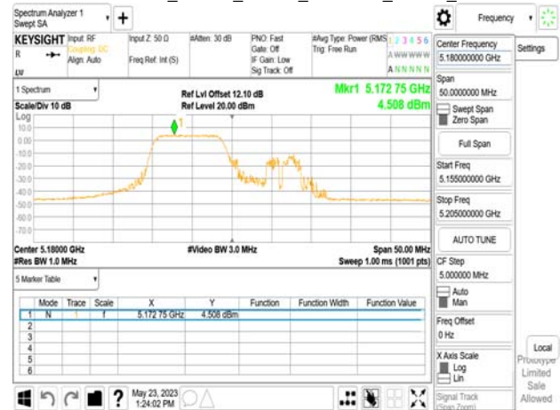
802.11be_20MHz_Chain0_5180MHz_RU26_0
