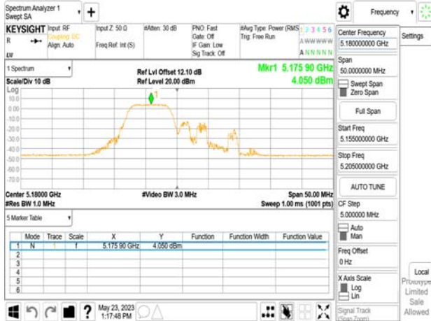
802.11be_20MHz_Chain0_5180MHz_52+26_MRU1
