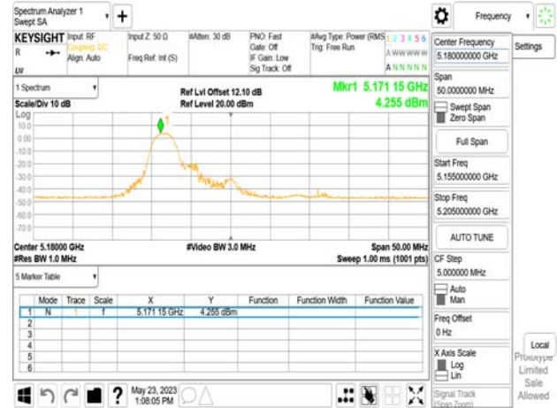
802.11be_20MHz_Chain0_5180MHz_RU52_37
