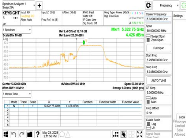
802.11be_20MHz_Chain0_5320MHz_RU26_8
