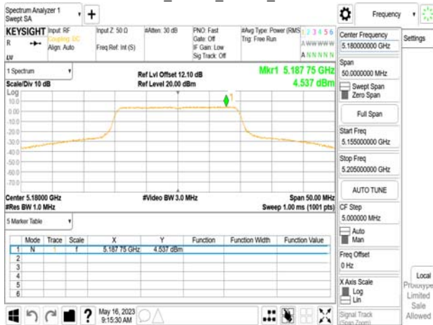
802.11be_20MHz_Chain1_5180MHz
