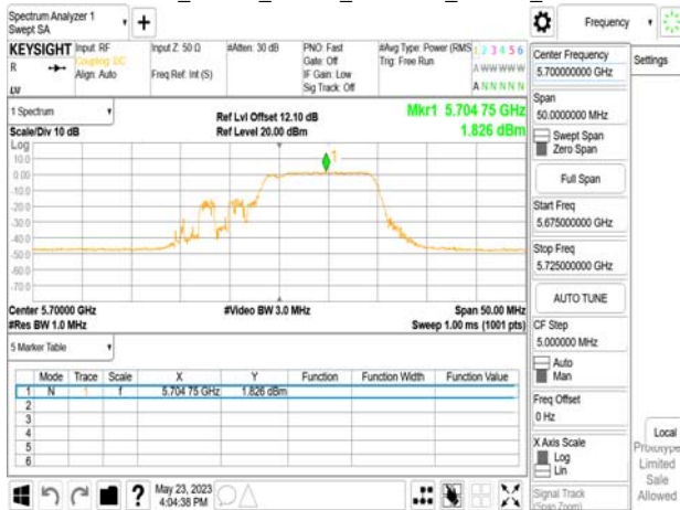
802.11be_20MHz_Chain0_5700MHz_52+26_MRU3
