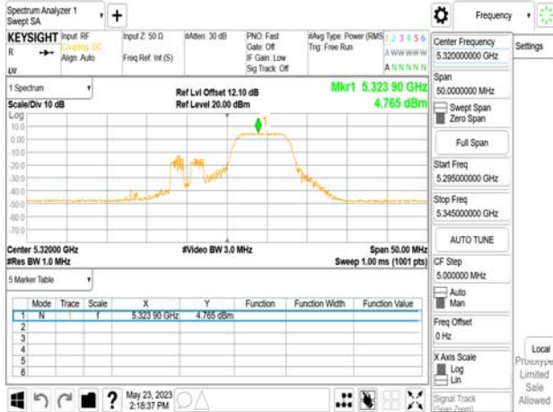
802.11be_20MHz_Chain1_5320MHz_52+26_MRU3
