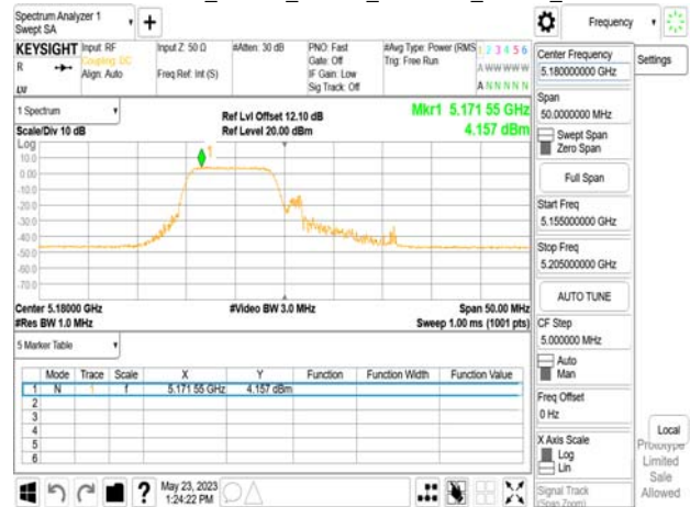
802.11be_20MHz_Chain1_5180MHz_RU106_53
