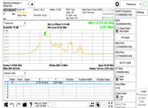
802.11be_20MHz_Chain0_5745MHz_RU26_0
