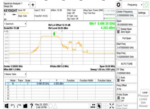
802.11be_20MHz_Chain1_5500MHz_RU26_0
