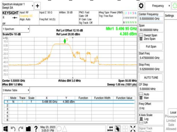
802.11be_20MHz_Chain0_5500MHz_RU106_53
