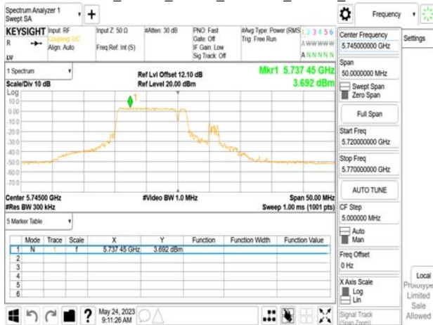
802.11be_20MHz_Chain0_5745MHz_106+26_MRUI
