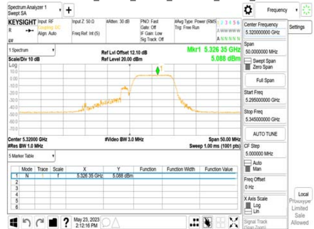
802.11be_20MHz_Chain1_5320MHz_RU26_8
