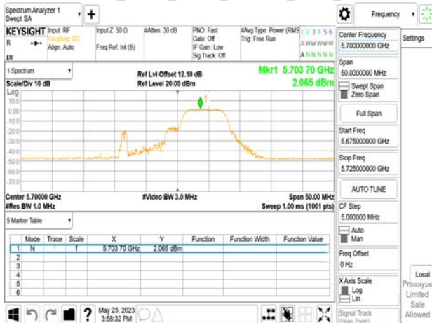
802.11be_20MHz_Chain0_5700MHz_RU106_54
