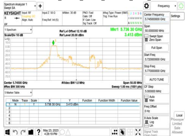
802.11be_20MHz_Chain0_5745MHz_RU26_0
