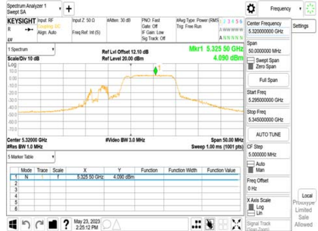
802.11be_20MHz_Chain0_5320MHz_106+26_MRU2
