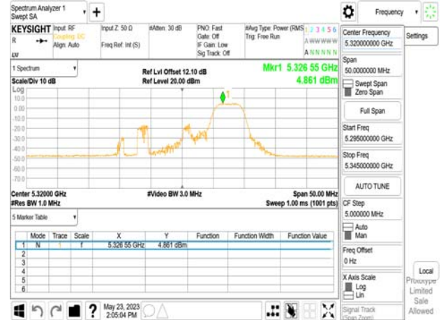
802.11be_20MHz_Chain1_5320MHz_RU52_40
