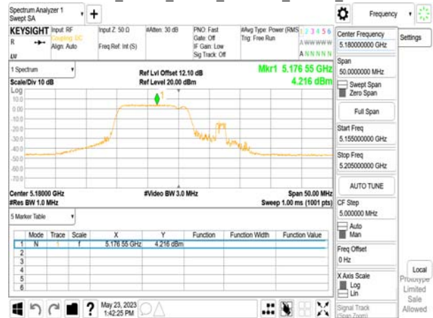
802.11be_20MHz_Chain1_5180MHz_52+26_MRUI
