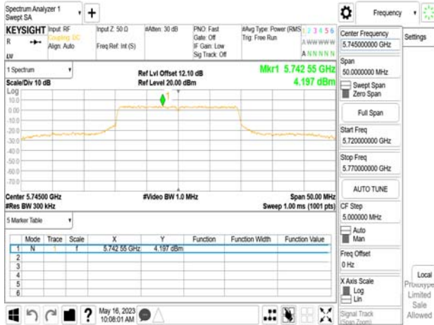
802.11be_20MHz_Chain0_5745MHz_106+26_MRUI
