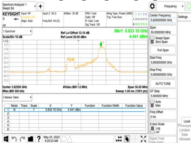
802.11be_20MHz_Chain0_5825MHz_RU52_40
