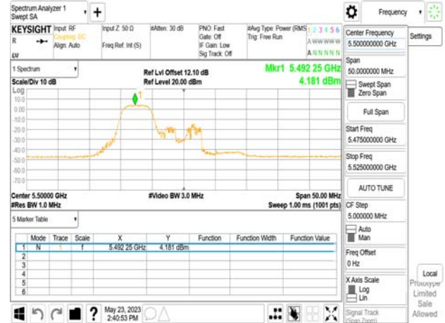
802.11be_20MHz_Chain1_5500MHz_RU52_37
