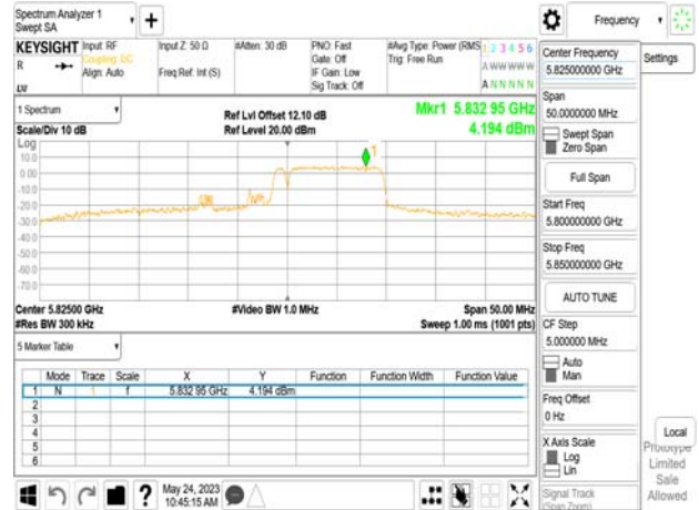
802.11be_20MHz_Chain0_5825MHz_52+26_MRU3
