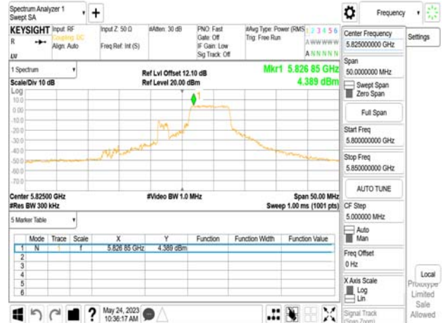
802.11be_20MHz_Chain0_5825MHz_RU106_54
