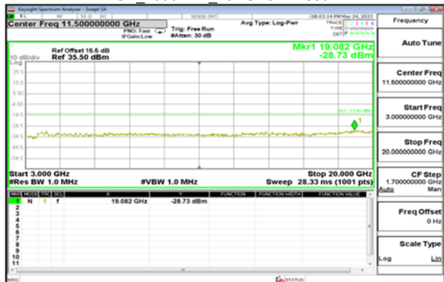
EDGE 1900MHz_MidCH661-1880
