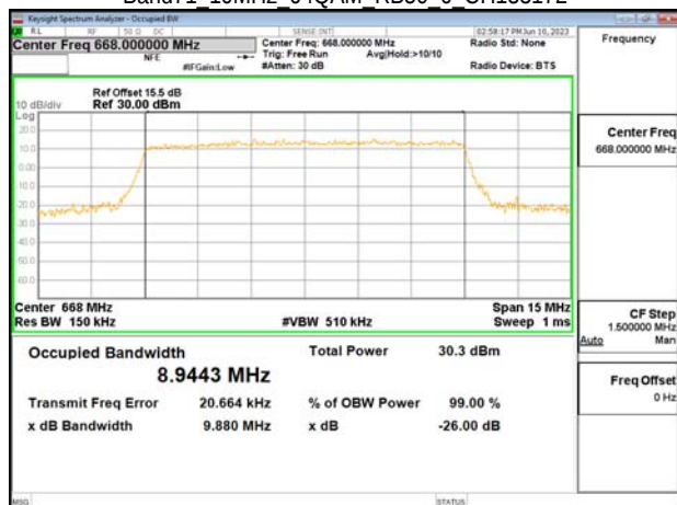
Band71 10MHz 64QAM RB50 0 CH133172
