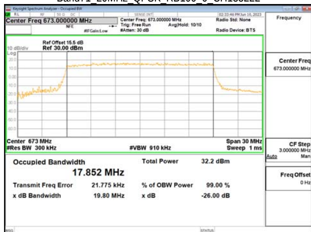
Band71 20MHz QPSK RB100 0 CH133222
