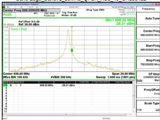
Band Edge Band71 10MHz QPSK RB1 49 CH133422
