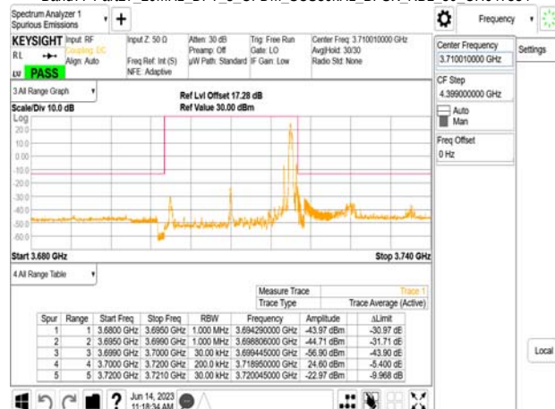
Band77-Part27_20MHz_DFT_s_OFDM_SCS30kHz_BPSK_RB1_50_CH647334
