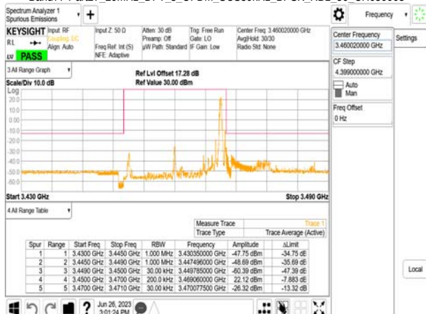
Band77-Part27_20MHz_DFT_s_OFDM_SCS30kHz_BPSK_RB1_50_CH630668
