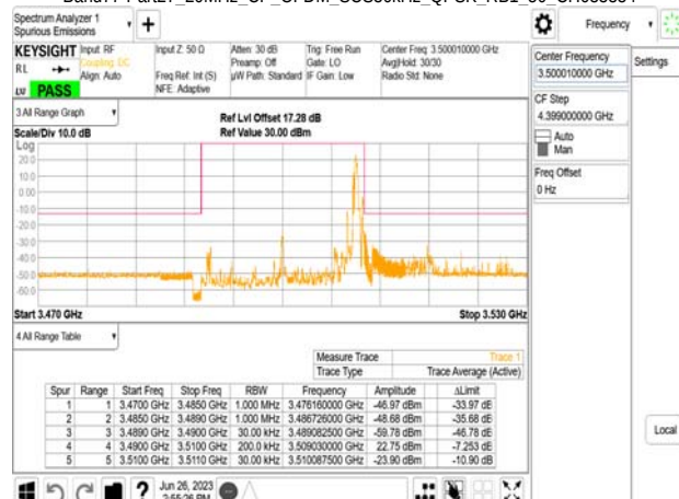
Band77-Part27_20MHz_CP_OFDM_SCS30kHz_QPSK_RB1_50_CH636000
