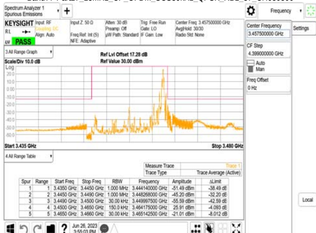
Band77-Part27_15MHz_CP_OFDM_SCS30kHz_QPSK_RB1_37_CH630500
