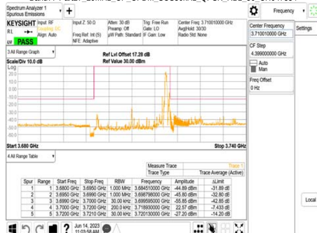
Band77-Part27_20MHz_CP_OFDM_SCS30kHz_QPSK_RB1_50_CH647334
