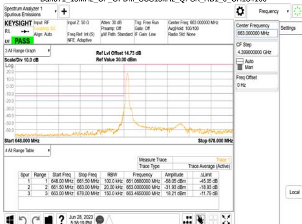
Band71_15MHz_CP_OFDM_SCS15kHz_QPSK_RB1_0_CH134100
