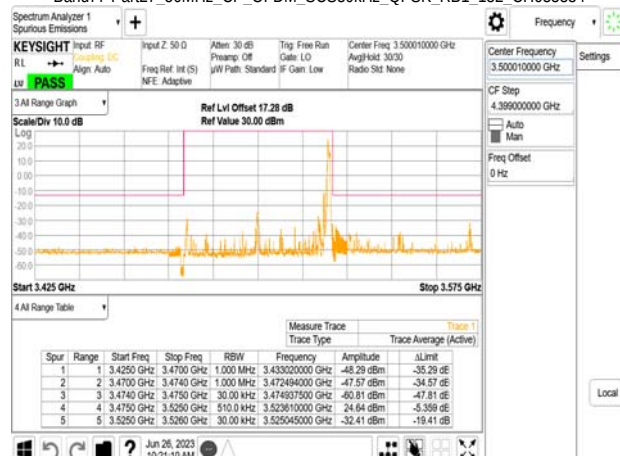
Band77-Part27_50MHz_CP_OFDM_SCS30kHz_QPSK_RB1_132_CH635000
