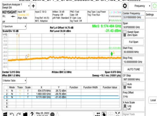
Band5_15MHz_DFT_s_OFDM_SCS15kHz_BPSK_RB1_1_CH168300
