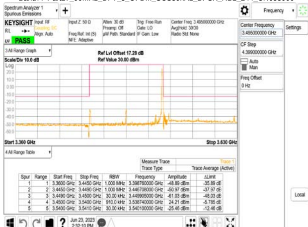
Band77-Part27_90MHz_DFT_s_OFDM_SCS30kHz_BPSK_RB1_244_CH633000
