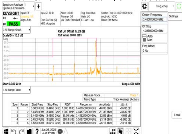
Band77-Part27_70MHz_CP_OFDM_SCS30kHz_QPSK_RB1_188_CH632334
