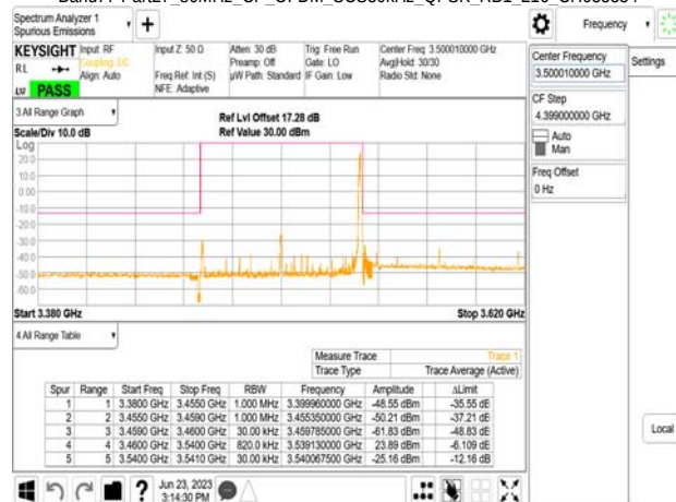
Band77-Part27_80MHz_CP_OFDM_SCS30kHz_QPSK_RB1_216_CH634000
