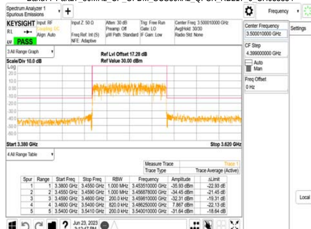
Band77-Part27_80MHz_CP_OFDM_SCS30kHz_QPSK_RB217_0_CH634000
