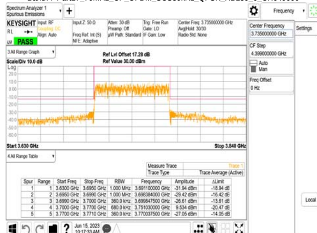
Band77-Part27_70MHz_CP_OFDM_SCS30kHz_QPSK_RB189_0_CH649000
