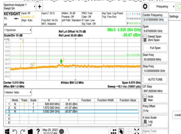
Band5_20MHz_DFT_s_OFDM_SCS15kHz_BPSK_RB1_1_CH16800
