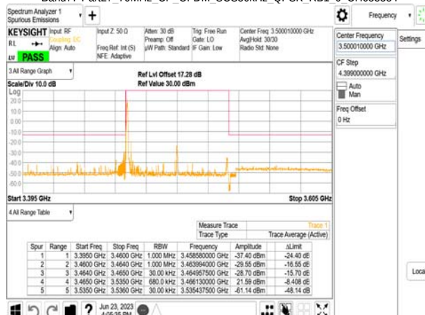
Band77-Part27_70MHz_CP_OFDM_SCS30kHz_QPSK_RB1_0_CH634332
