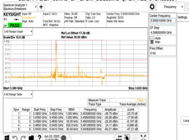
Band77-Part27_80MHz_CP_OFDM_SCS30kHz_QPSK_RB1_0_CH634000
