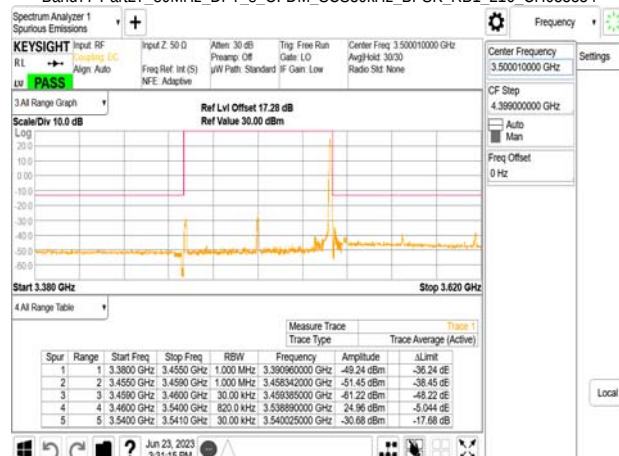
Band77-Part27_80MHz_DFT_s_OFDM_SCS30kHz_BPSK_RB1_216_CH634000
