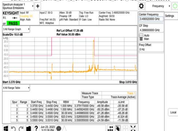
Band77-Part27_80MHz_DFT_s_OFDM_SCS30kHz_BPSK_RB1_216_CH632668
