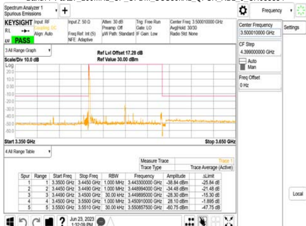
Band77-Part27_100MHz_CP_OFDM_SCS30kHz_QPSK_RB1_0_CH633334
