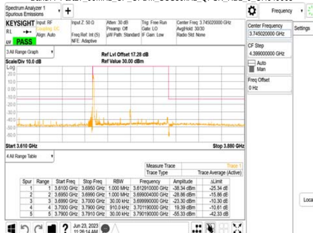
Band77-Part27_90MHz_CP_OFDM_SCS30kHz_QPSK_RB1_0_CH649668
