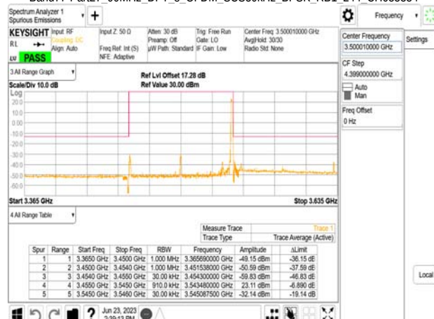
Band77-Part27_90MHz_DFT_s_OFDM_SCS30kHz_BPSK_RB1_244_CH633666
