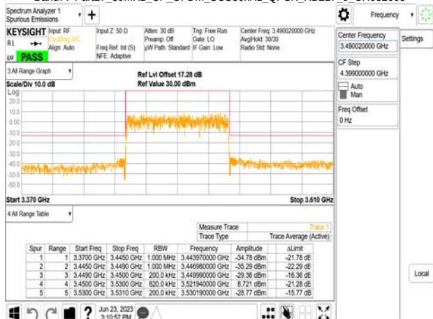
Band77-Part27_80MHz_CP_OFDM_SCS30kHz_QPSK_RB217_0_CH632668
