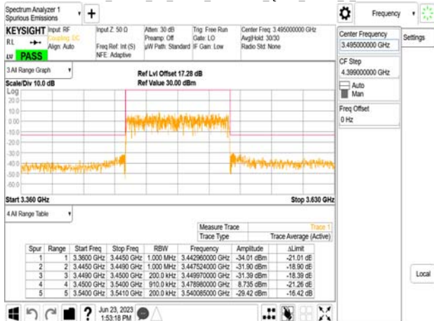
Band77-Part27_90MHz_CP_OFDM_SCS30kHz_QPSK_RB245_0_CH633000
