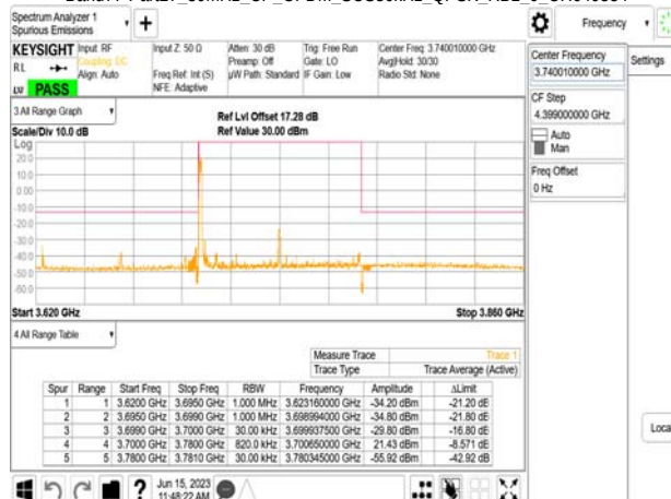
Band77-Part27_80MHz_CP_OFDM_SCS30kHz_QPSK_RB1_0_CH649334
