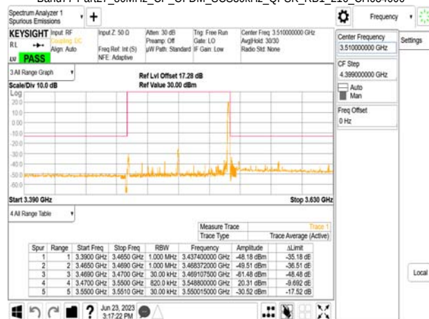
Band77-Part27_80MHz_CP_OFDM_SCS30kHz_QPSK_RB1_216_CH649334
