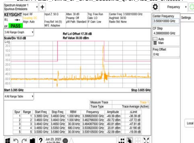
Band77-Part27_70MHz_CP_OFDM_SCS30kHz_QPSK_RB1_188_CH634332
