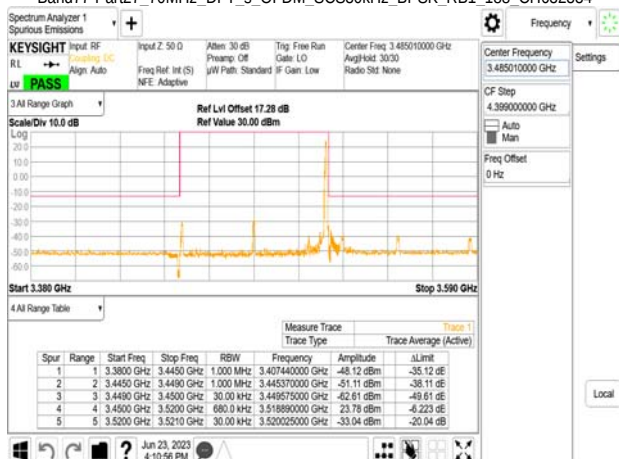
Band77-Part27_70MHz_DFT_s_OFDM_SCS30kHz_BPSK_RB1_188_CH632334
