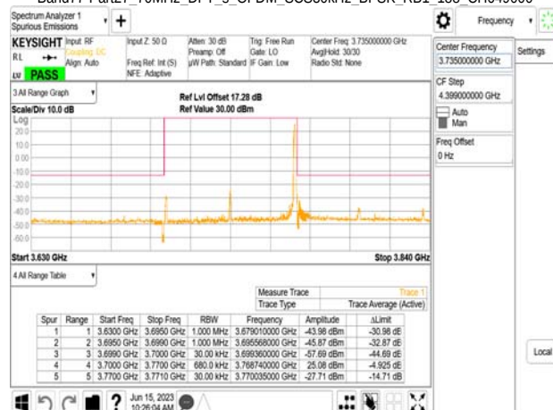
Band77-Part27_70MHz_DFT_s_OFDM_SCS30kHz_BPSK_RB1_188_CH649000
