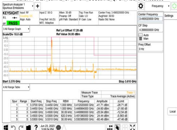
Band77-Part27_80MHz_CP_OFDM_SCS30kHz_QPSK_RB1_0_CH632668
