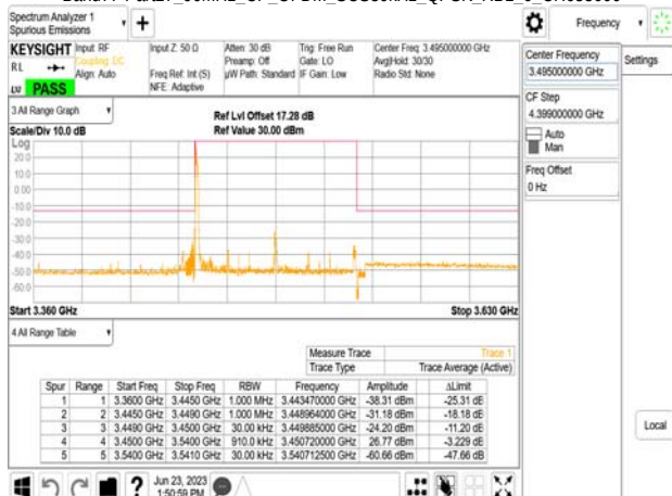
Band77-Part27_90MHz_CP_OFDM_SCS30kHz_QPSK_RB1_0_CH633000
