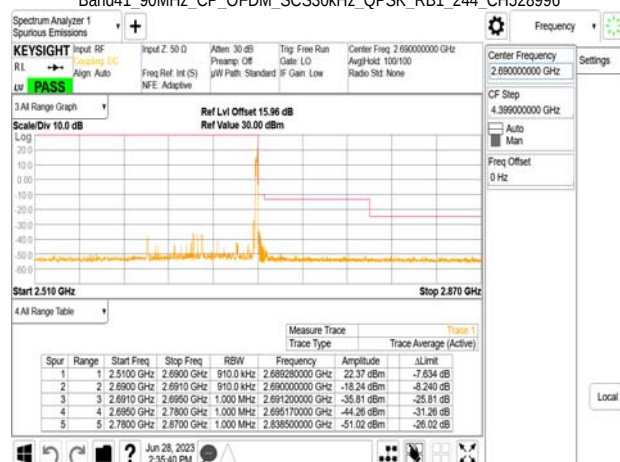
Band41_90MHz_CP_OFDM_SCS30kHz_QPSK_RB1_244_CH528996
