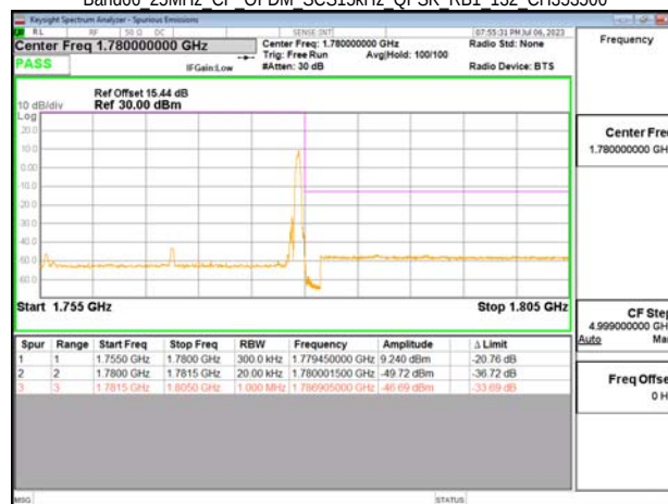
Band66 25MHz CP OFDM SCS15kHz QPSK RB1 132 CH353500
