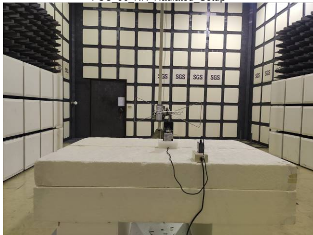
FCC 15 407 WLAN 6E Normal CBP Setup
