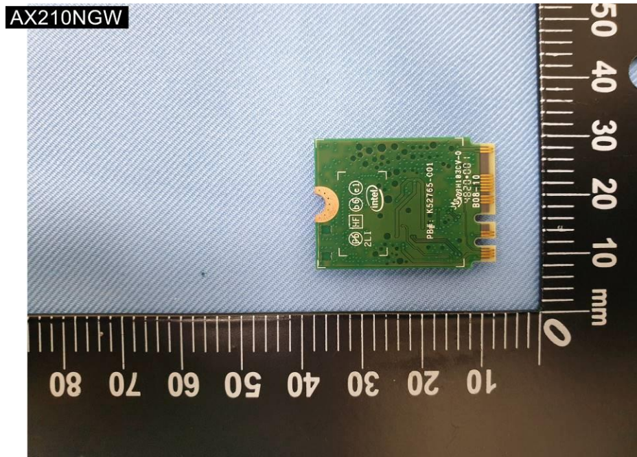
EUT Photo (4)
