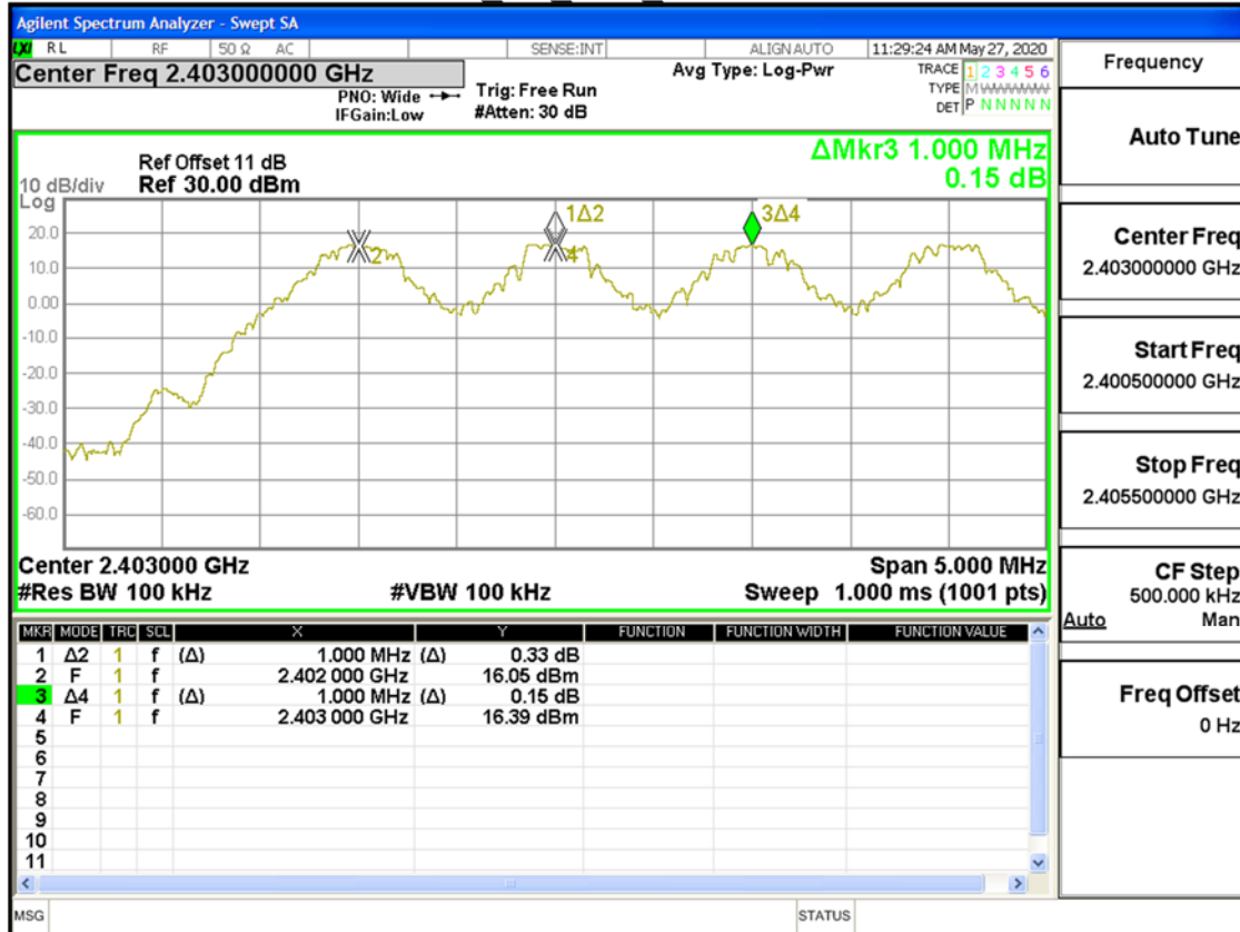
GFSK 1M DH5 CH0CH1CH2
