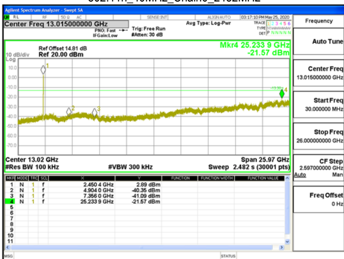
802.11n_40MHz_Chain0_2452MHz
