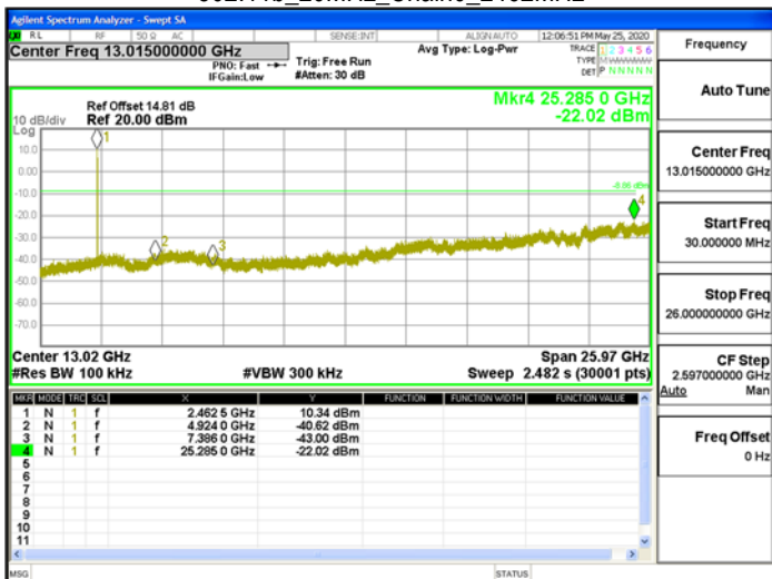
802.11b_20MHz_Chain0_2462MHz
