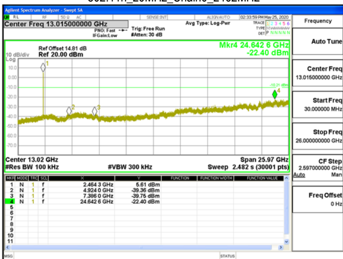
802.11n_20MHz_Chain0_2462MHz
