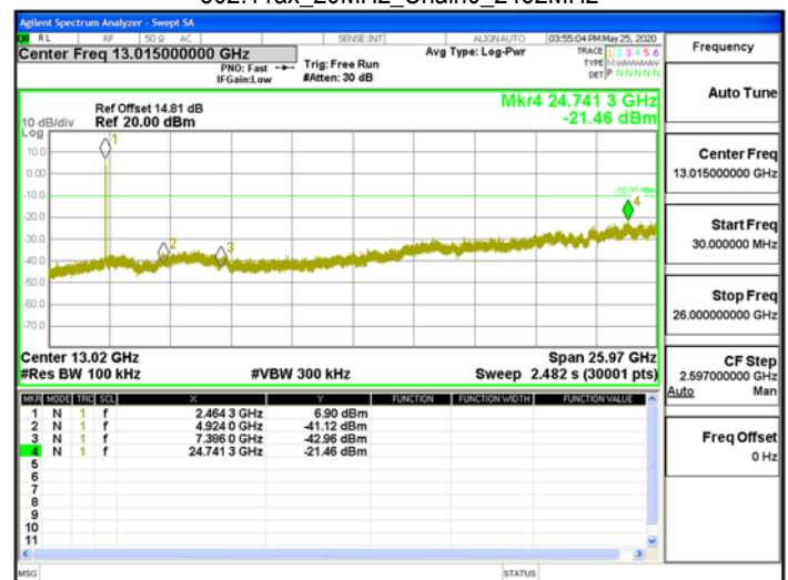
802.11ax_20MHz_Chain0_2462MHz
