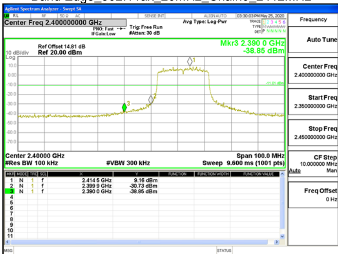
Band Edge 802.11ax 20MHz Chain0 2412MHz
