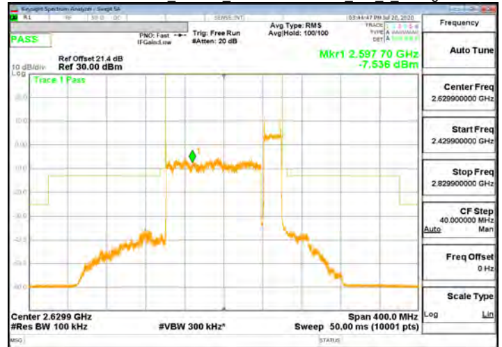
CP-OFDM Band41 20+40MHz\QPSK 1 0 CHLow
