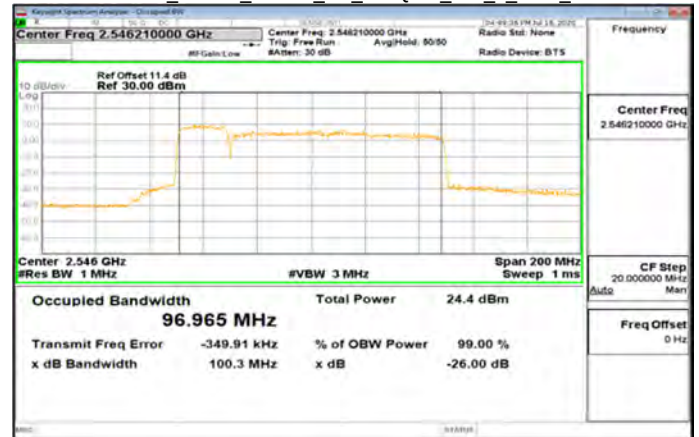
Band41 20MHz 80MHz CP 256QAM 217 0 Main Mid
