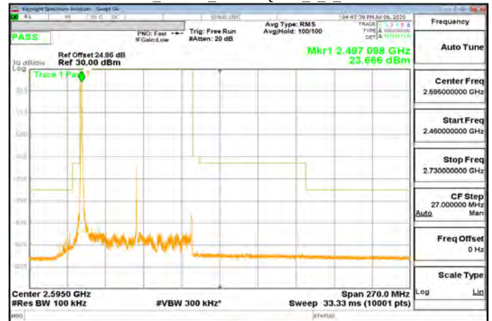
CP-OFDM_Band41_80MHz\QPSK_1_0_CH507204
