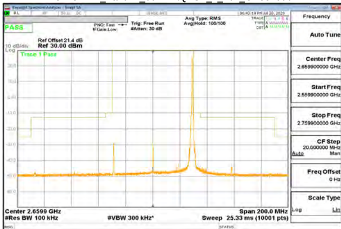
CP-OFDM_Band41_60MHz\QPSK_1_161_CH531996
