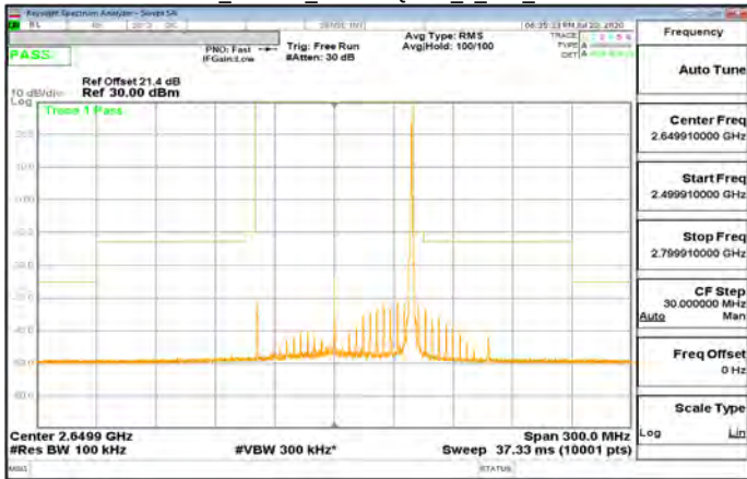
CP-OFDM_Band41_80MHz\QPSK_1_216_CH529998
