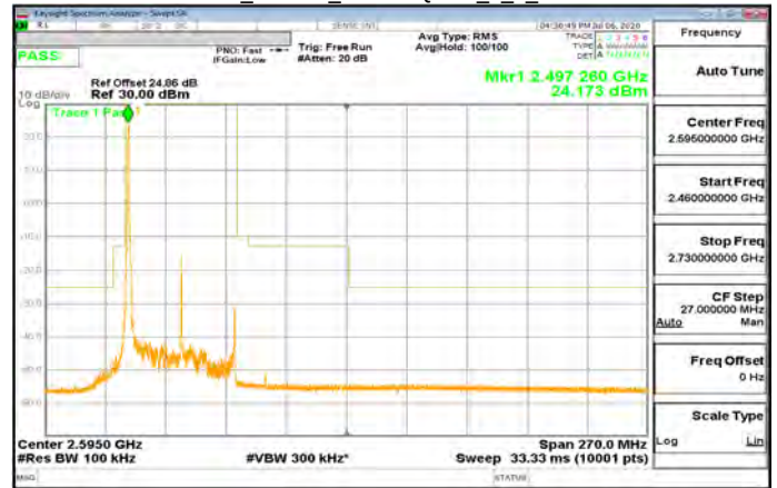
CP-OFDM_Band41_50MHz\QPSK_1_0_CH504204
