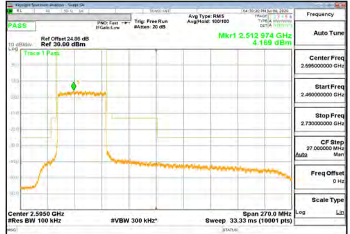
CP-OFDM_Band41_50MHz\QPSK_133_0_CH504204
