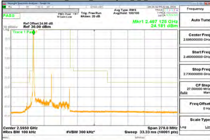
CP-OFDM_Band41_60MHz\QPSK_1_0_CH505200
