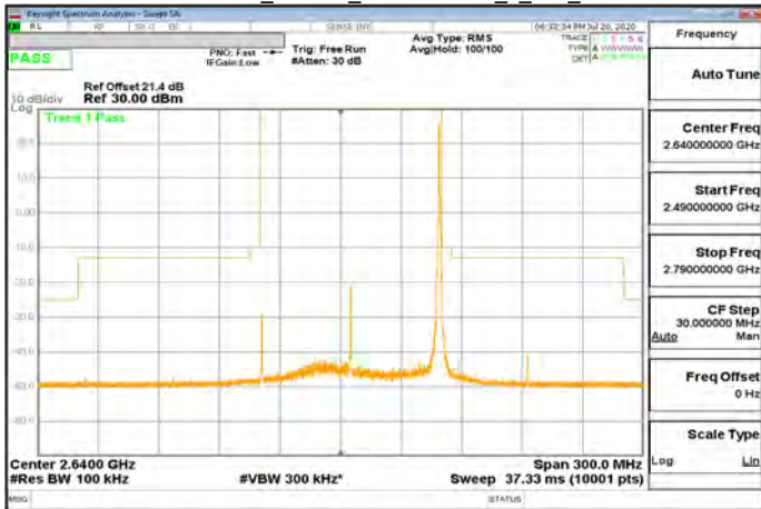
DFT-s-OFDM Pi/2_Band41_90MHz\BPSK_1_244_CH528996
