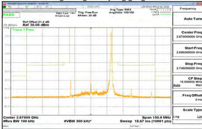
CP-OFDM_Band41_40MHz\QPSK_1_105_CH534000
