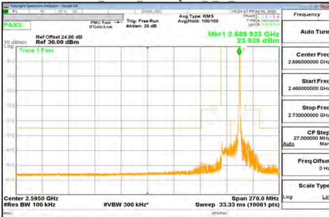
CP-OFDM_Band41_20MHz\QPSK_1_50_CH535998
