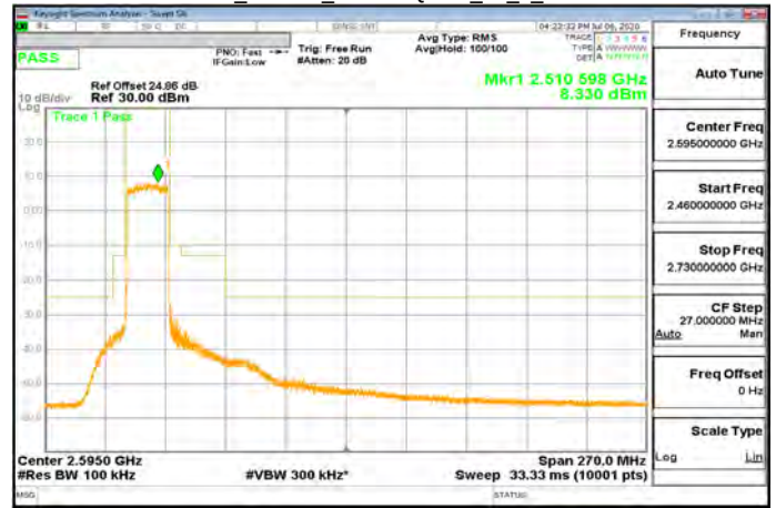
CP-OFDM_Band41_20MHz\QPSK_51_0_CH501204
