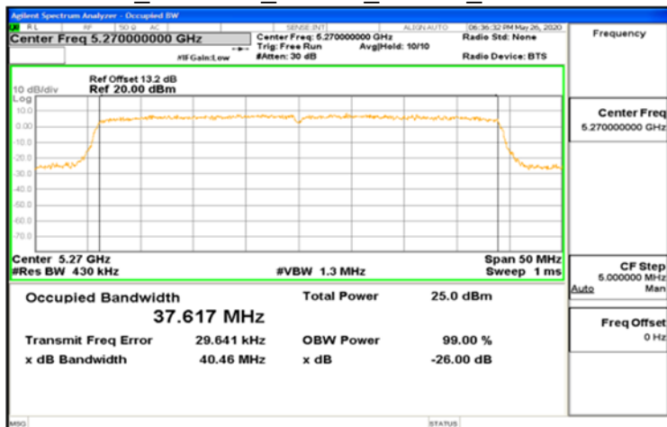
FCC_802.11ax_40MHz_Chain1_5270MHz
