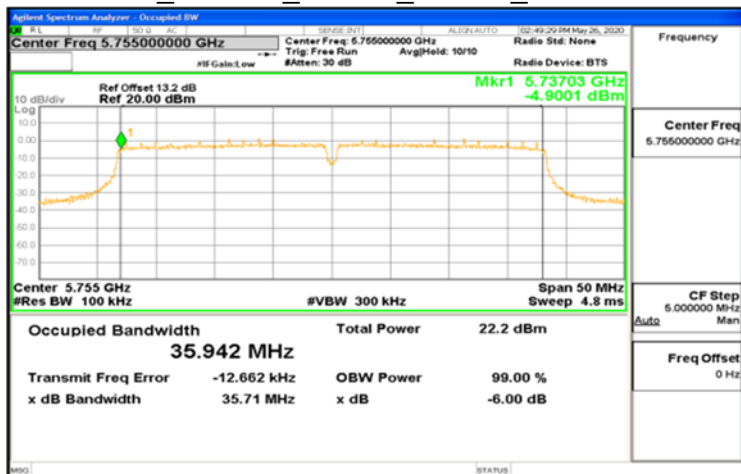
FCC_802.11n_40MHz_Chain0_5755MHz
