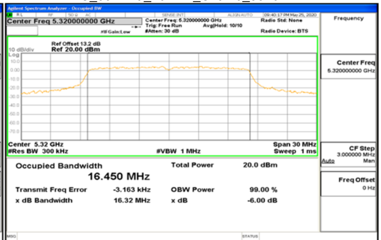
IC_802.11a_20MHz_Chain0_5320MHz
