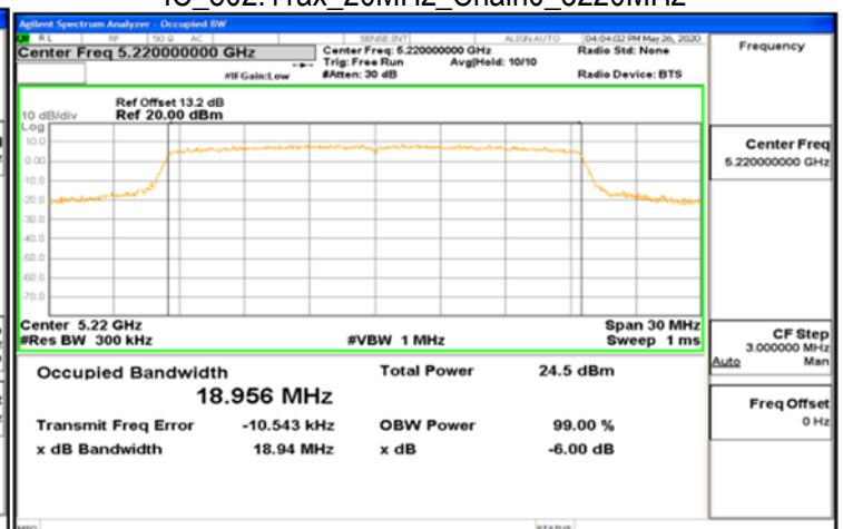
IC_802.11ax_20MHz_Chain0_5220MHz
