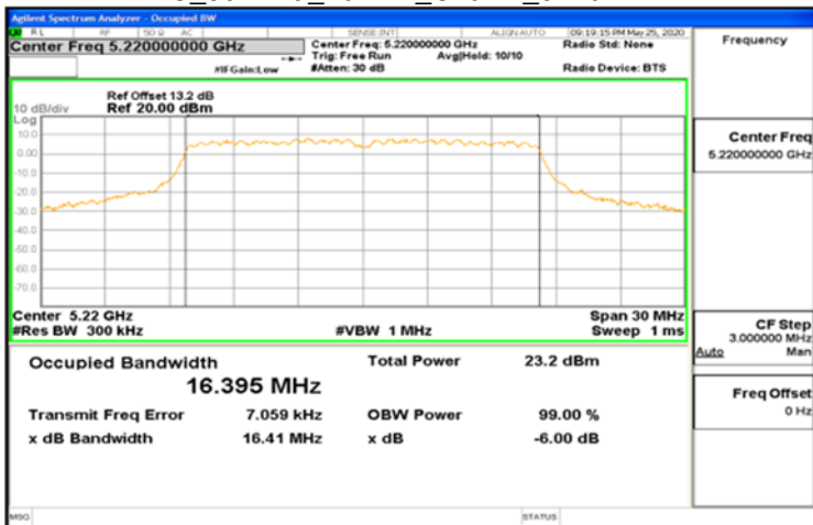
IC_802.11a_20MHz_Chain1_5220MHz
