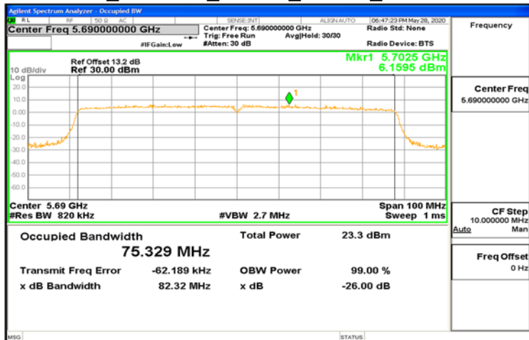
FCC_802.11ac_80MHz_Chain1_5690MHz
