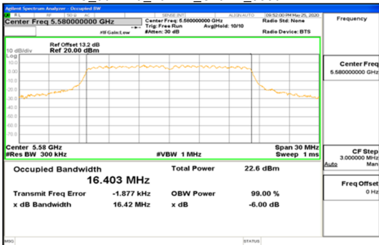
IC_802.11a_20MHz_Chain1_5580MHz
