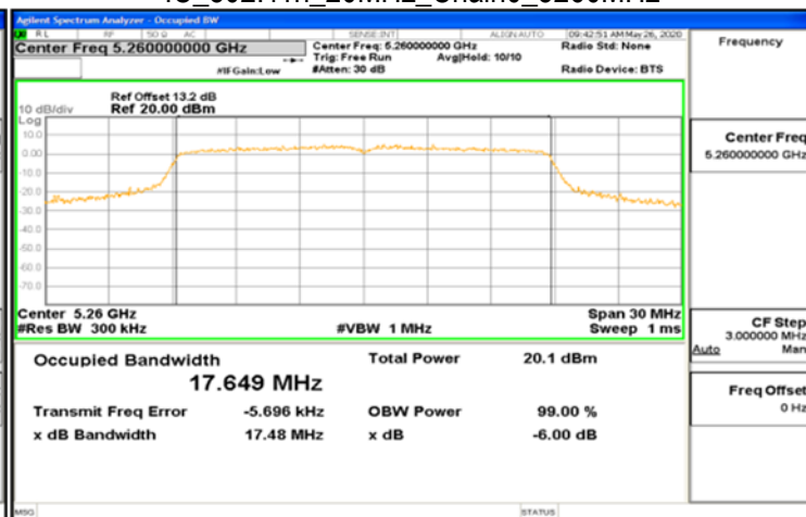
IC_802.11n_20MHz_Chain0_5260MHz
