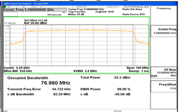
FCC_802.11ax_80MHz_Chain1_5290MHz
