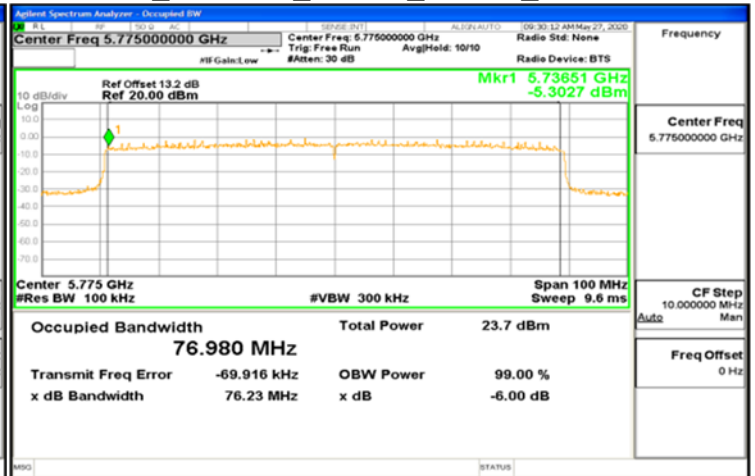
FCC_802.11ax_80MHz_Chain1_5775MHz
