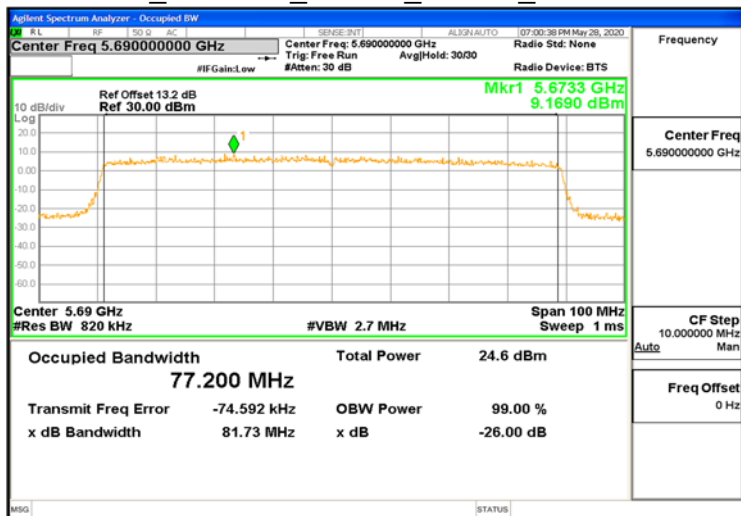
FCC_802.11ax_80MHz_Chain1_5690MHz
