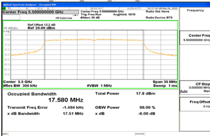
IC_802.11n_20MHz_Chain0_5500MHz
