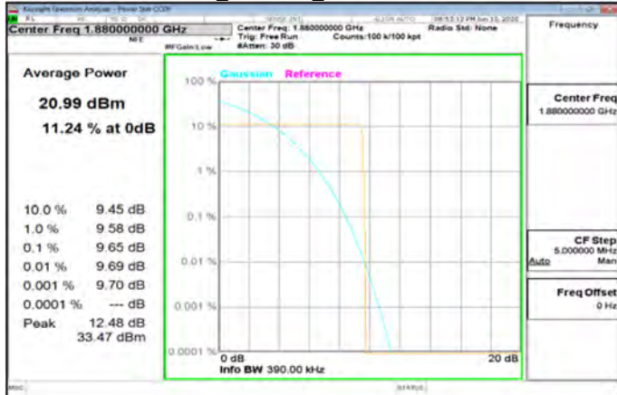
GPRS_1900MHz_MidCH661-1880
