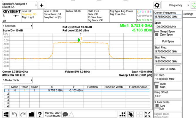
802.11ax_40MHz_Chain0_5755MHz_RU242_61
