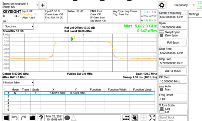
802.11ax_40MHz_Chain1_5670MHz
