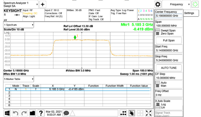
802.11ax_40MHz_Chain1_5190MHz
