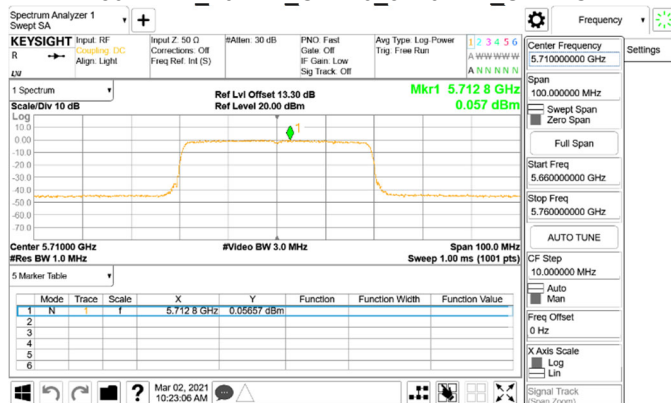
802.11ax_40MHz_Chain0_5710MHz_UNI2_C2
