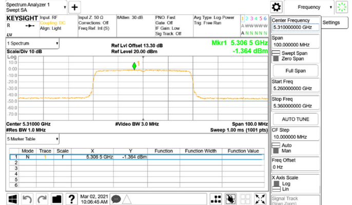
802.11ax_40MHz_Chain1_5310MHz_RU242_62
