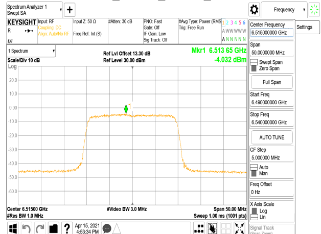
802.11ax_20MHz_Chain1_6515MHz_RU106_54
