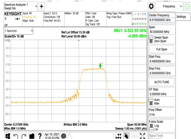
802.11ax_20MHz_Chain1_6515MHz_RU26_8
