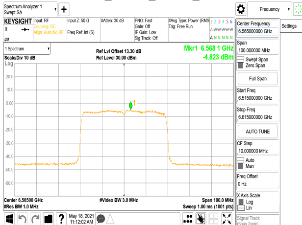
802.11ax_40MHz_Chain0_6565MHz_RU242_61
