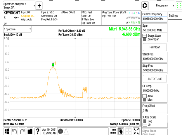
802.11ax_20MHz_Chain1_5955MHz_RU52_37
