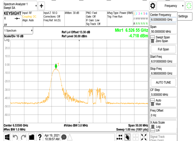
802.11ax_20MHz_Chain1_6535MHz_RU52_37
