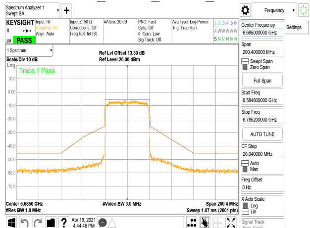
802.11ax_40MHz_Chain1_6685MHz
