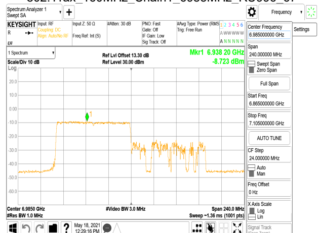
802.11ax_160MHz_Chain1_6985MHz_RU996_S67
