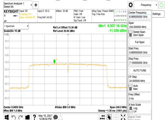
802.11ax_160MHz_Chain1_6985MHz_RU996_67
