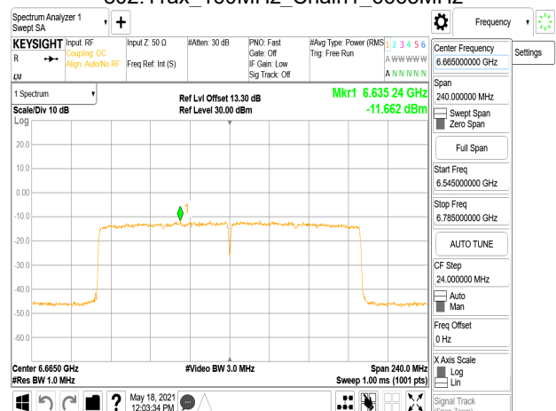
802.11ax_160MHz_Chain1_6665MHz
