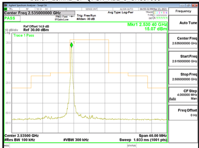
Band7 10MHz CP-QPSK RB1_0 CH507000
