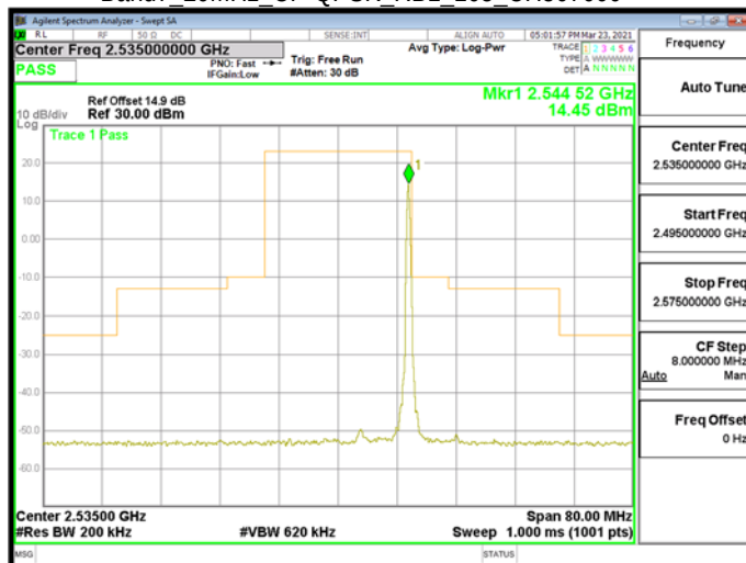
Band7 20MHz CP-QPSK RB1_105 CH507000
