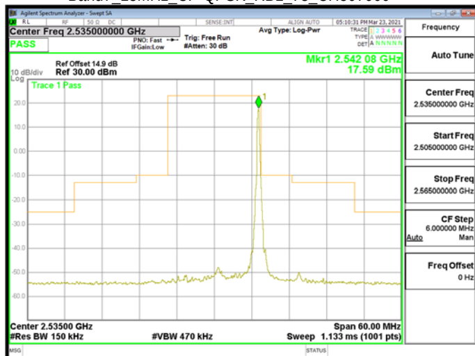
Band7_15MHz_CP-QPSK_RB1_78_CH507000
