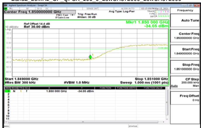
Band2 20MHz CP QPSK 106 0_LowCH372000_LowCH372000
