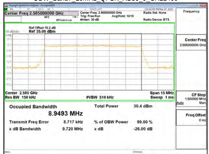
OBW Band7 10MHz QPSK_RB50_0_CH21400
