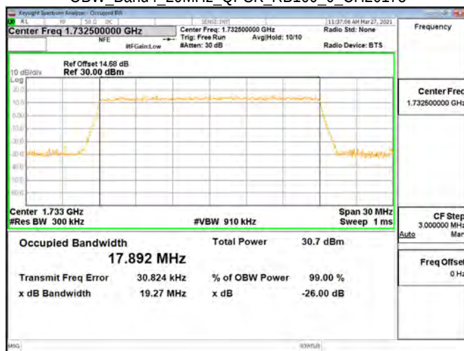
OBW Band4 20MHz QPSK RB100 0 CH20300
