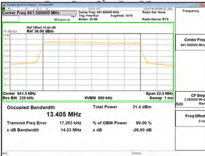
OBW_Band26_15MHz_QPSK_RB75_0_CH26965
