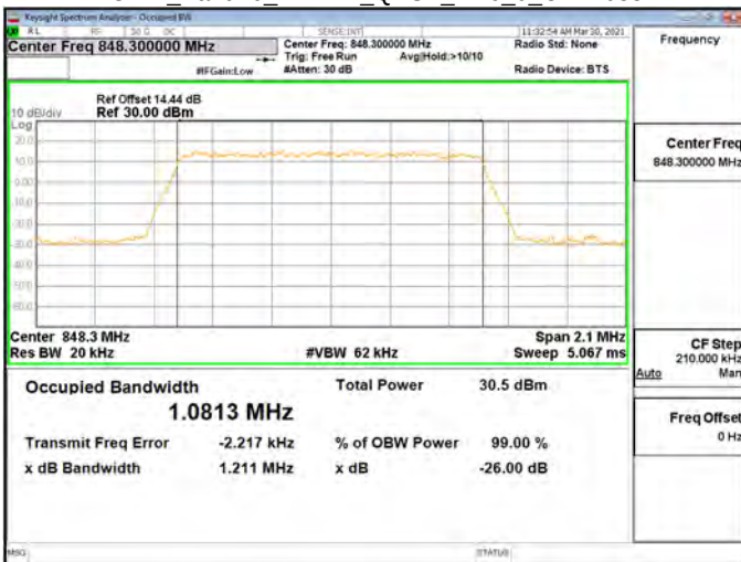
OBW_Band26_1.4MHz_QPSK_RB6_0_CH27033
