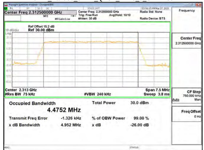
OBW_Band30_5MHz_QPSK_RB25_0_CH27735
