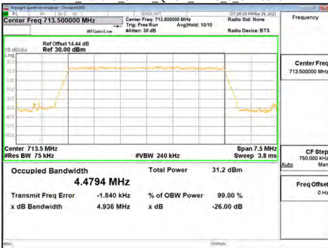
OBW_Band17_5MHz_QPSK_RB25_0_CH23825
