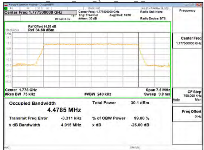
OBW_Band66_5MHz_QPSK_RB25_0_CH132647
