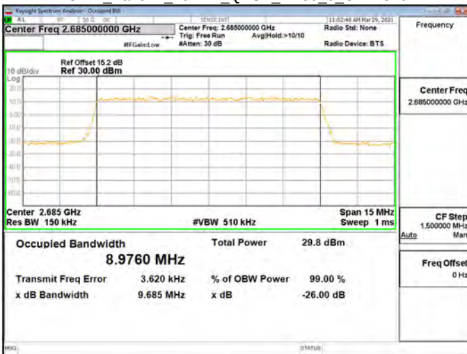
OBW_Band41_10MHz_QPSK_RB50_0_CH41540
