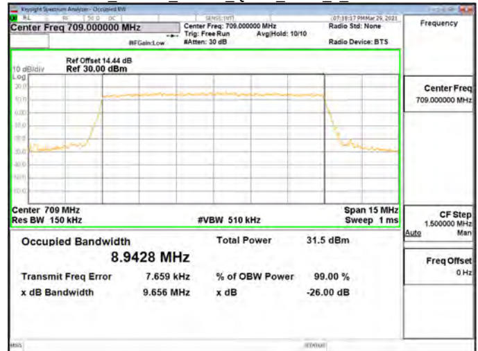
OBW_Band17_10MHz_QPSK_RB50_0_CH23790
