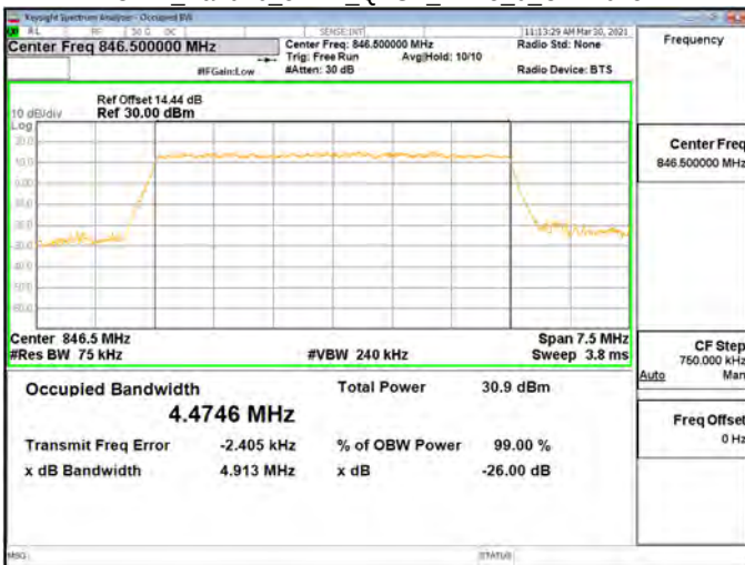
OBW_Band26_5MHz_QPSK_RB25_0_CH27015
