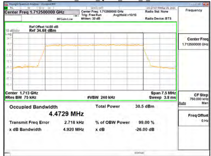
OBW_Band66_5MHz_QPSK_RB25_0_CH132322
