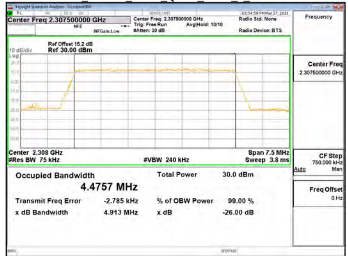
OBW_Band30_5MHz_QPSK_RB25_0_CH27710
