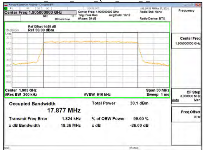
OBW_Band25_20MHz_QPSK_RB100_0_CH26590
