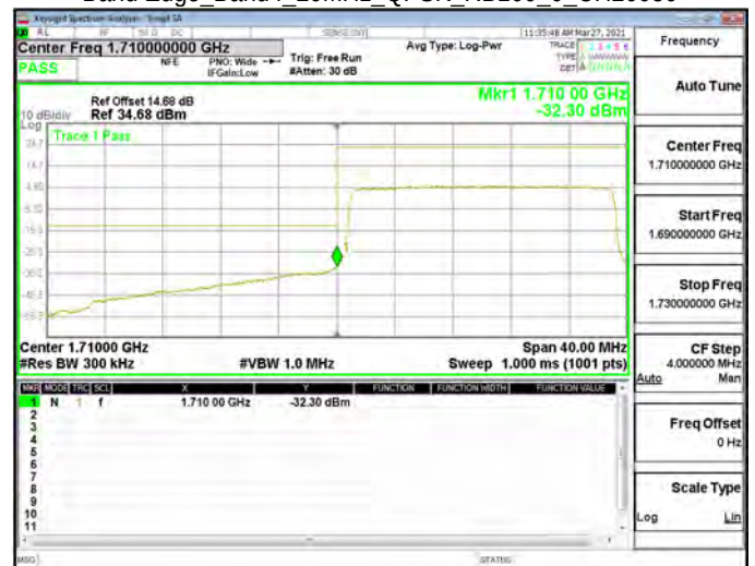
Band Edge_Band4_20MHz_QPSK_RB100_0_CH20300
