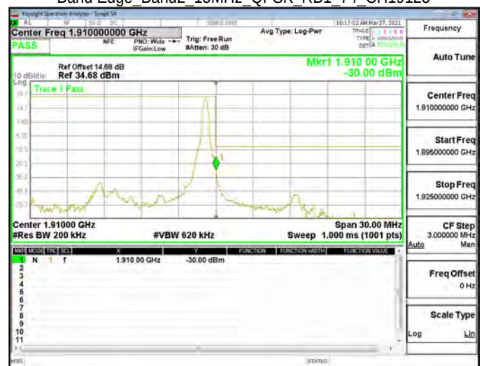
Band Edge_Band2_15MHz_QPSK_RB1_74_CH19125
