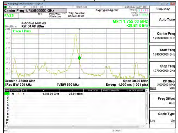
Band Edge_Band4_15MHz_QPSK_RB1_74_CH20325
