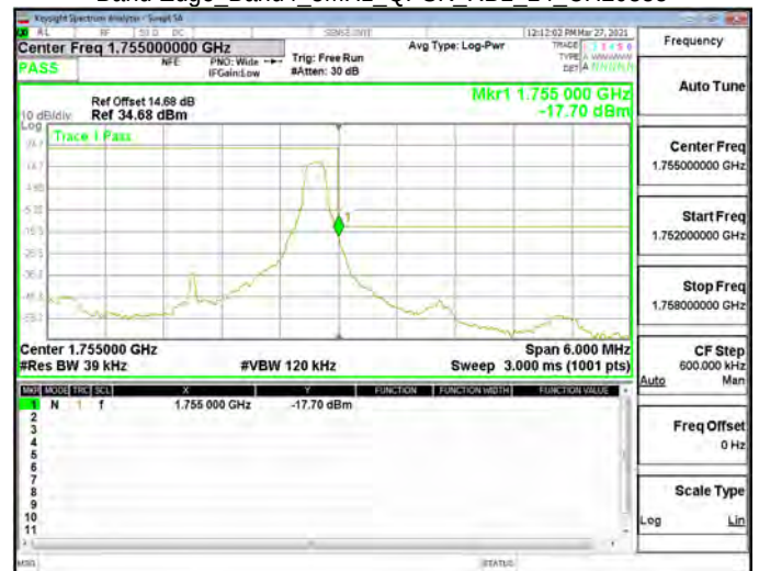
Band Edge_Band4_3MHz_QPSK_RB1_14_CH20385
