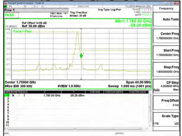
Band Edge_Band66_20MHz_QPSK_RB100_0_CH132072
