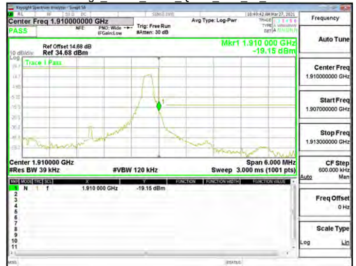
Band Edge_Band2_3MHz_QPSK_RB1_14_CH19185
