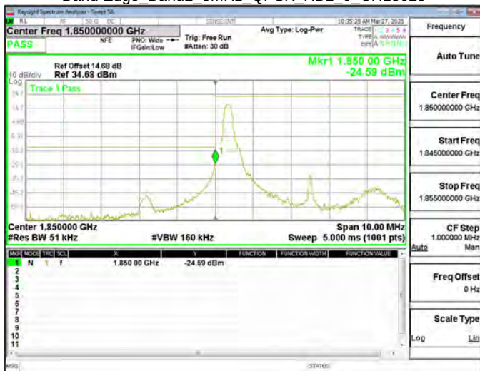
Band Edge_Band2_5MHz_QPSK_RB1_0_CH18625
