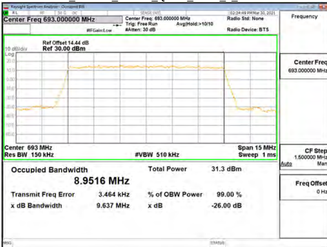
OBW_Band71_10MHz_QPSK_RB50_0_CH133422
