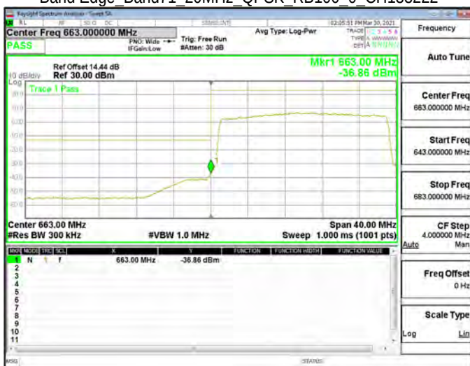
Band Edge_Band71_20MHz_QPSK_RB100_0_CH133222
