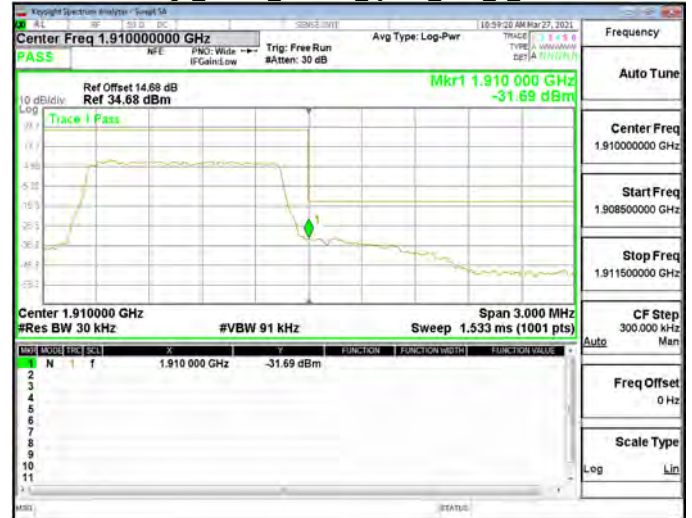
Band Edge_Band2_3MHz_QPSK_RB1_0_CH18615
