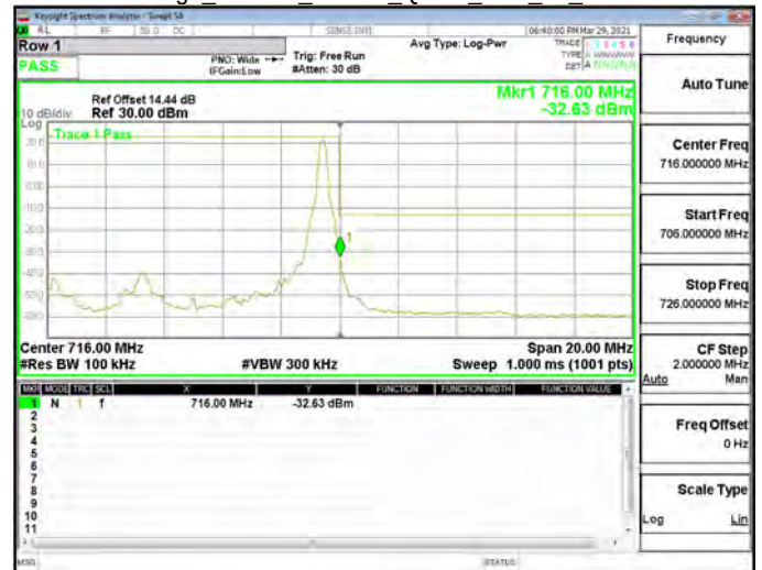
Band Edge_Band12_10MHz_QPSK_RB1_49_CH23130
