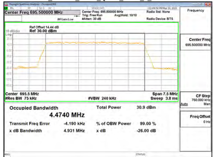
OBW_Band71_5MHz_QPSK_RB25_0_CH133447
