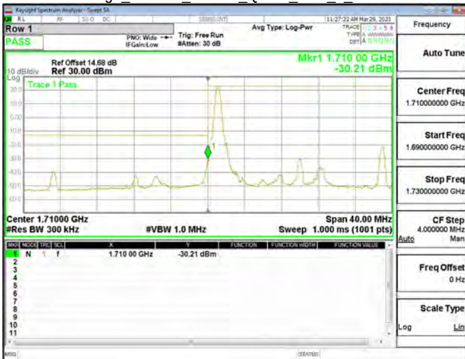
Band Edge_Band66_20MHz_QPSK_RB1_0_CH132072
