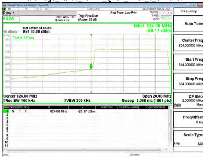
Band Edge_Band5_10MHz_QPSK_RB50_0_CH20450
