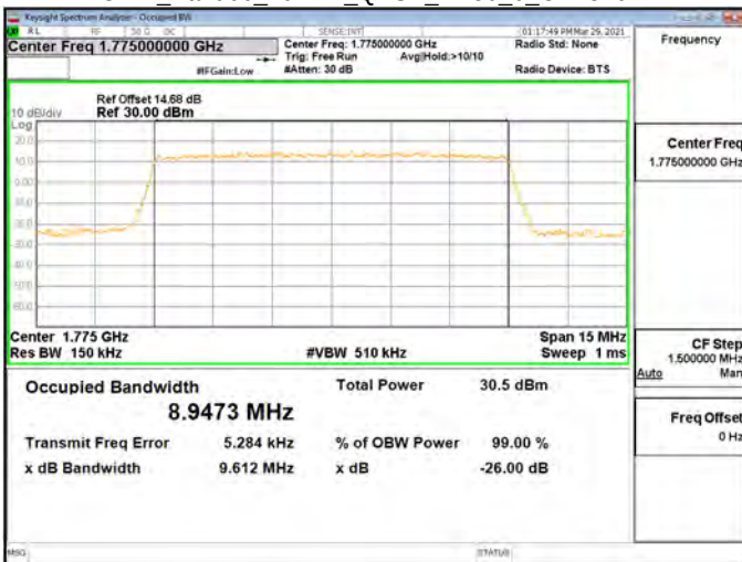
OBW_Band66_10MHz_QPSK_RB50_0_CH132622
