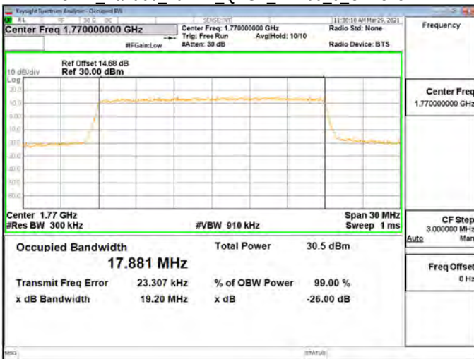
OBW_Band66_20MHz_QPSK_RB100_0_CH132572
