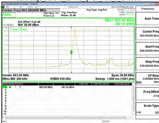
Band Edge_Band71_15MHz_QPSK_RB1_0_CH133197
