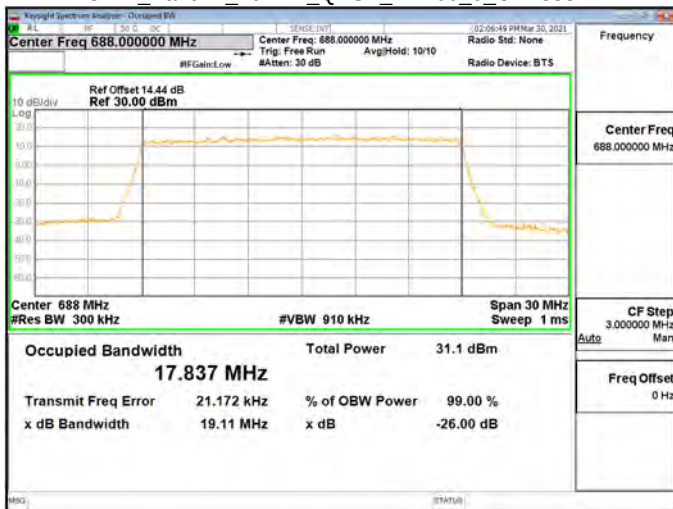
OBW Band71_20MHz_QPSK_RB100_0_CH133372
