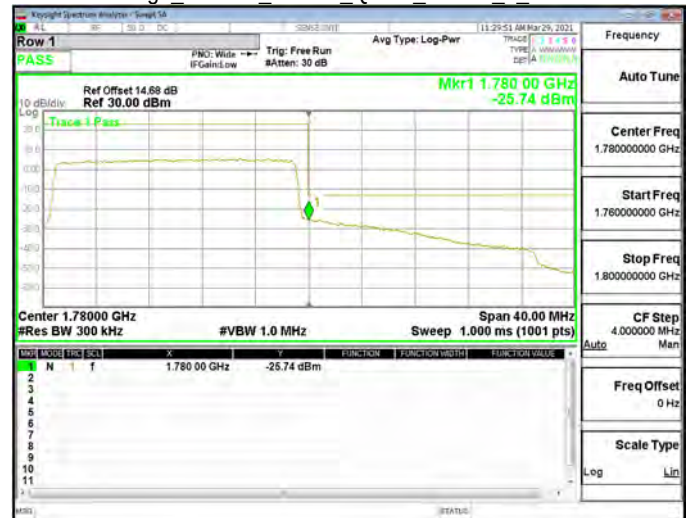
Band Edge_Band66_20MHz_QPSK_RB100_0_CH132572
