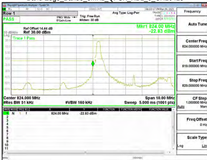
Band Edge_Band5_5MHz_QPSK_RB1_0_CH20425
