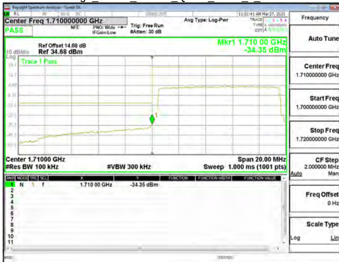
Band Edge_Band4_10MHz_QPSK_RB50_0_CH20000
