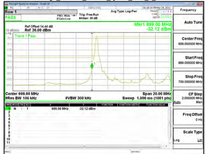
Band Edge_Band12_10MHz_QPSK_RB1_49_CH23130
