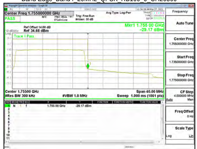
Band Edge_Band4_20MHz_QPSK_RB100_0_CH20300
