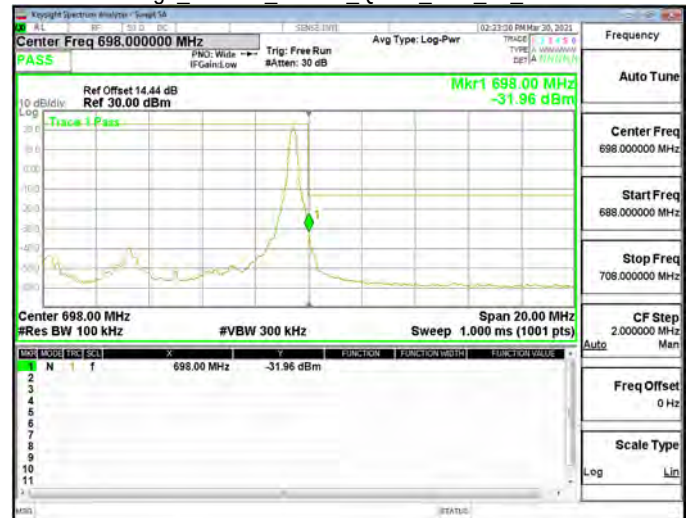
Band Edge_Band71_10MHz_QPSK_RB1_49_CH133422
