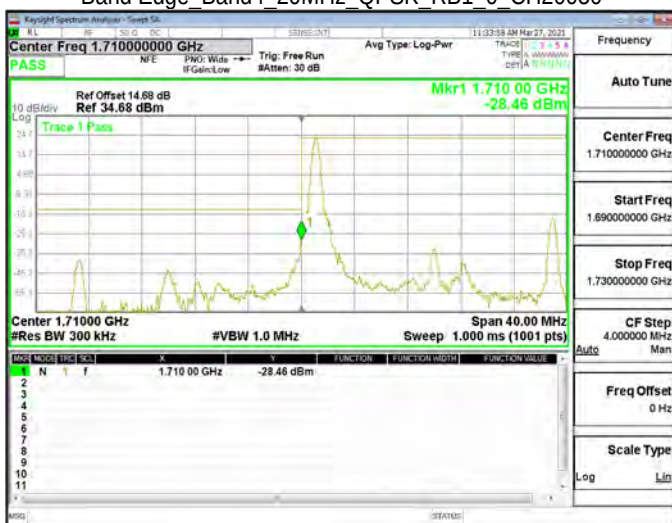
Band Edge_Band4_20MHz_QPSK_RB1_0_CH20050
