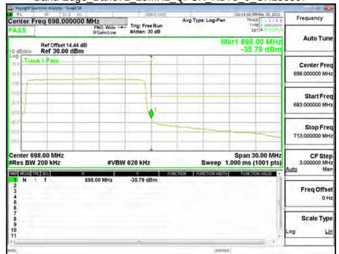
Band Edge_Band71_15MHz_QPSK_RB75_0_CH133397
