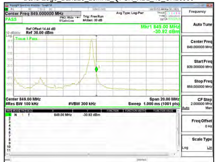
Band Edge_Band26_10MHz_QPSK_RB1_49_CH26990
