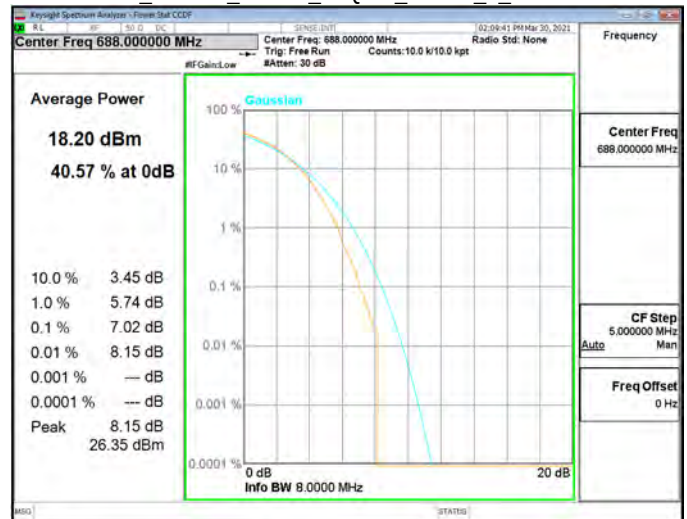
CCDF Band71 20MHz 64QAM_RB100_0 CH133372
