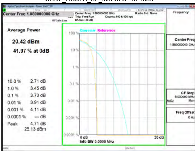
CCDF_HSUPA_B2_Mid CH9400-1880
