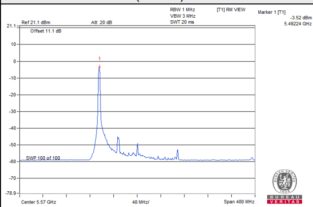
802.11ax (HE160) / CH 114
