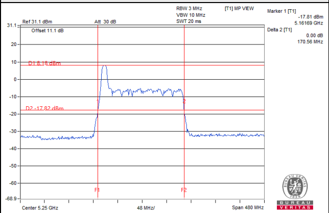
802.11ax (HE160)
