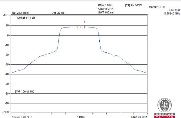
802.11ax (HE40)
