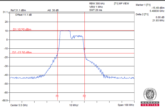
802.11ax (HE80)
